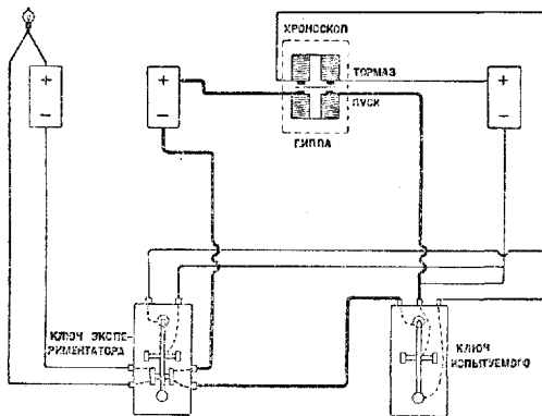
Рис. 4. Схема соединений для измерения времени психической реакции: жирная черта—цепь «спусковых» электромагнитов. Пунктир—соединения отдельных частей ключа внутри последнего.
