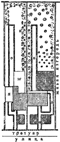
Рис. 10. Разбивка строительных участков в городе-саде (Борнвиль): а—дорожка из гравия; в—фрукт. деревья; г—газоны; ж—площадка для игр; л—двор; о—дорожки; п—посадки; С и с—здания котеджей.
