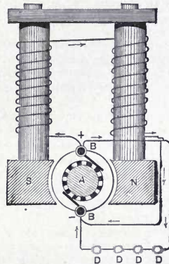
Fig. 357. Shunt Dynamo.
