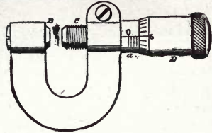
Fig. 283. Vernier Wire Gauge.
