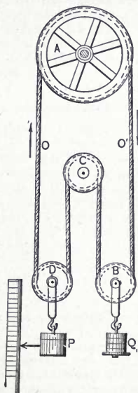
Fig. 223. Parsons' Dynamometer.
