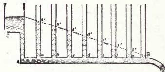
Fig. 449. Hydraulic Gradient.
