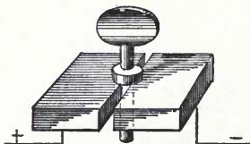
Fig. 327. Plug Key.
