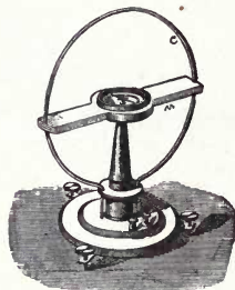
Fig. 277. Tangent Galvanometer.
