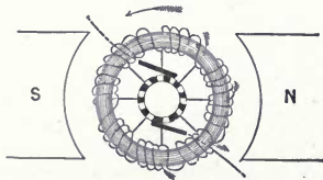
Fig. 20. Bi-polar Armature.
