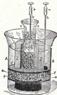
Fig. 113. Siemens-Halske Cell.
