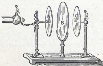
Fig. 167. Æpinus Air Condenser.
