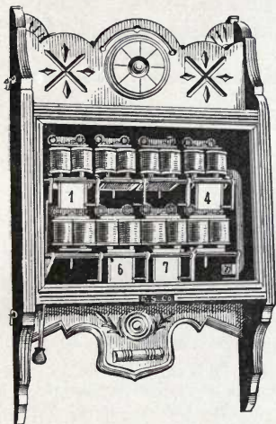
Fig. 16. Gravity-Drop Annunciator.
