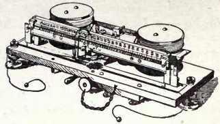
Fig. 33. Centi-Ampère Balance.
