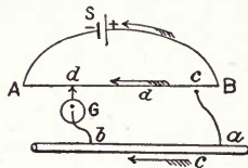
Fig. 451. Potentiometer.
