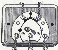
Fig. 25. Comb Lightning-Arrester.
