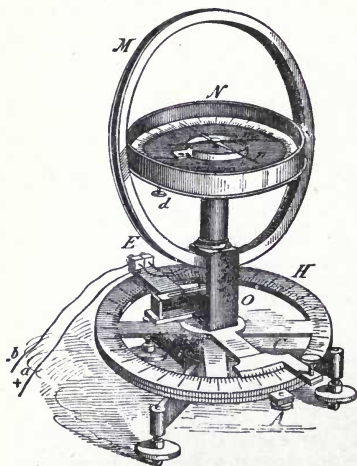
Fig. 276. Sine Galvanometer.
