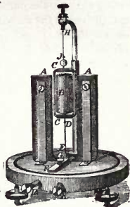
Fig. 271. Deprez-D'Arsonval Galvanometer.
