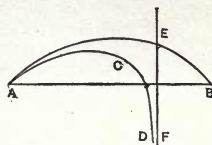
Fig. 187. Ballistic Curve.
