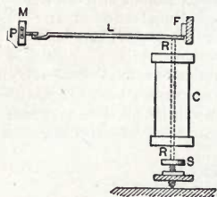
Fig. 383. Bidwell Apparatus.
