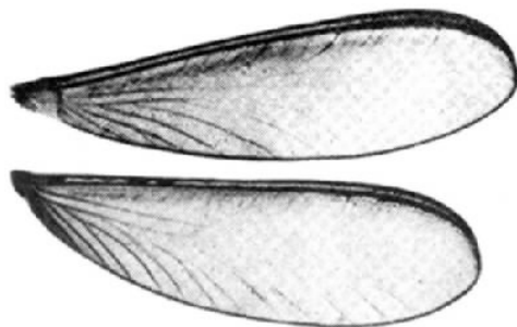
Fig. 126 - Asas de Coptotermes . (Foto J. Pinto)
