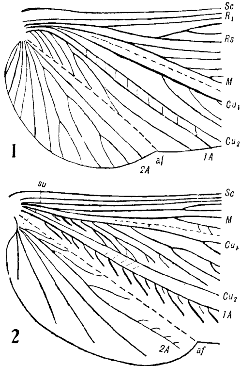
Fig. 154 - 1) Pycnoblattina sp., asa posterior (metade basal); Permiano inferior de Kansas; 2) Mastotermes darwiniensis Frog. Especie recente, Australia septentrional; af, dobra anal; su, sutura humeral (De Tillyard, 1936).
