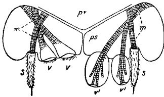
Fig. 6 - Esternitos de Machilidae, com os apêndices ancestrais e respectiva musculatura, m , músculos; pr , prosegmento; ps , post-segmento; s , styli; v , vesículas coxais retraídas; v , vesículas coxais protraídas.
