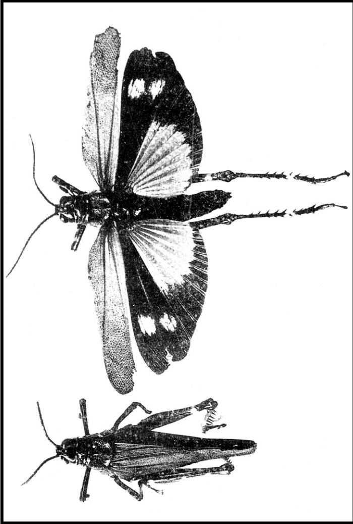
Fig 68 - Chromacris miles (Drury, 1773) (Fam. Acrididae subfam. Cyrtacanthaerinae).
