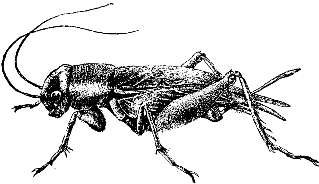
Fig. 80 - Gryllus assimilis Fabr., 1775, ♀ (Fam. Gryllidae) (X 2).
