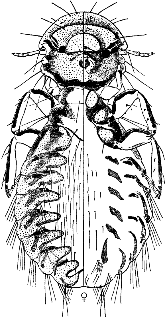
Fig. 175 - Goniocotes gigas Taschenberg; o grande piolho da galinha; á esquerda, aspecto dorsal; á direita, ventral (desenho de Ferris em "Insects of W. N. America", de Essig, fig. 78).
