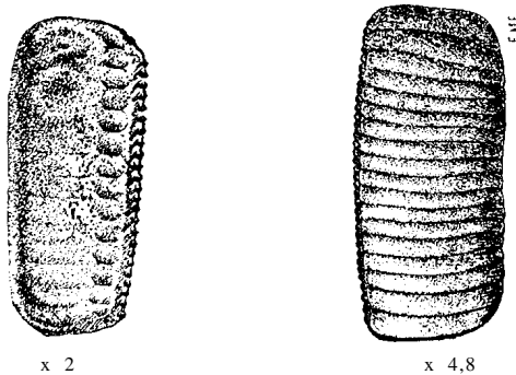
Fig. 110 - Ootécas de Periplaneta australasiae (C. Lacerda del.), (a da esquerda) e de Blattella germanica (segundo Patton, insects, 1931, etc.)
