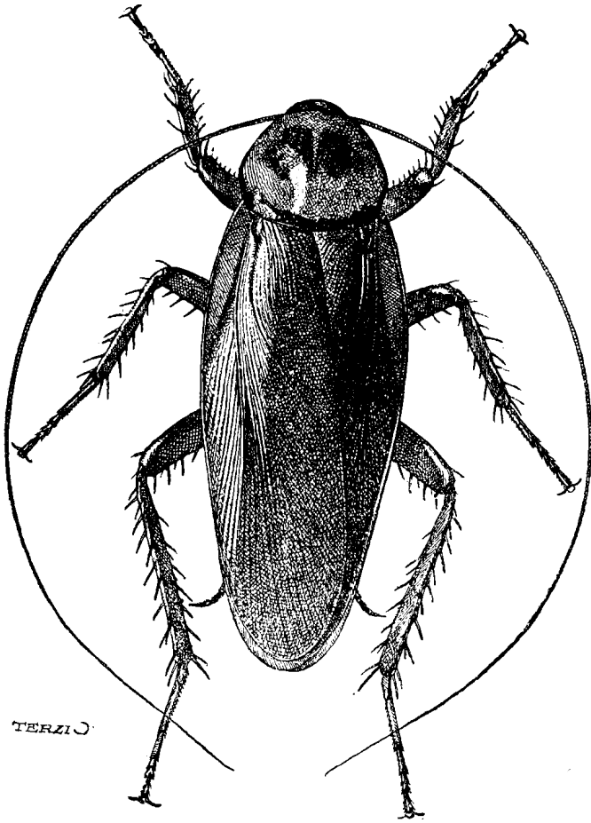
Fig. 106 - Periplaneta americana ♀ (De Patton, Insects, etc., 1931).
