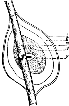
Fig. 140 - Corte esquemático de um ninho arborícola ( cabeça de negro ) de Nasutitermes rippertii . I, involucre exterior; II, camada quebradiça, constituída por camaras arredondadas; III, camada de consistência variável de 2 a 5 cm. de espessura, constituída por celulas menores que as da camada precedente, porém de paredes espessas e duras; IV, camada em que se acha a ninhada, constituída por celulas grandes e chatas; V, nucleo central, em cartão muito duro; no meio a celula real, chata e horizontal (De Holmgren, 1906, fig. Q2).
