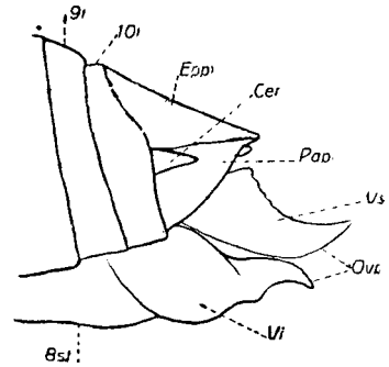
Fig. 62 - Extremidade do abdômen da fêmea de Schistocerca : Eppt , placa supranal ou epiprocto (12° tergito); Cer , cerco; Ovp , ovipositor; Papt , paraprocto; Vi , valva inferior do ovipositor; Vs , valva superior do ovipositor; 8st , pisco infranal ou subgenital (8° esternito).
