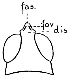
Fig. 58 - Vertex com foveolas laterais: fas. , fastigium; fov , foveolas; dis , disco do vertex (De Blatchley, 1920, fig. 4, segundo Luggler).
