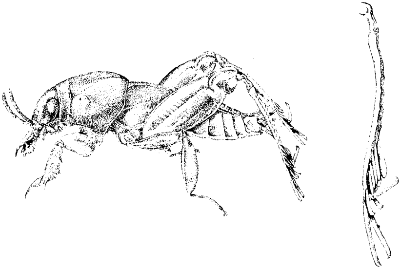
Fig. 86 - Tridactylus politus Bruner, 1916 (Fam. Tridactylidae) (X 14): ao lado a tibia posterior, fortemente aumentada.
