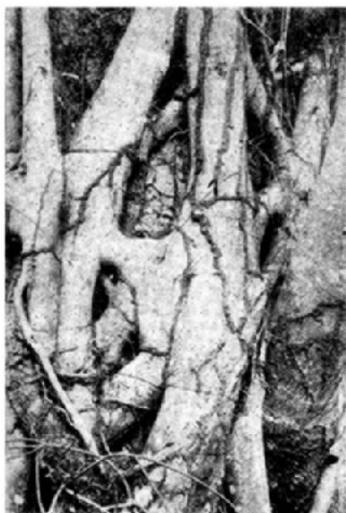
Fig. 141 - Raízes de Ficus sobre um tronco de árvore, com galerias de Nasutitermes , que comunicam a parte subterrânea da comunidade com o termiteio (cabeça de negro) assestado na parte superior do tronco (De Massart, Miss. Biol. Brésil, 1929, 1, fig. 39).
