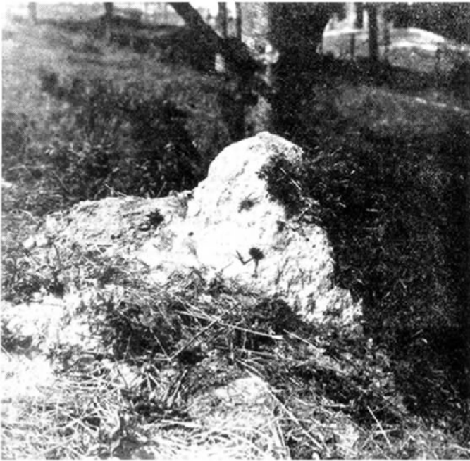
Fig. 148 - Termiteiro de Syntermes dirus , em Manguinhos (pouco mais de 1 metro de altura).
