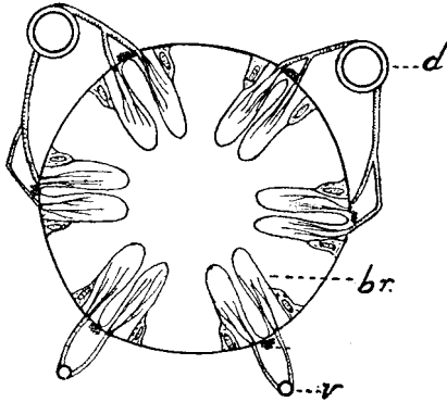
Fig. 43 - Secção transversal, esquemática, do réto de uma ninfa de libelula (De Tillyard, 1917).
