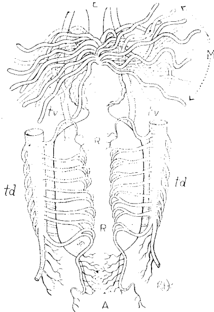
Fig. 42 - Proctodaeum (intestino posterior) de uma ninfa de Aeshna com a empola fetal recebendo as ramificações dos 2 grossos troncos traqueais dorsais, que se distribuem nas traqueo-branquias internas: A, anus; E, mesenteron (intestino medio); M, tubos de Malpighi; R, réto; td, troncos traquiaes dorsais; tv, troncos traquiaes ventrais (De Oustalet, 1869).
