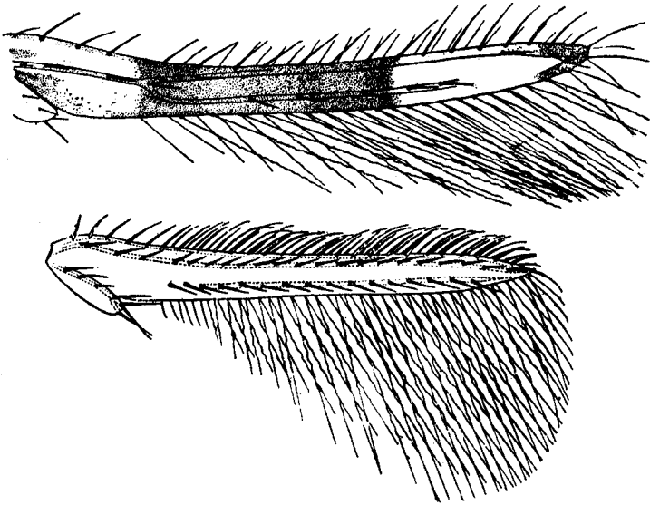
Fig. 199 - Asas anteriores de especies da subordem Terebrantia; em cima, de Hercothrips phaseoli (Hood) (X 361) (De Hood, 1912); em baixo, de Frankliniella insularis (Franklin) (De Franklin, 1908, est. 65, fig. 19).
