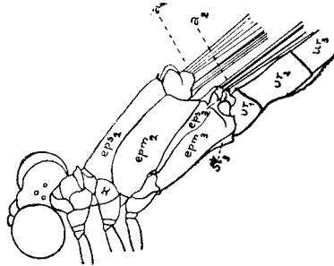
Fig. 24 - Mecistogaster sp. (Zygoptera, Coenagriidae, Pseudostigmatinae); a_1 e a_2 1° e 2° pares de asas; epm_2 e epm_3 epimeros do mesotorax e do metatorax eps_2 e eps_3 episternos do mesotorax e do metatorax st_3 , metasternum; ur_1 , ur_2 , ur_3 , 1°, 2° e 3° uromeros; x , mesinfraepisternum.
