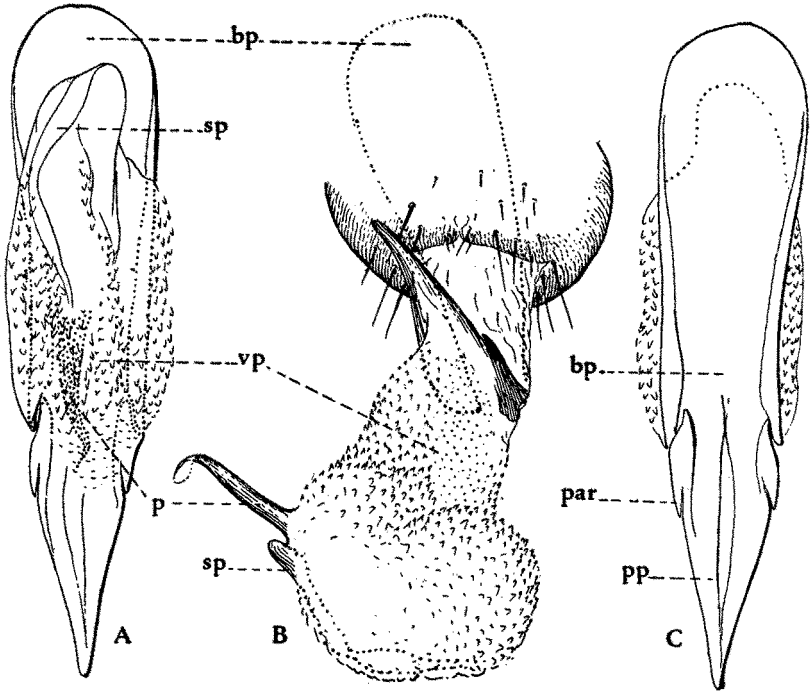
Fig. 184 - Pediculus humanus Linnaeus genitalia do macho; A, aspecto dorsal; B, em prolapso; C, aspecto ventral; bp, placa basal; p, penis; par, parameros; pp, pseudopenis; sp, statumen penais; vp, vesícula do penis. (Desenho e terminologia de Ferris, 1935, fig. 325).
