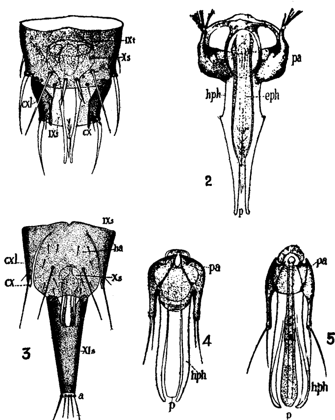
Fig. 202 - 1-2, Frankliniella insularis (Franklin) (subordem Terebrantia); 1, aspecto dorsal do 9º uromero do macho (10º e 11º tergitos retirados); 2, genitalia do macho; 3-4, Leptothrips mali Fitch; 5, Trichothrips americanus Hood (ambos da subordem Tubulifera); 3, aspecto dorsal dos uromeros terminais; 4-5, aspecto dorsal da genitalia do macho. a, orifício anal; ex, coxito; cxl, lobo coxal; eph, epiphallus; ha, hypandrium; hph, hypophallus (parameros de Verhoeff); p, phallus; pa, perianthrium; IXs-XIs, 9º, 10º e 11º esternitos; IXt-XIt, 9º, 10º e 11º tergitos. Figuras e terminologia de De Gryse & Treherne, 1924).
