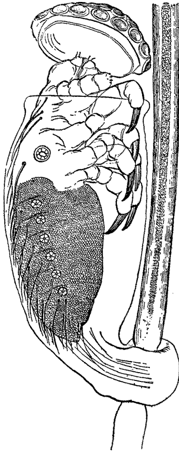
Fig. 188 - Linognathus pedalis (Osborn). Ecdusão da forma joven. (De Lahille, 1920, est. 3).
