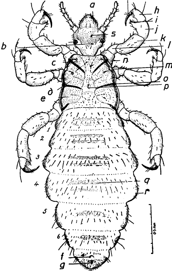
Fig. 180 - Pediculus humanus Linnaeus macho, aspecto dorsal; a, clypeus; b, linha correspondente a sutura epicraneana; c, pro-torax; d, mesotorax; e, metatorax; f, anus; g, dilator; h, tarso; i, polex; j, tibia; k, femur; l, trochanter; n, coxa; m, estigma; o, costela; p, cova esternal; q, faixas transversais; r, placa pleural; 1-6 estigmas abdominais (De Keilin & Nuttall, 1930, est. 3).
