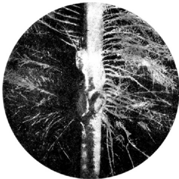
Fig. 169 - Ovos de Mallophaga ao longo do canhão de uma pena (De Reis & Nobrega, 1936, fig. 307)
