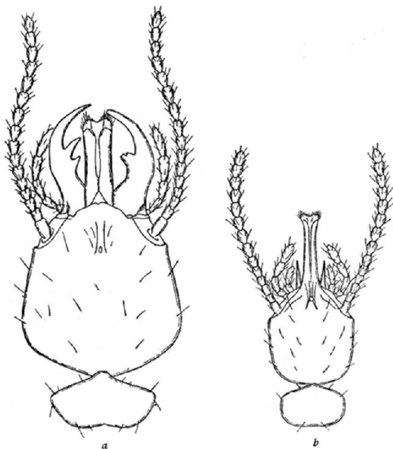
Fig. 132 - Cabeças de 2 tipos de soldados encontrados na mesma colonia de Rhinotermes latilabrum Snyder, 1926 da bacia do Amazonas; em ambas o labrum é consideravelmente alongado e sobre ele escorre a secreção emitida pela fontanela, toxica para as formigas; no soldado de cabeça grande (a) as mandibulas são bem desenvolvidas; no de cabeça pequena (b) eles são vestigiais, X 20 (De Snyder, in Kofoid, 1934, fig. 2).
