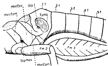
Fig. 60 - Parte do tórax e do abdômen de um acrídeo (vista lateral): Fm 2 , fêmur mesotorácico; Fm 3 , fêmur metatorácico; MesEpm , mesoepimero; MetEps , metaepisternum; Stg 1 , 1º estigma abdominal; Stg Mes , estigma mesotorácico; Tymp , tímpano; 1t-5t , 1º-5º urotergitos.
