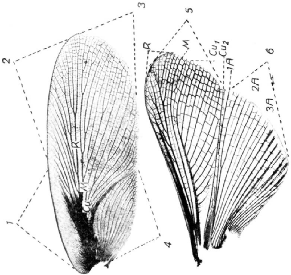
Fig. 98 - Asas de Blaberus sp. 1, campo marginal; 2, campo escapular; 3, campo podisoidal; 4, campo anal; 5, campo anterior (campo marginal + campo discoidal); 6, campo posterior; Cu_1 , cubital (ulnaris posterior); Cu_2 , Vena dívidens ou sutura analis; M , medial (ulnaris anterior, na asa posterior: spuria); R , radio (radialis).
