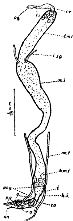
Fig. 204 - Tubo digestivo de Heliothrips haemorrhoidalis ; er , proventriculo; fi , intestino anterior (stomodaeum); f.m.i. , porção anterior do mesenteron; g , parte glandular; h.m.i. , porção posterior d mesenteron; h.i. , intestino posterior; i , ilium; l.s.g. , canais escretores das longas glandulas salivares; m.i. , mesenteron; m.t. , tubo de Malpighi; oe , esofago, r , rectum; rg , glandula rectal; h.g. , parte post-glandular; pr.g. , parte pre-glandular. (De Sharga, 1933, est. X, fig. 4).
