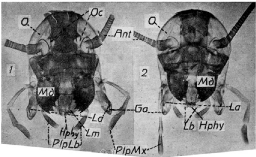
Fig. 97 - Cabeças de Periplaneta americana (1) e de P. australasiae (2); Ga , galea, Hphy , hipofaringe, la , lacinia (em P. americana ponteaguda, em P. australasiae truncada no apite), Lb , labium (só aparecem as paraglossas), Lm , labrum (de bordo reintrante no meio), Md , mandíbula (com dentes mais agudos em P. americana ), O , olho, Oc , fenestras , PlpMx , palpo maxilar, PlpLb , palpo labial (x 56).
