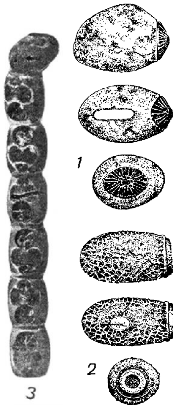
Fig. 91 - Ovos de Fasmídeos: 1, de Phibalosoma phyllinum , X 5; 2, de Pseudocyphides tithonus (Gray, 1835) (sub-fam. Pseudophasminae), X 10; 3, de Prisopus ohrtmanni (Lichtenstein 1802), X 3,5 (sub-fam. Pseudophasminae).
