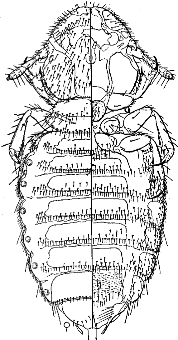
Fig 178 - Trichodectes bovis (Linne); Mallophago do boi; à esquerda, aspecto dorsal; à direita, ventral (desenho de Ferris em "Insects of N. W. America", de Essig, fig. 77).
