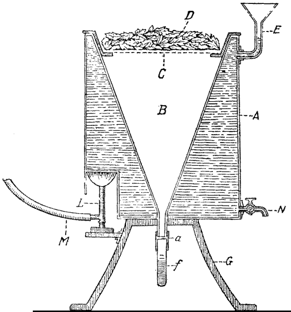
Fig. 9 - Aparelho de Berlese para colheita de Thysanura e Collembola. A, recipiente contendo água; B, funil interior; C, prateleira com fundo de tela metálica; D, material a examinar; E, funil para entrada de água; G, suporte do aparelho; L, bico de gás; M, tubo condutor; N, torneira de descarga; a, cano de borracha ligando o funil interno ao tubo de vidro com álcool; f, que recebe os insetos.
