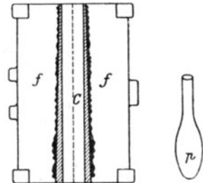
Fig. 278 a. Fig. 278 b. Fig. 278 a und b. Gießform nach Guthmann.
