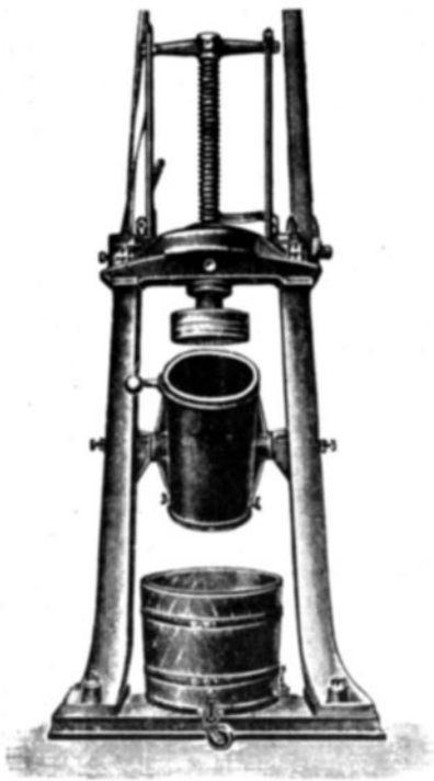
Fig. 51. Butterpresse Bavaria (gekippte Stellung).
