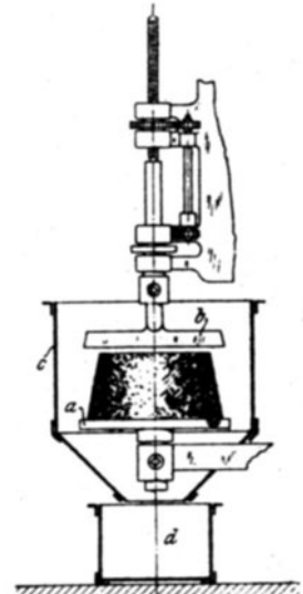
Fig. 66. Abschabeapparat von Schlinck.
