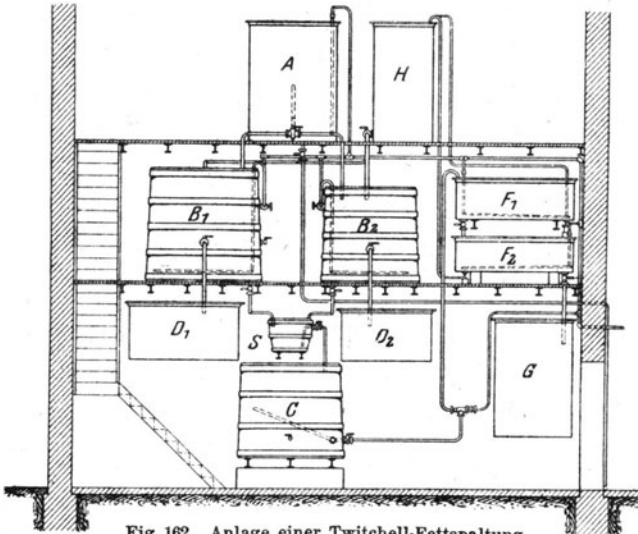
Fig. 162. Anlage einer Twitchell-Fettspaltung
