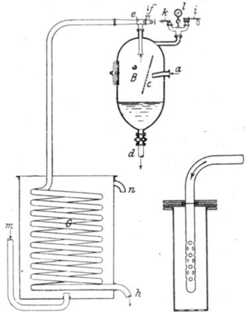
Fig. 99. Ausblasvorrichtung von Friccius Grobian.
