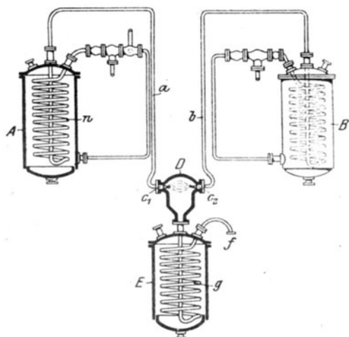
Fig. 114. Schema des Verfahrens Perrelet-Becker.
