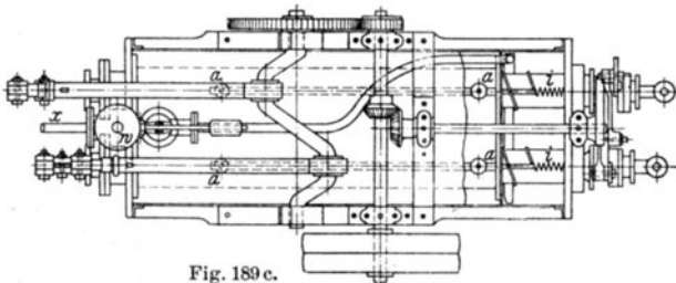
Fig. 189 a—d. Entstearinisierapparat nach Messener.
