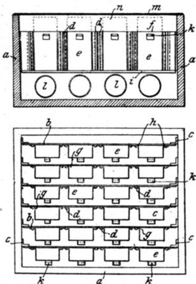
Fig. 64. Formapparat nach de Bruyn.
