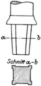
Fig. 270. Kerze mit angesessenem Pyramidenstumpf.
