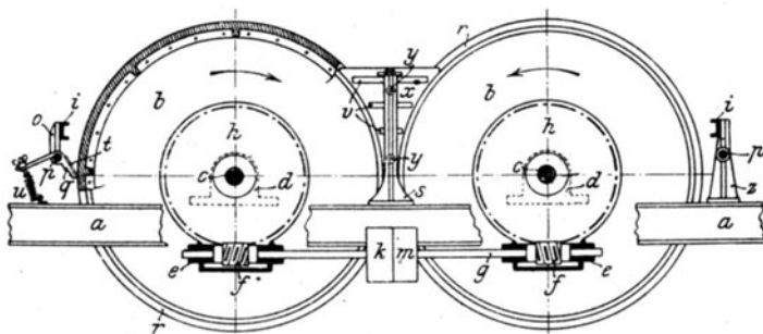
Fig. 29. Kühlapparat nach Schou.
