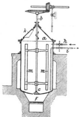
Fig. 69. Apparat zum Voroxydieren des Leinöles in den Linoleumfabriken.
