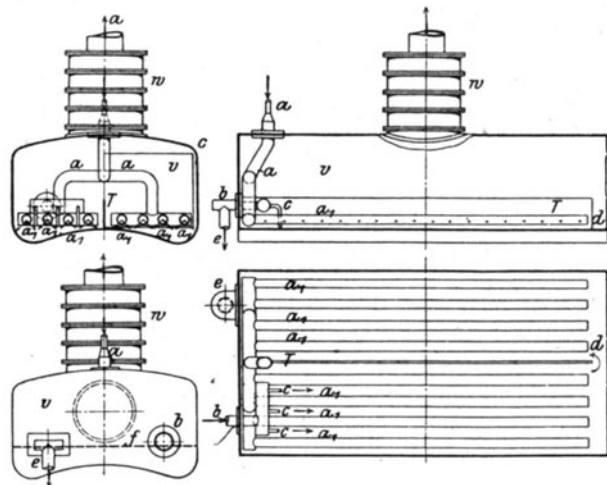
Fig. 158. Kontinuierliche Destillation nach Hirzel.
