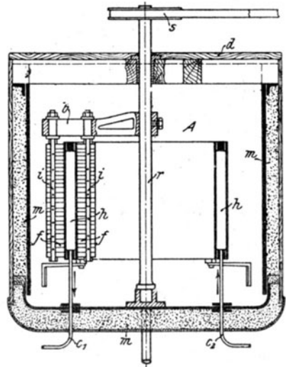
Fig. 186. Kühlapparat nach Zuccari.
