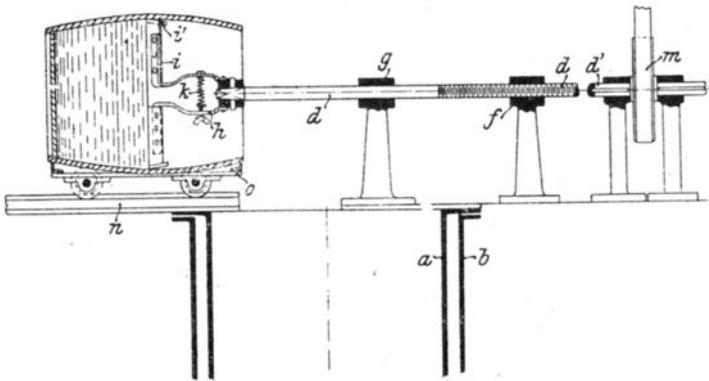
Fig. 14. Horizontale Anordnung des Pfütznerschen Bohrapparates.
