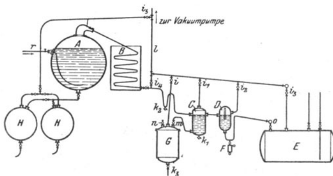
Fig. 161. Schema einer Destillation nach Bokelberg und Sachs.
