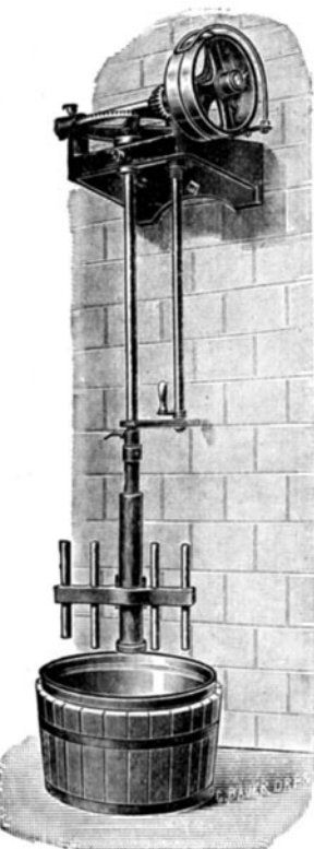
Fig. 234. Vorrichtung zum Kaltrühren der Kerzenmasse.
