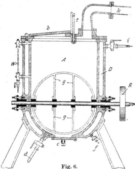
Talgschmelzapparat von Jaroslawski.
