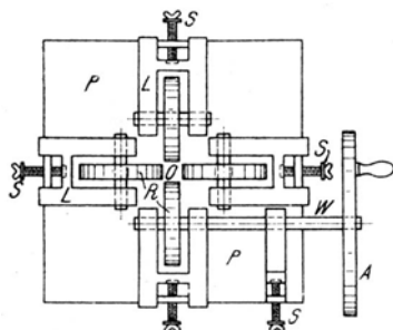
Fig. 274 a. Grundriß.
