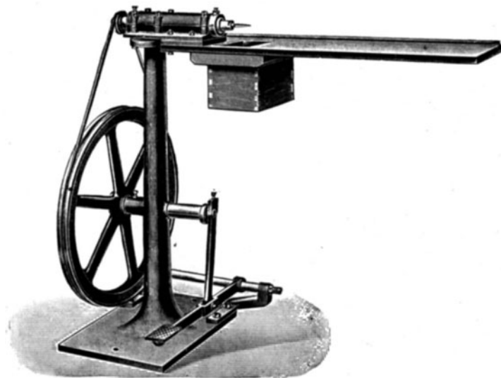
Fig. 253. Kerzenbohrmaschine.
