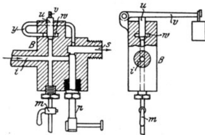
Fig. 55. Pumpendetail des Apparates der Société française pour la conservation des beurres.
