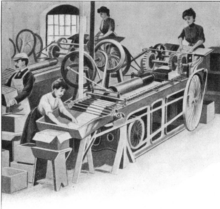
Fig. 259. Kerzenpoliermaschine.
