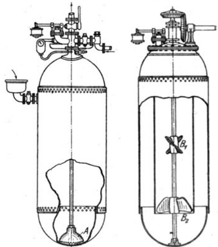
Fig. 91. Autoklav mit Dampfverteilungs- haube.
