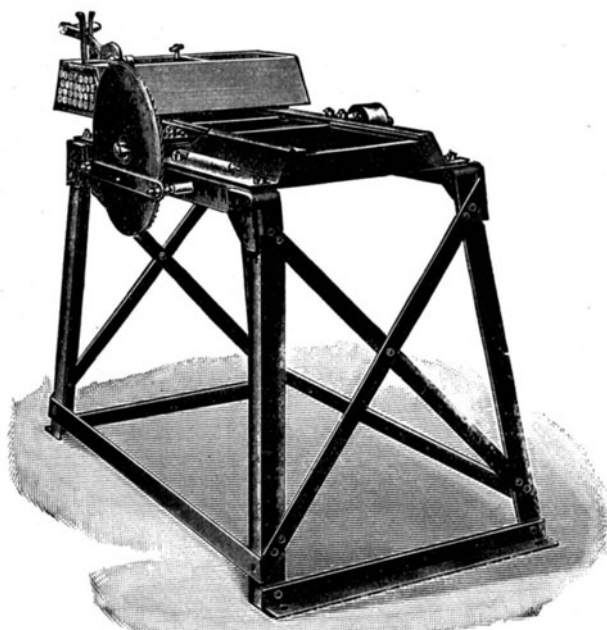
Fig. 252. Kerzenschneidmaschine (Kreissäge mit maschinellm Antrieb).
