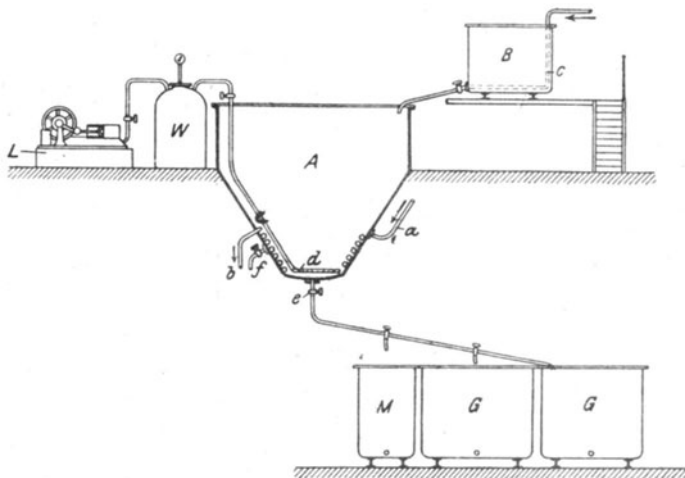
Fig. 164. Schematische Darstellung einer fermentativen Fettspaltungsanlage.
