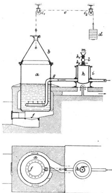
Fig. 70. Apparat zur Herstellung von Linoxyn nach Parnacott.
