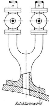
Fig. 88. Gabelrohr für Autoklaven.
