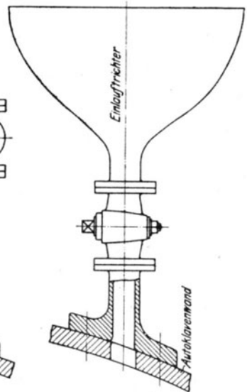
Fig. 89. Fülltrichter.
