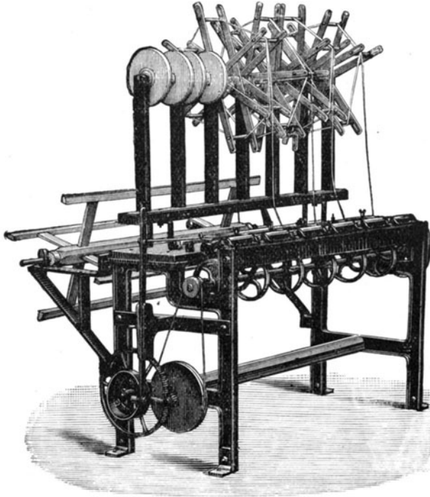
Fig. 206. Sechsgängige Dochtspulmaschine mit Transmissiontrieb.
