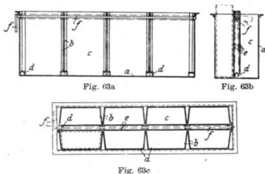
Fig. 63a, b, c. Vorrichtung zum Formen von Kokosbutter von Widmer-Ackermann.
