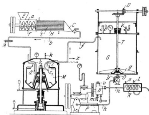
Fig. 54. Apparat zum Haltbarmachen von Kunstbutter.
