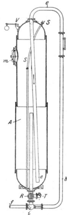
Fig. 94. Autoklav nach Michelin.
