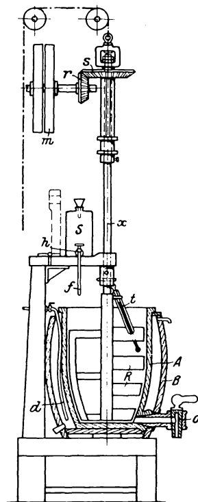
Fig. 83. Vorrichtung zum Sulfurieren von Ölen.
