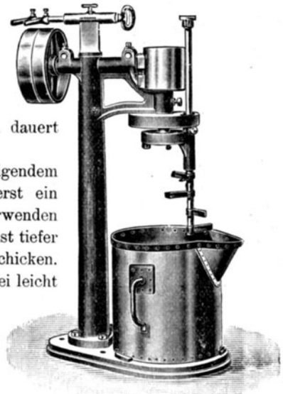
Fig. 235. Vorrichtung zum Kaltrühren der Kerzenmasse.
