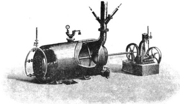
Fig. 128. Sulfurationsapparat nach Droux.
