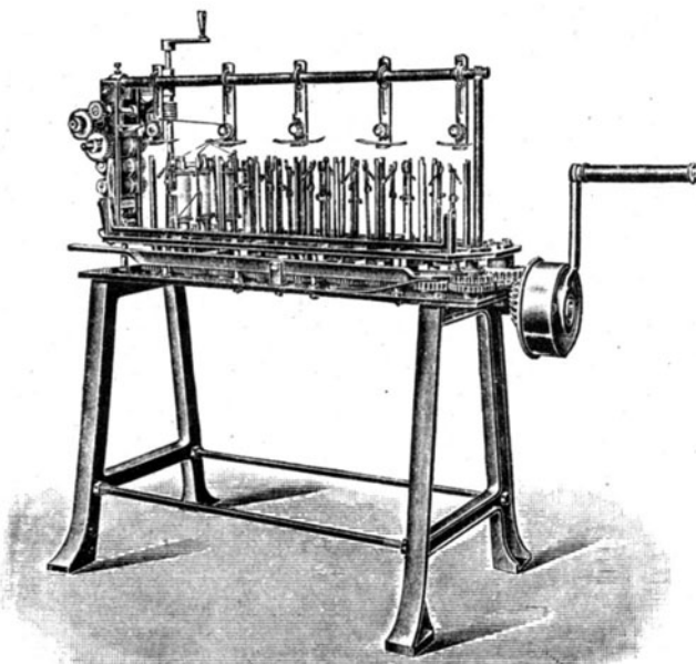
Fig. 201. Dochtflechtmaschine für Handarbeit (System Rost).
