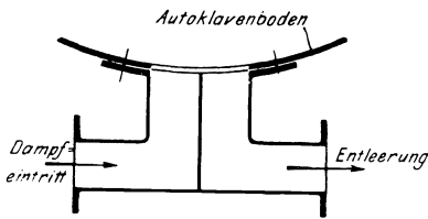
Fig. 90. Entleerungsstutzen.
