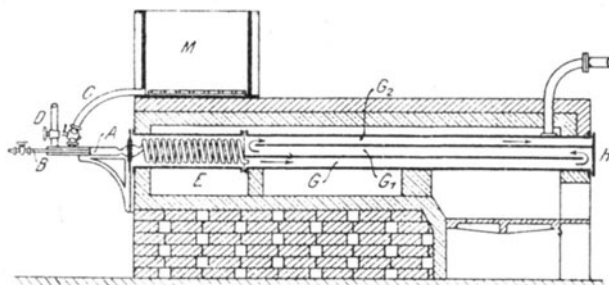
Fig. 113. Apparat von Pielsticker.
