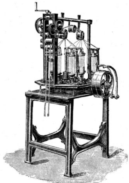
Fig. 202. Dochtflechtmaschine für Kraftbetrieb (System Rost).
