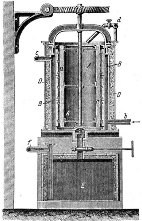
Fig. 185. Kühlapparat für den Kaltpressenablauf.
