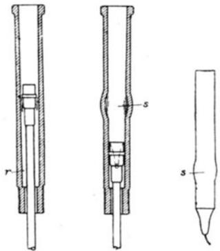
Fig. 242 a. Hochgestelltes Piston. Fig. 242 b. Aufgetriebene Form. Fig. 242 c. Kröpfige Kerze.
