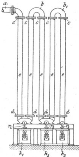
Fig. 146. Luftkühler für Fettsäuredämpfe.
