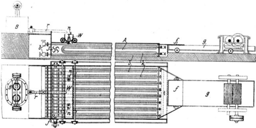
Fig. 28. Kühlvorrichtung nach Donkers.
