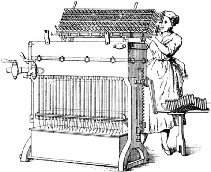
Fig. 232. Herausnehmen der fertigen Kerzen.
