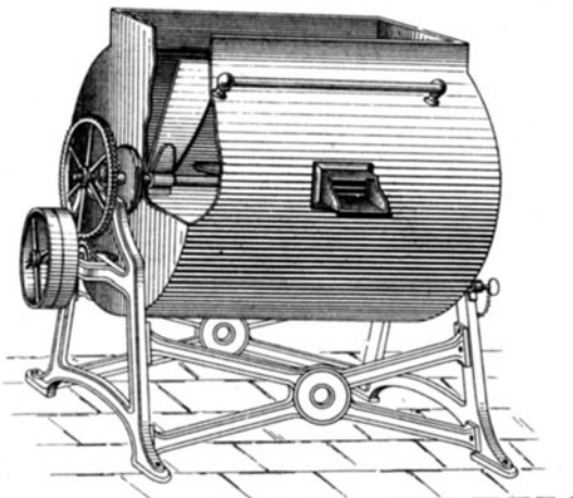
Fig. 236. Vorrichtung zum Kaltrühren der Kerzenmasse.
