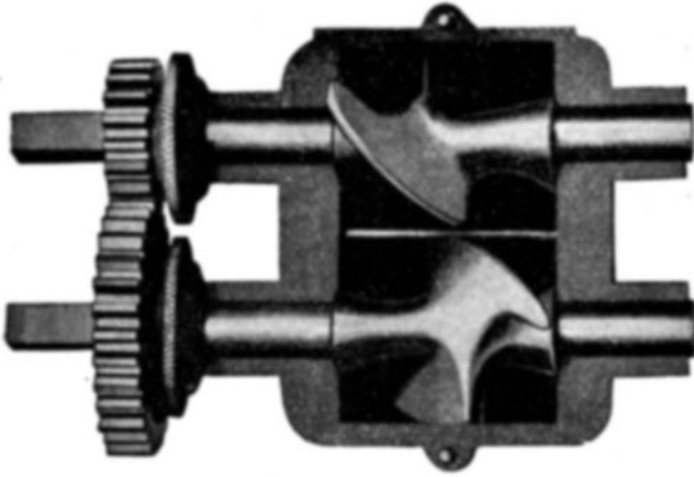
Fig. 47. Prinzip der Werner-Pfleidererschen Misch- und Knetmaschinen.
