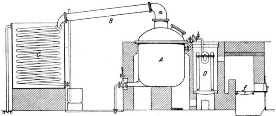
Fig. 134. Schema einer Fettsäuredestillation.
