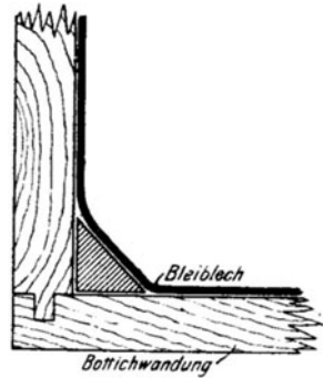
Fig. 123. Details der Bleiverkleidung.
