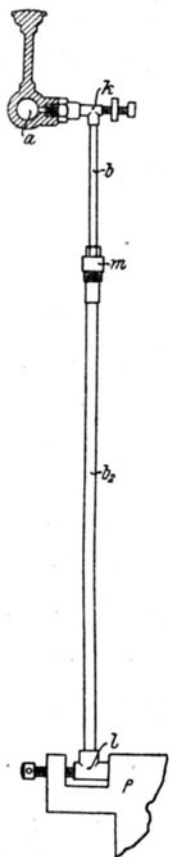
Fig. 177. Detail der Dampf- zuführung bei den Warmpreßplatten.
