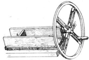
Fig. 250. Kerzenschneidevorrichtung.
