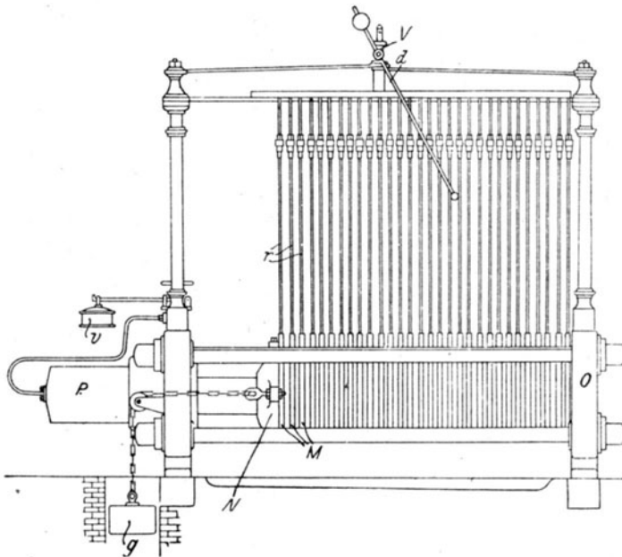
Fig. 169. Stearinwarmpresse.
