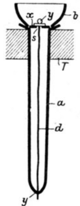
Fig. 220. Talgkerzenform.
