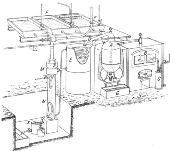
Fig. 153. Vakuumdestillation nach Droux.
