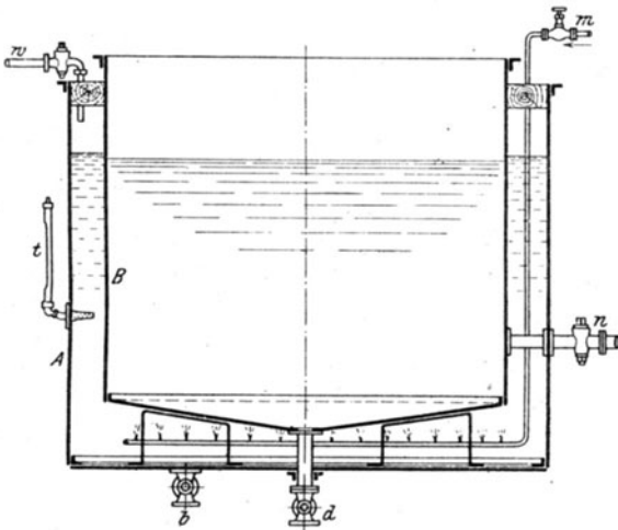
Fig. 8. Marienbad für Premier-jus-Klärung.
