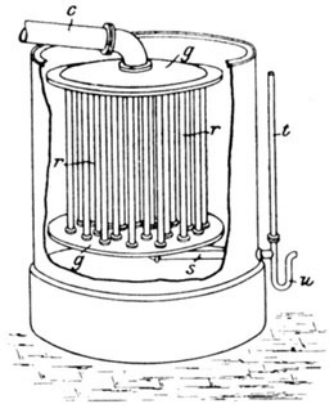
Fig. 143. Wasserkühler mit vertikalen Röhren.
