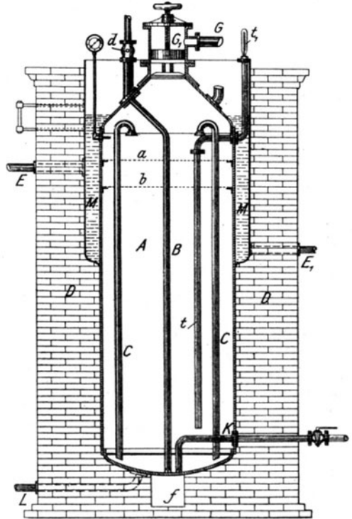
Fig. 104. Fettsplittingsapparat nach Marix.
