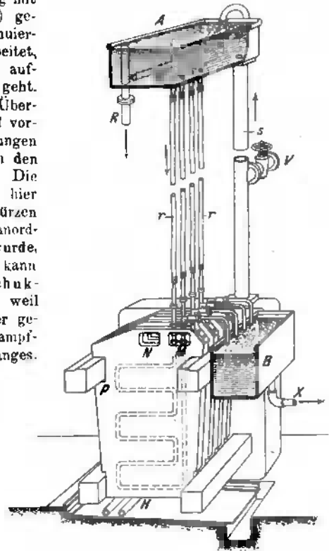
Fig. 178. Preßplatten mit Warmwasserheizung nach Droux.
