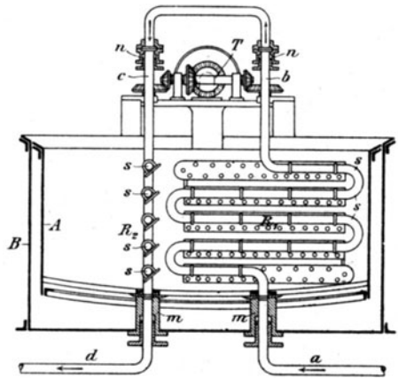
Fig. 17. Kirne mit Rohrrührern nach Donkers.
