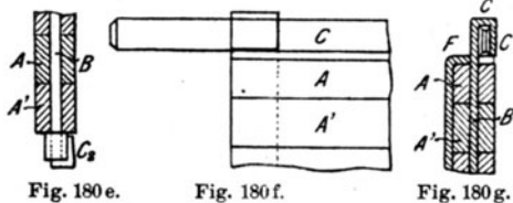
Fig. 180 a—g. Étreindelle nach Lévy.
