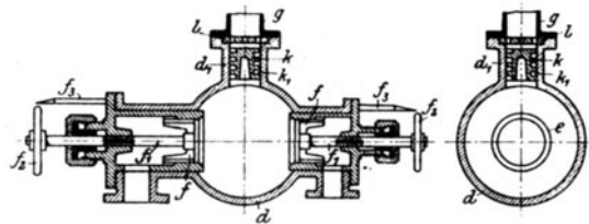
Fig. 116. Streudüse nach Perrelet-Becker.
