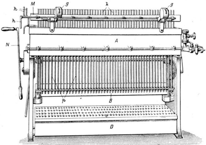
Fig. 226. Moderne Kerzengießmaschine.
