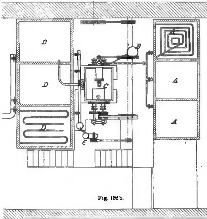
Fig. 182a und b. Sulfurationsanlage nach Engelhardt.
