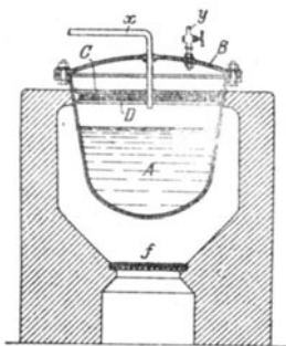
Fig. 290. Apparat zum Eindicken von Pflanzenölen nach Schmitz.
