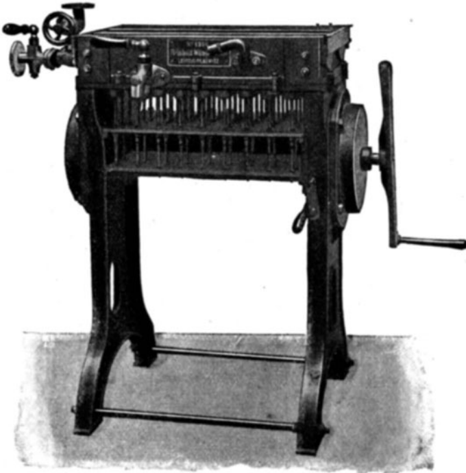
Fig. 288. Gießmaschine für Nachtlichte mit Dochtkanal.
