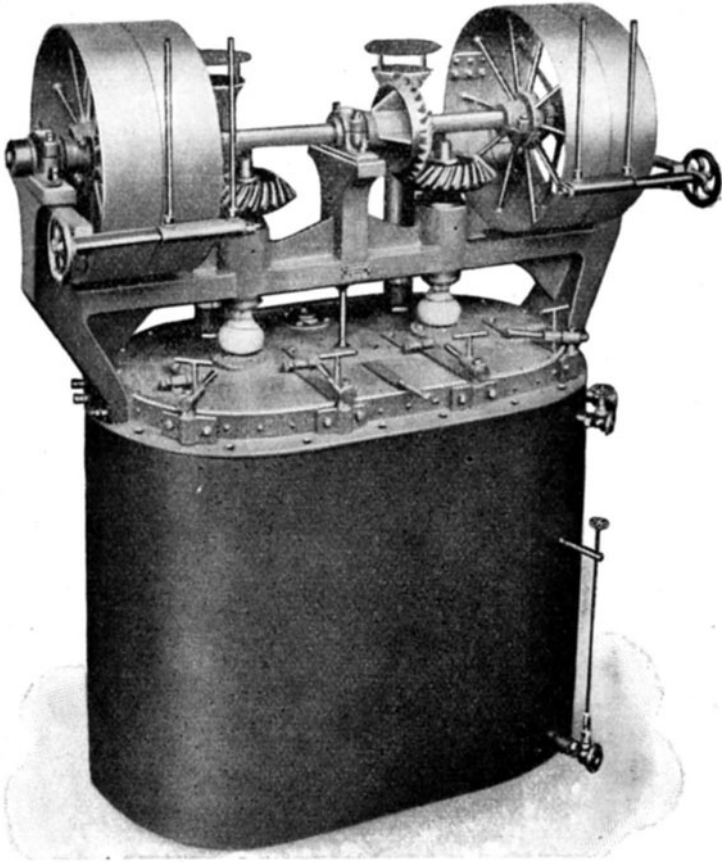
Fig. 16. Kirnapparat.
