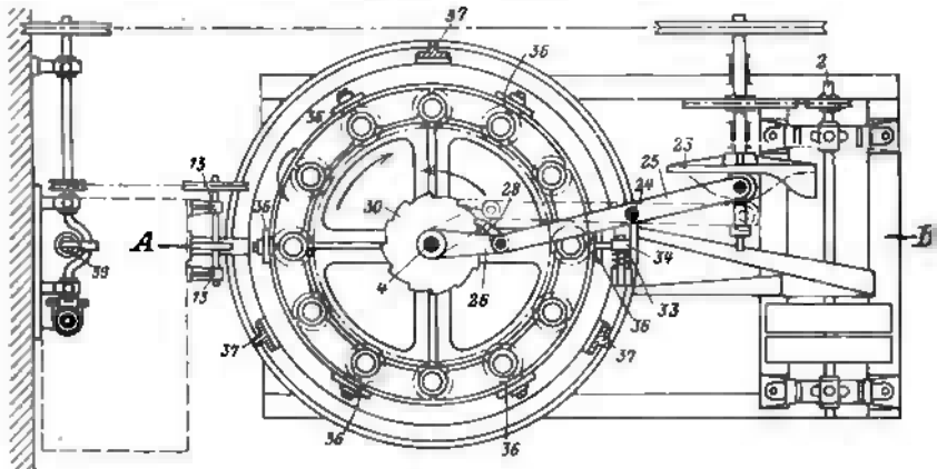
Fig. 219b. Grundriß.
