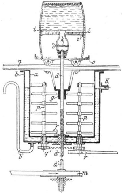
Fig. 13. Fettausbohrvorrichtung von Pfützn er .
