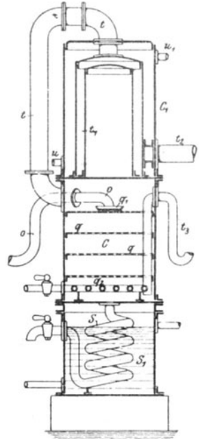
Fig. 141. Destillationsblase nach Sahlfeld.
