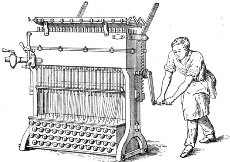
Fig. 231. Ausdrücken der frischgegossenen Kerzen.
