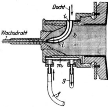
Fig. 207. Wachskerzenpresse nach Rieß.
