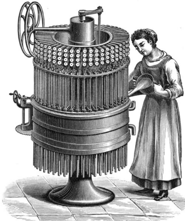
Fig. 245. Kerzengießmaschine.
