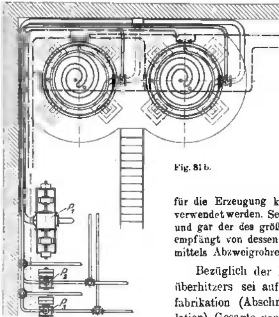
Fig. 81 a und b. Moderne Firnissiederei-Einrichtung.
