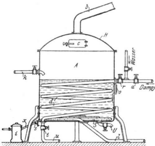
Fig. 68. Apparat zur Herstellung geblasener Öle.
