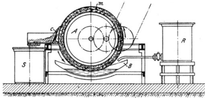
Fig. 30. Kühlvorrichtung nach Möllinger.
