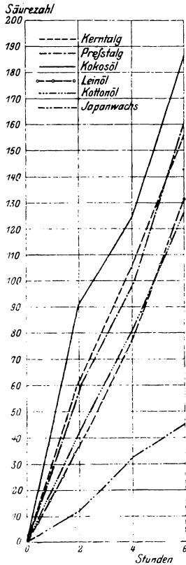
Fig. 121. Verhalten verschiedener Öle und Fette gegenüber Wasserdampf von 15 Atmosphären.
