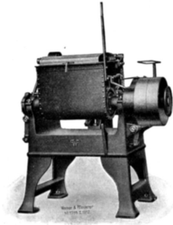
Fig. 48. Misch- und Knetmaschine (System Werner & Pfleiderer) geschlossen
