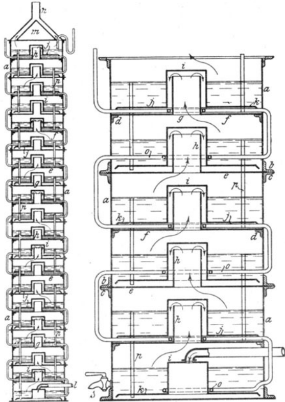
Fig. 60. Desodorisierapparat von Rocca.
