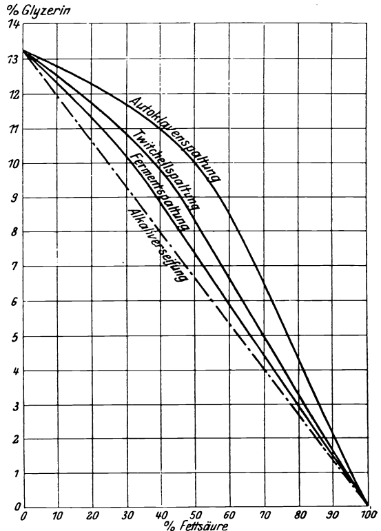
Fig. 84. Verlauf des Verseifungsprozesses bei den verschiedenen Spaltungsmethoden.
