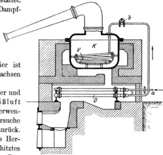
Fig. 76. Firniskochkessel nach Lehmann. D = Dampfüberhitzer, K = Firniskochkessel, a = Einströmung des vom Dampfkessel kommenden Dampfes, b = Absperrventil, V = Dampfspirale.
