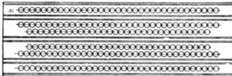
Fig. 241. Draufsicht auf eine Formkastenfläche von 0,514 qm mit 202 Formen (System Rost).
