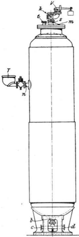
Fig. 85. Zylindrischer Autoklav. T = Fülltrichter, n = Füllstutzen, m = Mannloch, b, s und t = Rohr- stutzen, V = Sicherheitsventil, c und d = Dampfeintritts- bzw. Ent- leerungsstutzen.
