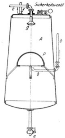
Fig. 119. Fettspaltungsapparat nach Mannig.
