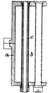
Fig. 243. Eibich-Kuhn- sche Art des Formeinsetzens in den Formkasten.
