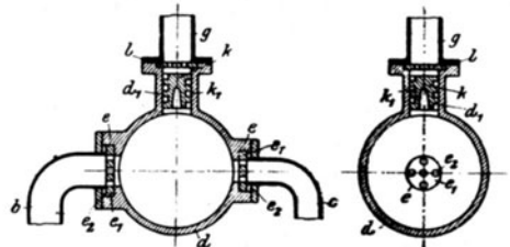
Fig. 115. Streudüse nach Perrelet-Becker.
