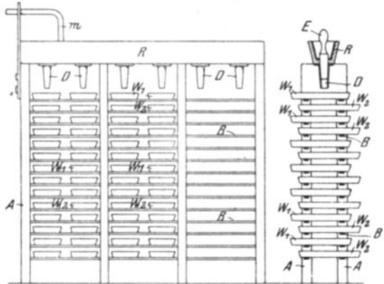
Fig. 166. Binetsches Gestell.
