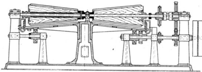
Fig. 46. Bavaria-Butterknetmaschine.
