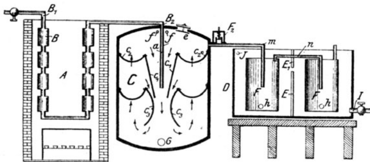
Fig. 112. Fettspaltungsapparat nach William West.
