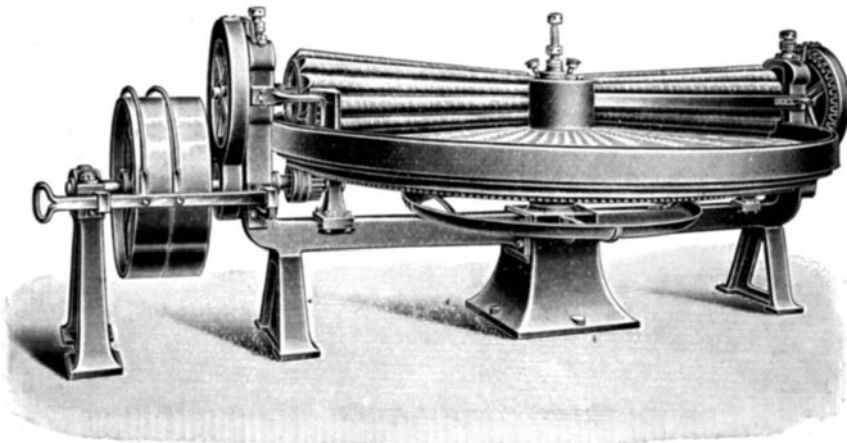
Fig. 44. Malaxeur nach Donkers.
