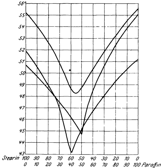
Fig. 200. Schmelzpunkte von Paraffin-Stearin-Gemischen.
