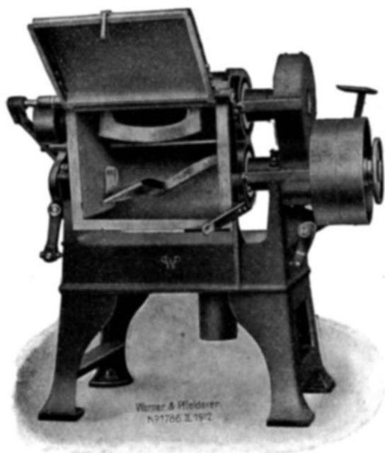
Fig. 49. Misch- und Knetmaschine (System Werner & Pfleiderer) gekippt und geöffnet.
