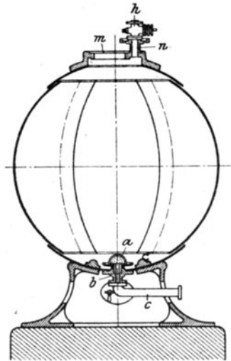
Fig. 86. Kugelförmiger Autoklav. m = Mannloch, n = Füllstutzen, h = Füllhahn, c = Dampfeintritts- und Ausblasrohr, a = Dampfverteilungsbrause, b = Rohrstützen.
