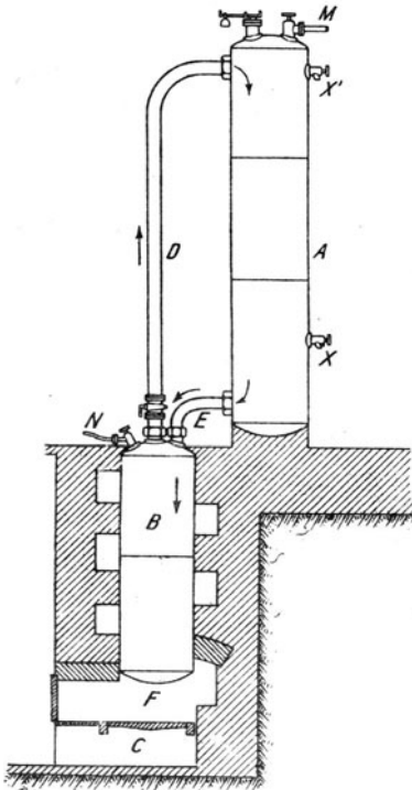
Fig. 102. Fettspaltungsapparat von Wright & Fouché.
