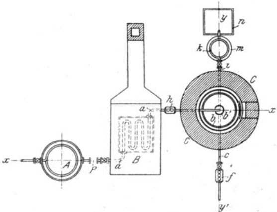
Fig. 100. Fettspaltungsanlage nach Korschelt.
