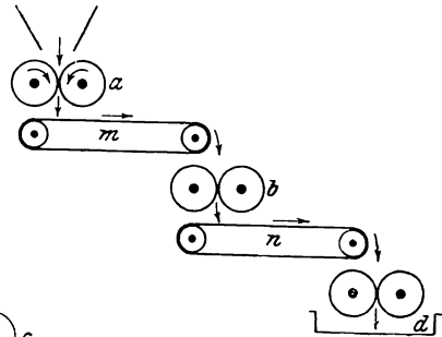
Fig. 36. Schematische Darstellung der Knetvorrichtung nach Plötz (mit endlosem Förderband).
