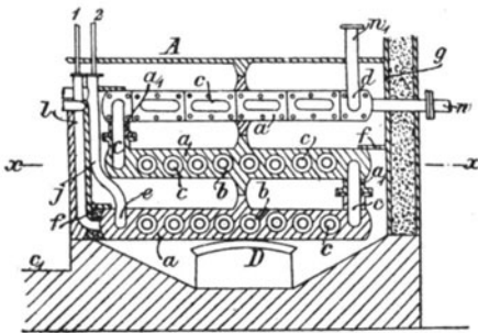
Fig. 151 a. Vertikalschnitt.
