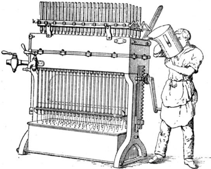
Fig. 230. Eingießen des Kerzenmaterials.
