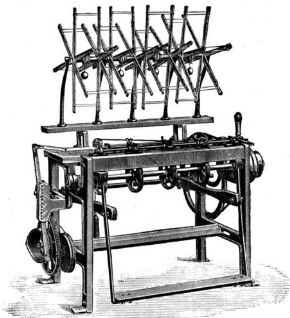
Fig. 205. Viergängige Dochtspulmaschine mit Fußbetrieb.
