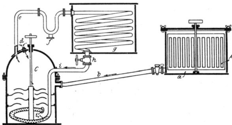
Fig. 27. Kühlvorrichtung nach Scheffel.
