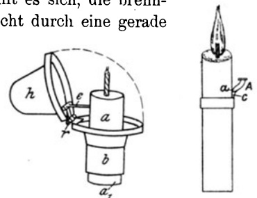
Fig. 283. Kerzen- löscher von Hutwitz.
