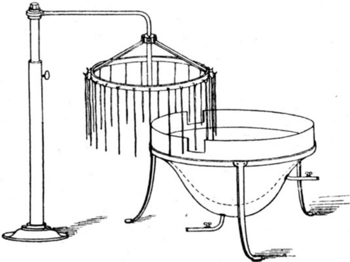
Fig. 218. Vorrichtung zur Herstellung von Kerzen durch Angießen.
