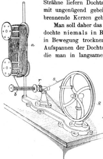
Fig. 208. Einfache Aufspulvorrichtung.
