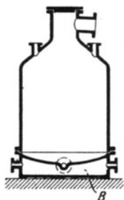
Fig. 135. Fettsäuredestillierblase nach Levy.
