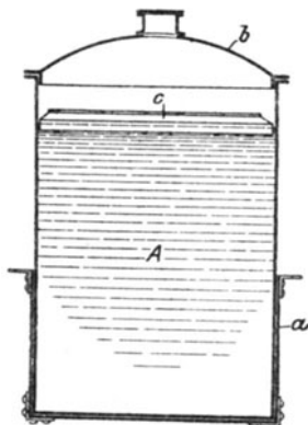
Fig. 291. Apparat zum Eindicken von Pflanzenölen nach Genthe.
