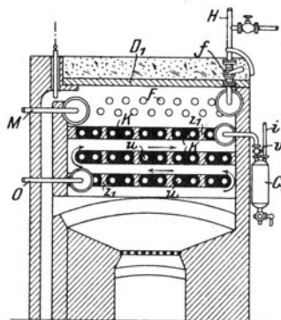
Fig. 149. Überhitzer von Slama.
