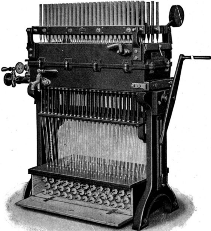
Fig. 229. Kerzengießmaschine nach Wünschmann.
