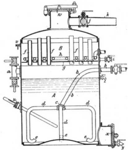
Fig. 137. Destillationsblase nach Scharza.
