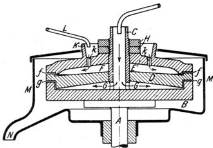
Fig. 21. Emulsor von Schach.
