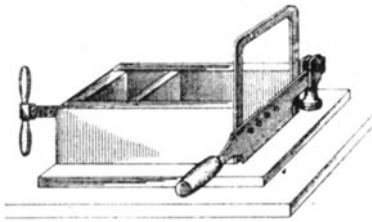
Fig. 249. Kerzenschneidevorrichtung.
