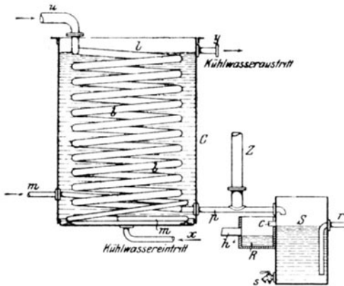
Fig. 142. Schlangenkühler.
