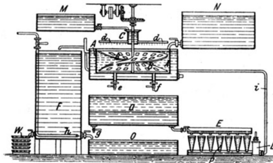
Fig. 194. Anlage zur Umwandlung von Ölsäure in Kerzenmaterial (nach David).
