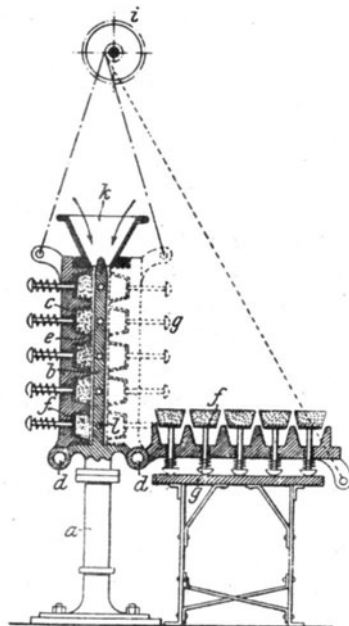
Fig. 62. Vorrichtung zum Formen der Kokosbutter.
