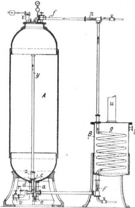
Fig. 93. Autoklav nach Herrnhut.
