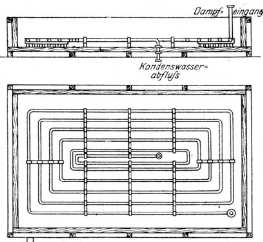
Fig. 126. Eindampfpfanne für das Glycerinwasser.
