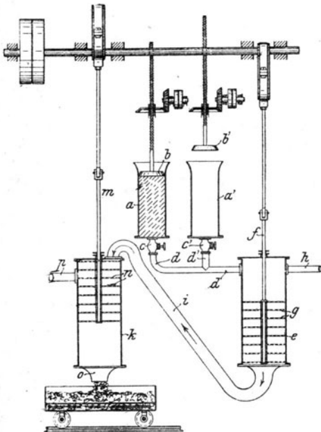
Fig. 18. Kirnvorrichtung von Theberath.
