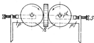
Fig. 274 b. Aufriß.
