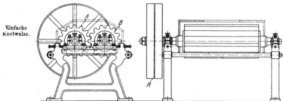
Fig. 32. Einfache Walze für Kunstbutter.
