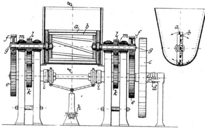
Fig. 50. Misch- und Knetmaschine nach Reibel.
