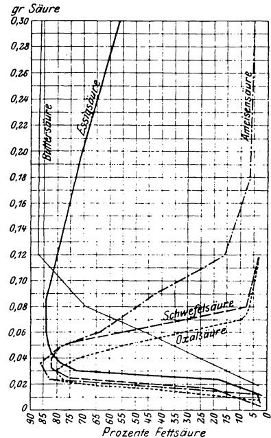
Fig. 163. Graphische Darstellung des Einflusses verschiedener Säuren auf die Spaltwirkung.
