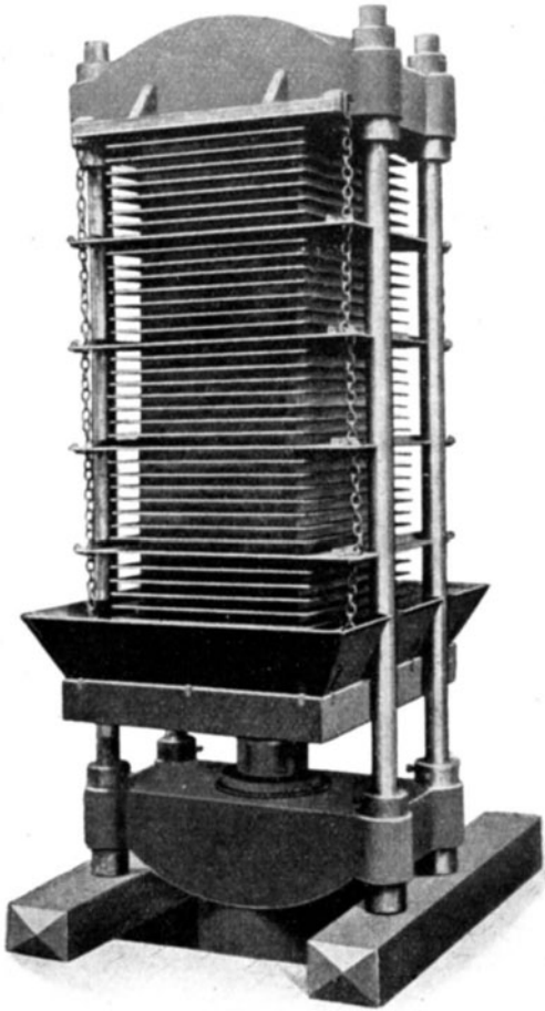
Fig. 10. Oleomargarinpresse.
