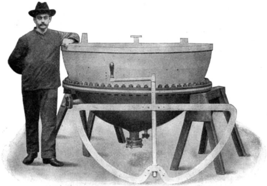
Fig. 77. Firniskochkessel nach Heraeus.
