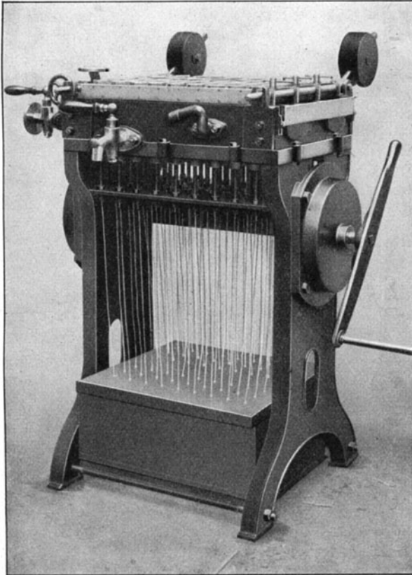
Fig. 287. Nachtlicht-Gießmaschine.
