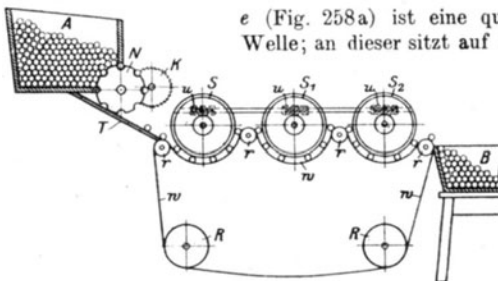
Fig. 257. Schema einer Kerzenpoliermaschine.
