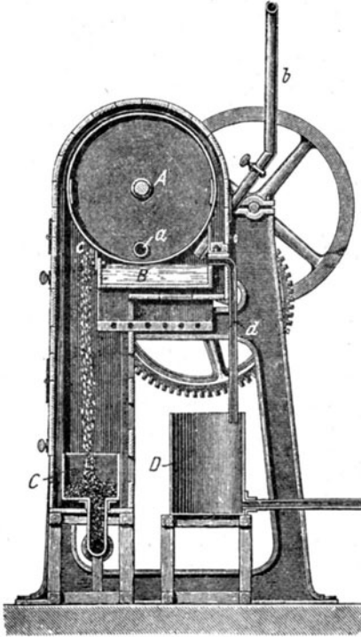
Fig. 184. Kühlapparat für den Kaltpressenablauf.
