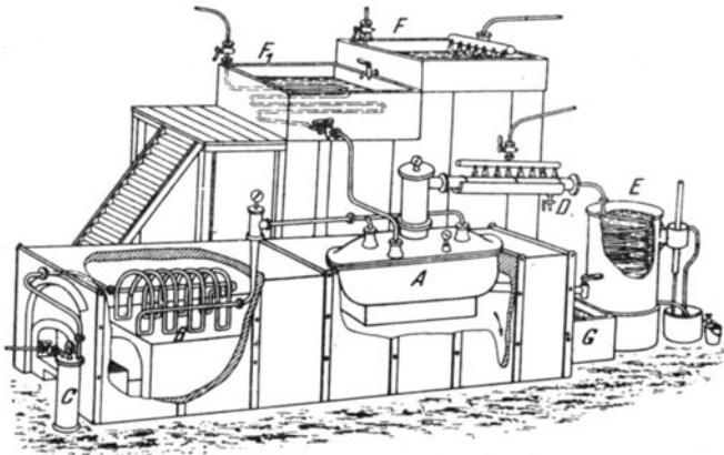
Fig. 154. Destillationsanlage nach holländischem Muster.
