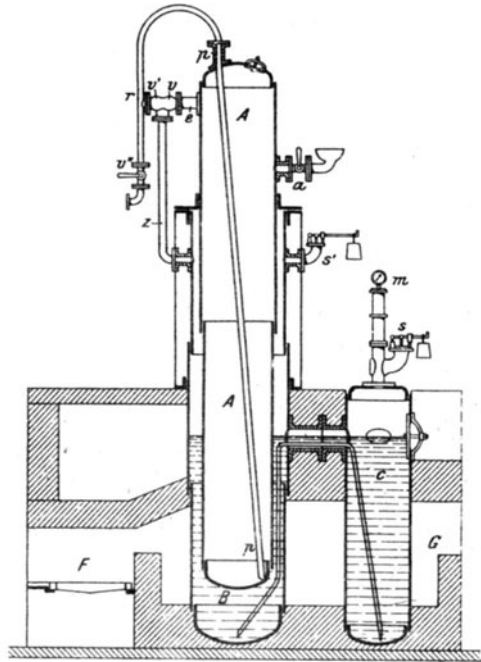
Fig. 103. Apparat von Droux.
