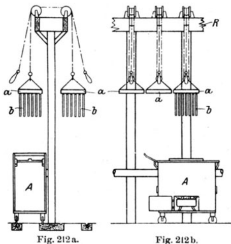
Fig. 212 a und b. Vorrichtung zum Kerzentunken.
