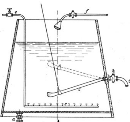
Fig. 7. Schmelzbottich für Premier-jus-Bereitung.
