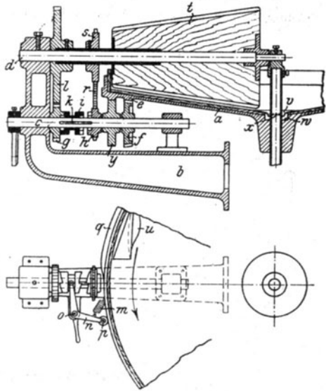
Fig. 45. Tellerknetzer nach Fischer.
