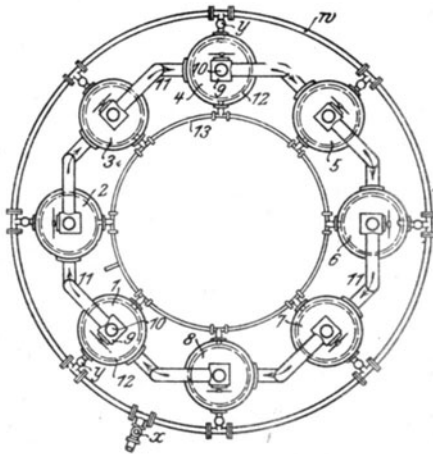
Fig. 61. Desodorisierapparat von Rocca.
