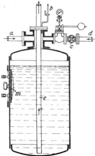
Fig. 95. Montejus.
