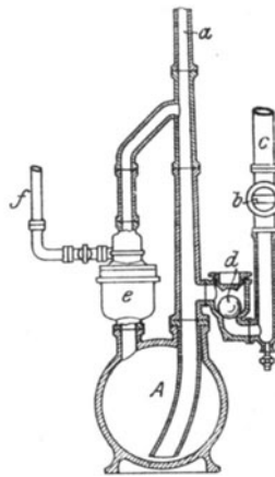
Fig. 97. Selbsttätig arbeitendes Monte- jus von Plath.
