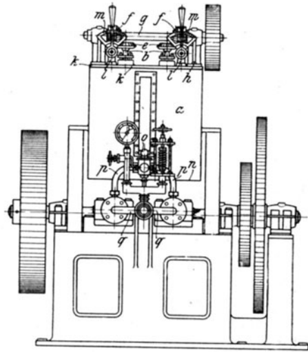
Fig. 24. Homogenisiermaschine „Schröder“.
