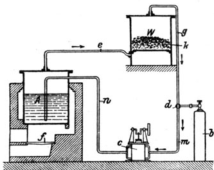
Fig. 198. Apparat zur Herstellung von Fettsäureamiden.
