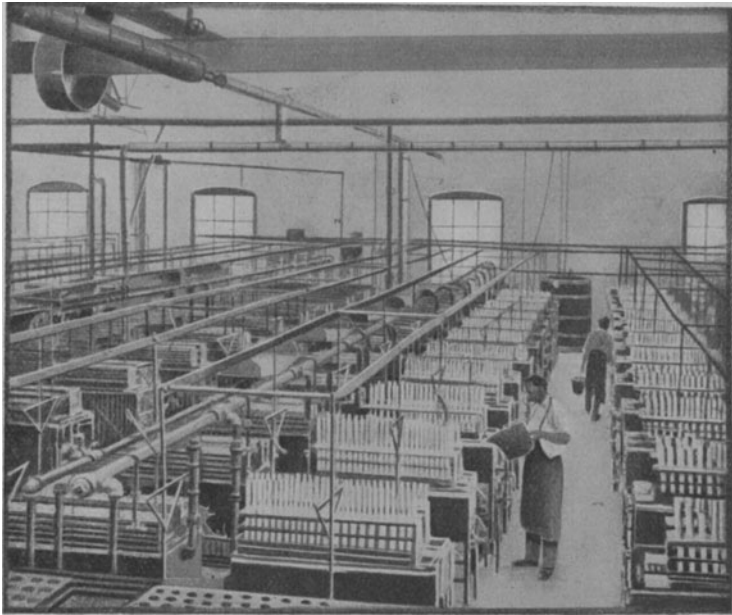
Fig. 289. Gießsaal einer Kerzenfabrik.
