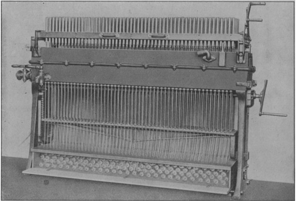
Fig. 238. Kerzengießmaschine mit 200—300 Formen.
