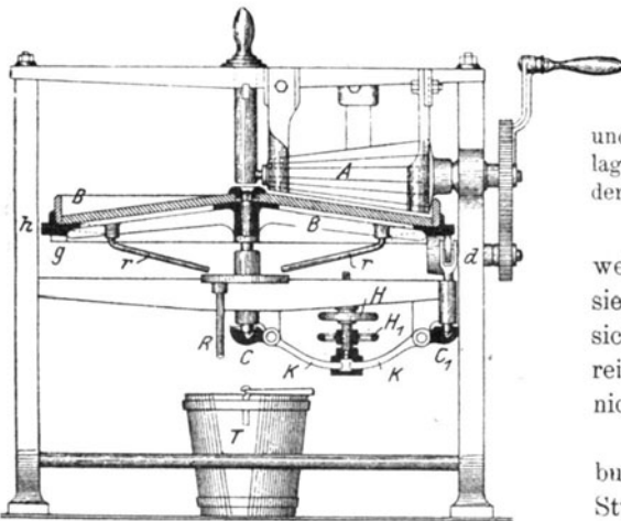
Fig. 42. Butterkneter nach Dürkoop & Co.
