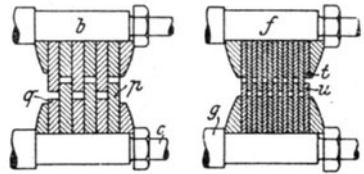
Fig. 4. Konstruktion der Schneidwalzen der Langeschen Rohthalgzerkleinerungsmaschine.
