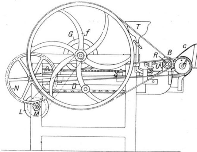
Fig. 258 c. Fig. 258 a—c. Kerzenpoliermaschine nach Daviron.
