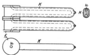
Fig. 150. Detail des Slama'schen Überhitzers.
