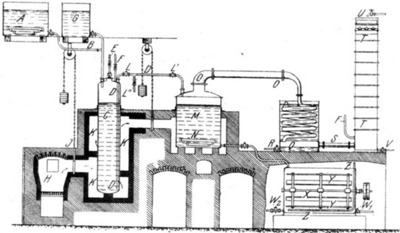
Fig. 101. Verseifungsanlage nach Violette und Buisine.
