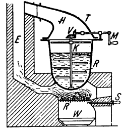
Fig. 75. Firniskochkessel nach Andres.
