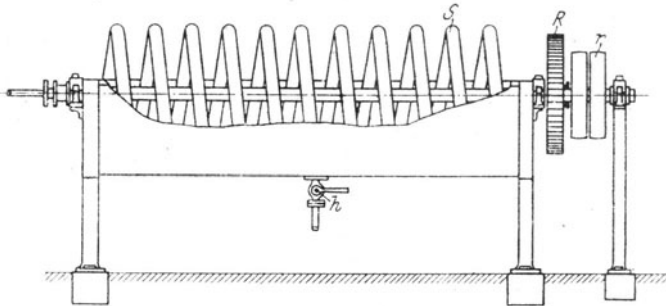
Fig. 127. Vorrichtung zum Konzentrieren des Glycerinwassers.
