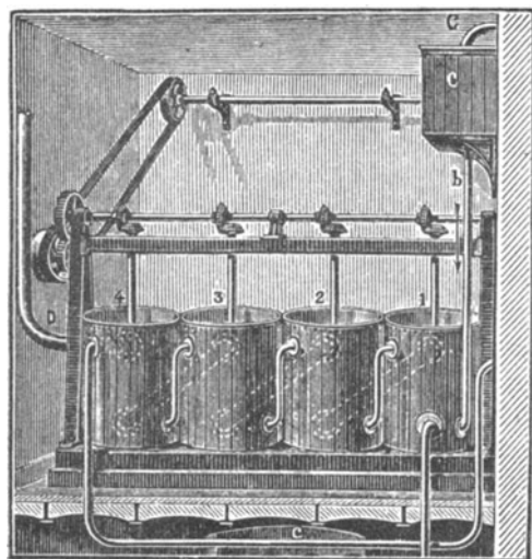
Fig. 181. Ölsäurekühlapparat nach Engelhardt.
