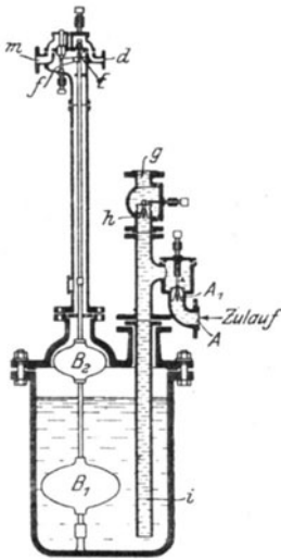
Fig. 96. Selbsttätig arbeitendes Monte- jus von Paul Schütze & Co.
