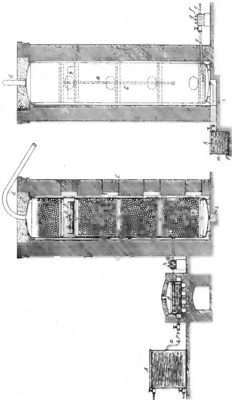
Fig. 110b. Schnitt \nu\nu_1 der Fig. 109.
