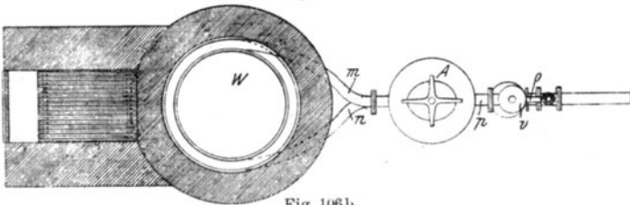
Fig. 106 a und b. Fettspaltungsapparat von L. Hugues.
