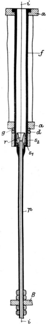
Fig. 225. Moderne Form für das Gießen von Stearinkerzen.
