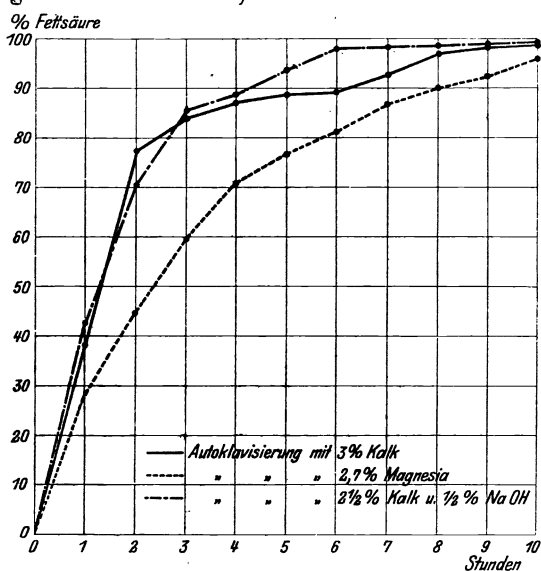
Fig. 120. Graphische Darstellung des Verlaufes des Autoklavenprozesses.
