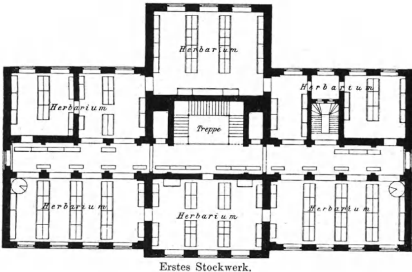
Erstes Stockwerk.
