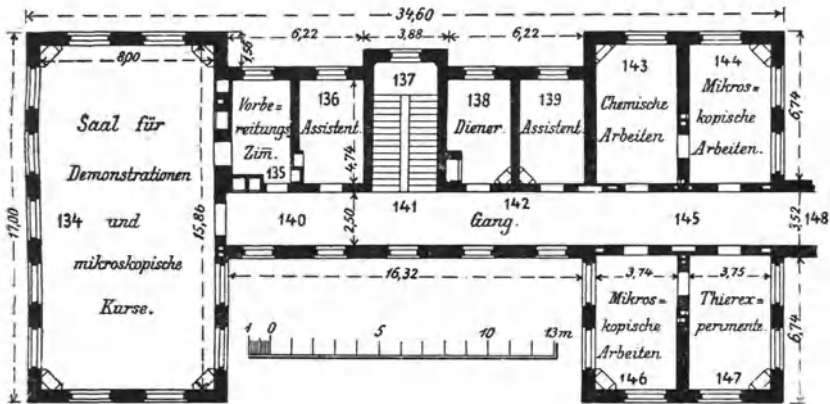
Erstes Stockwerk.
