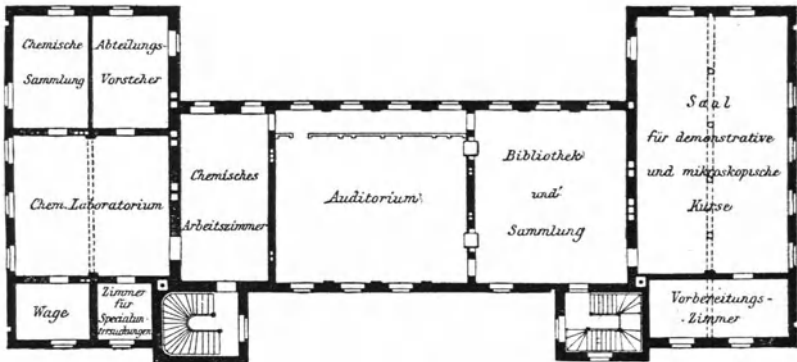
Erstes Stockwerk.
