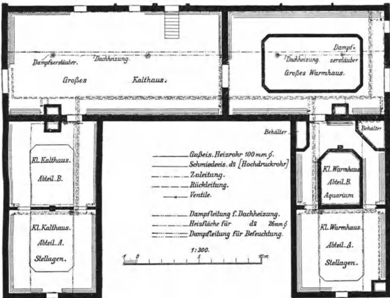
Heizungsanlagen der Gewächshausbauten.
