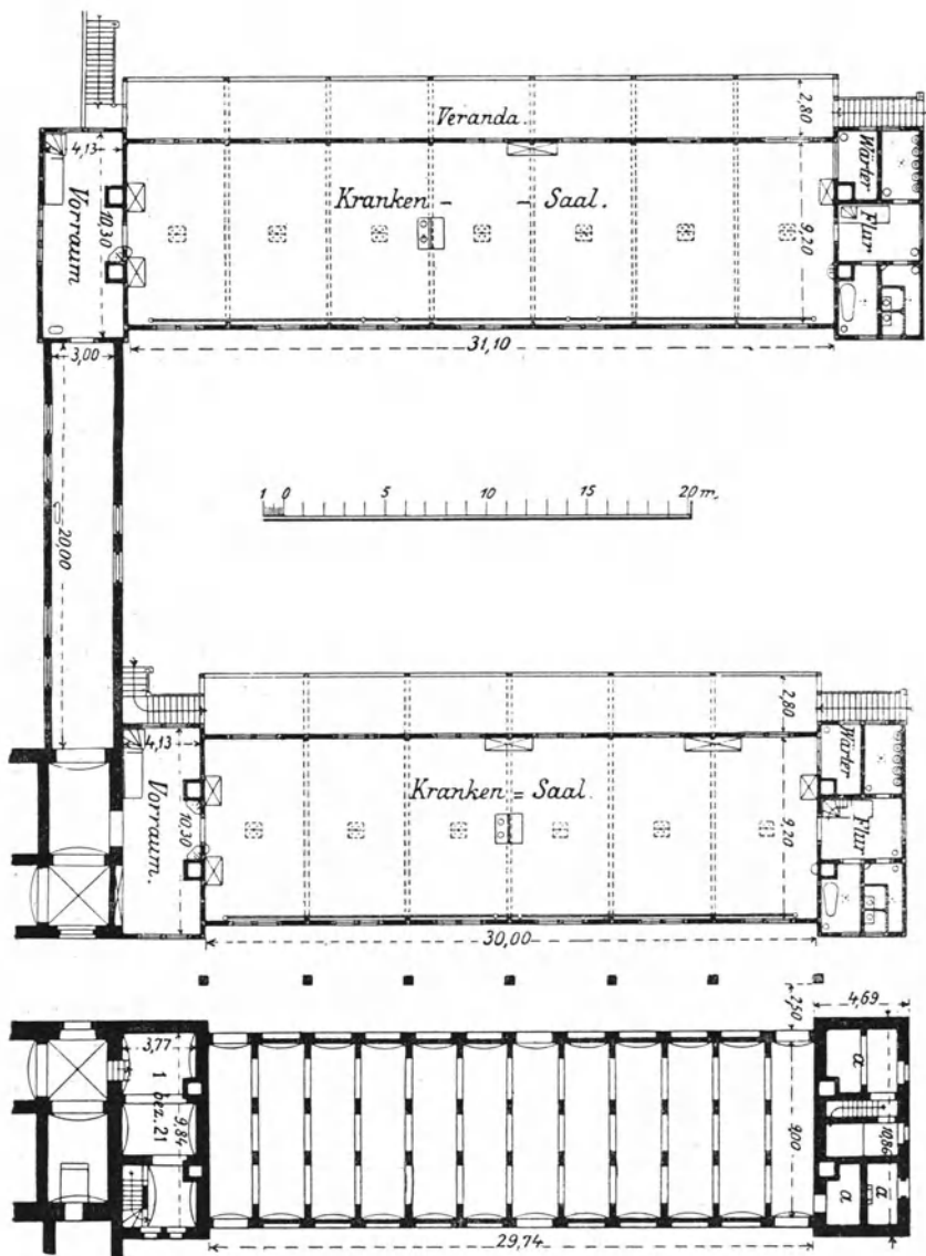
Block 1—3 und Unterbau.
