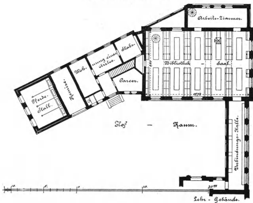
Bibliotheks-Gebäude.
