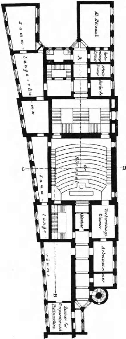
Erstes Stockwerk.
