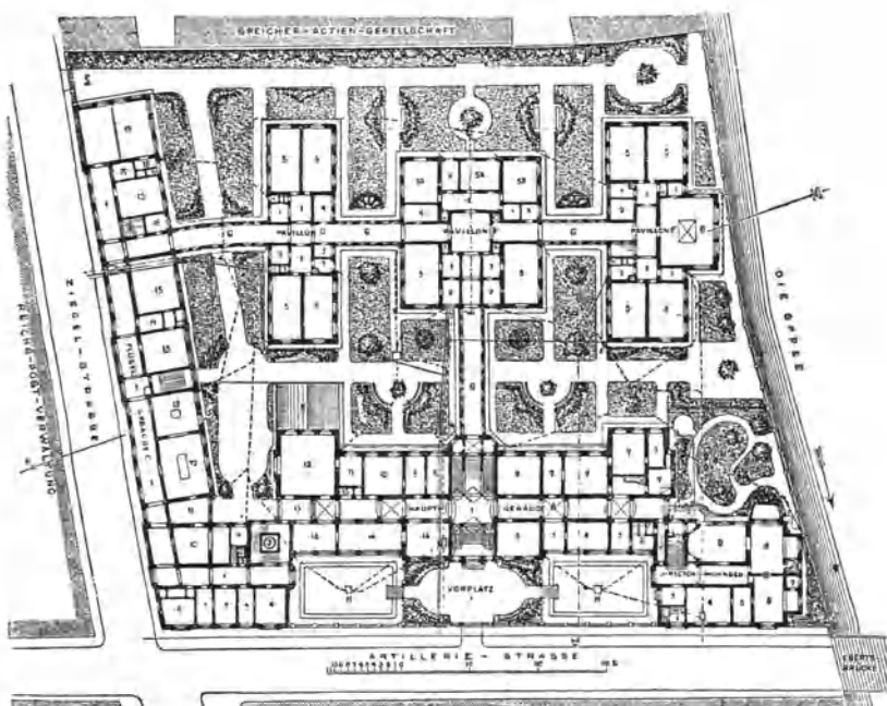
Lageplan.
