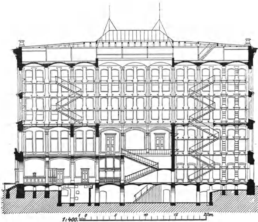
Querschnitt.
