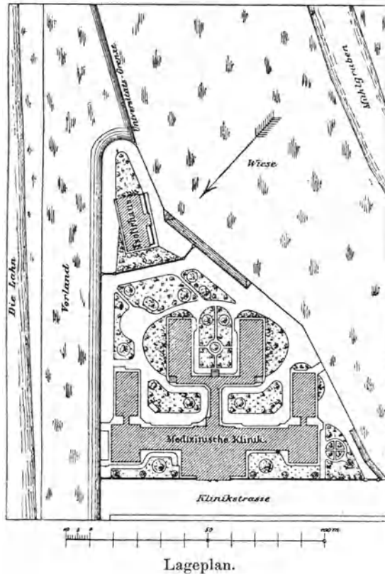
Lageplan.
