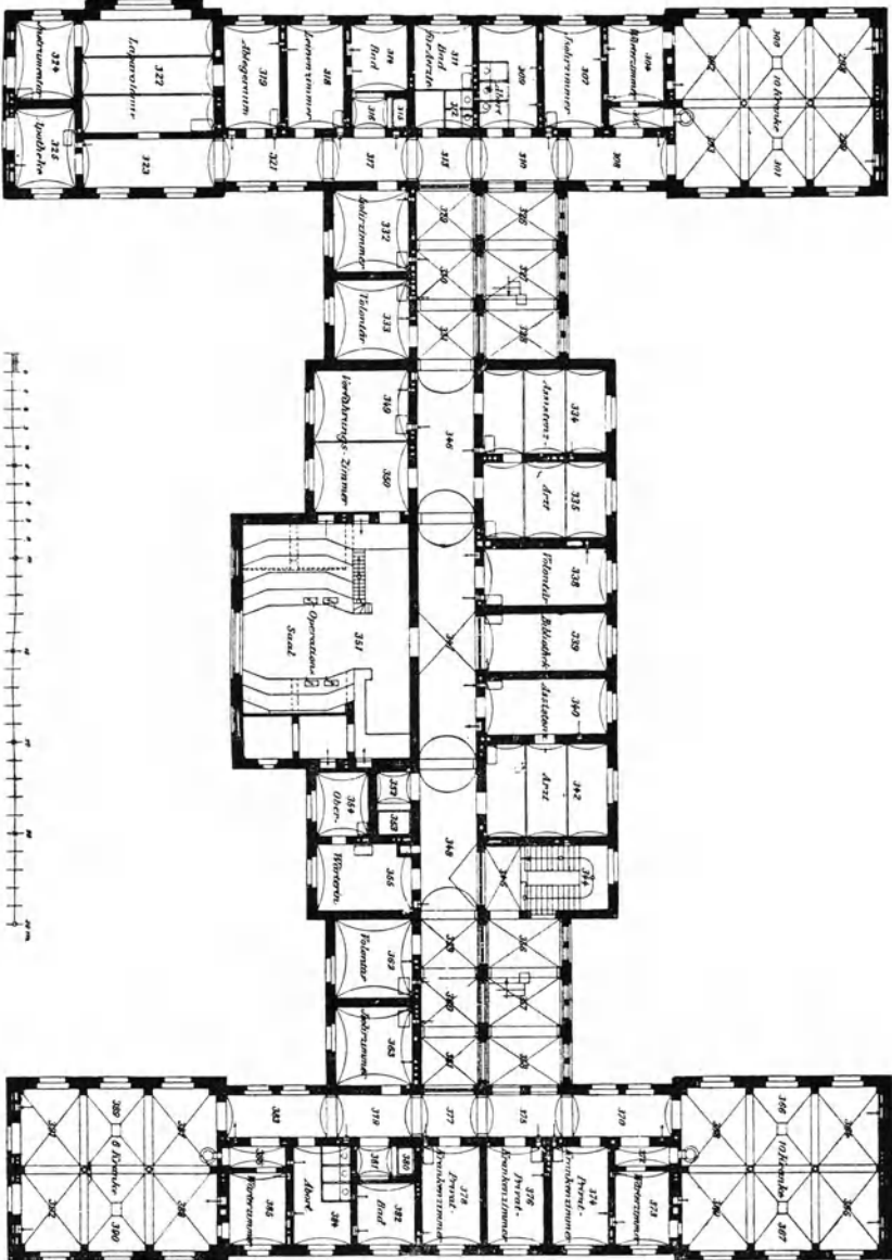
Erstes Stockwerk.
