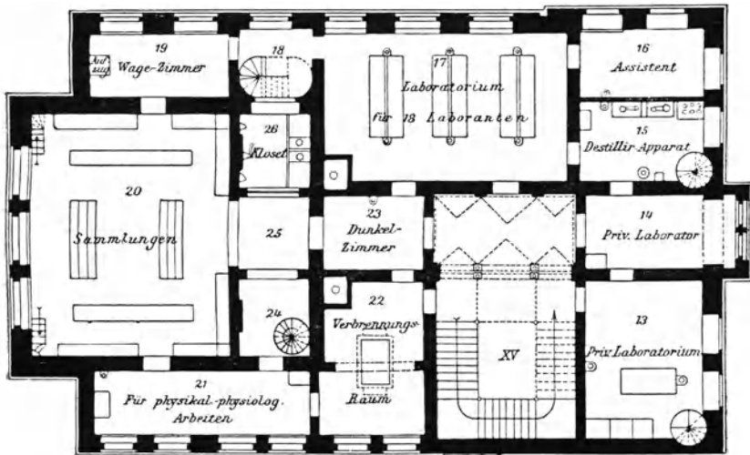
Erstes Stockwerk.
