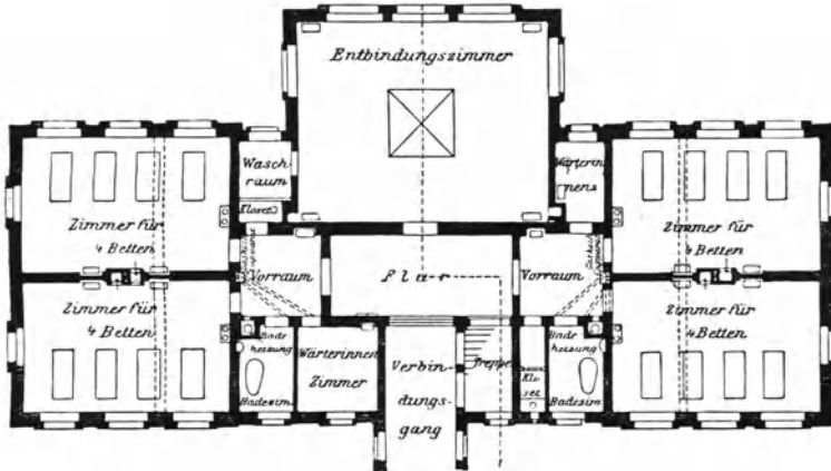
Pavillon F.
