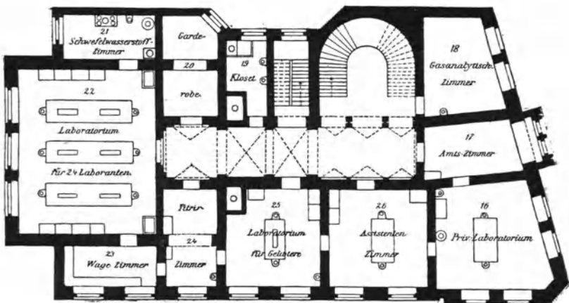
Erstes Stockwerk.
