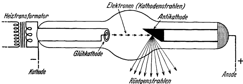
Abb. 1. Röntgenröhre.
