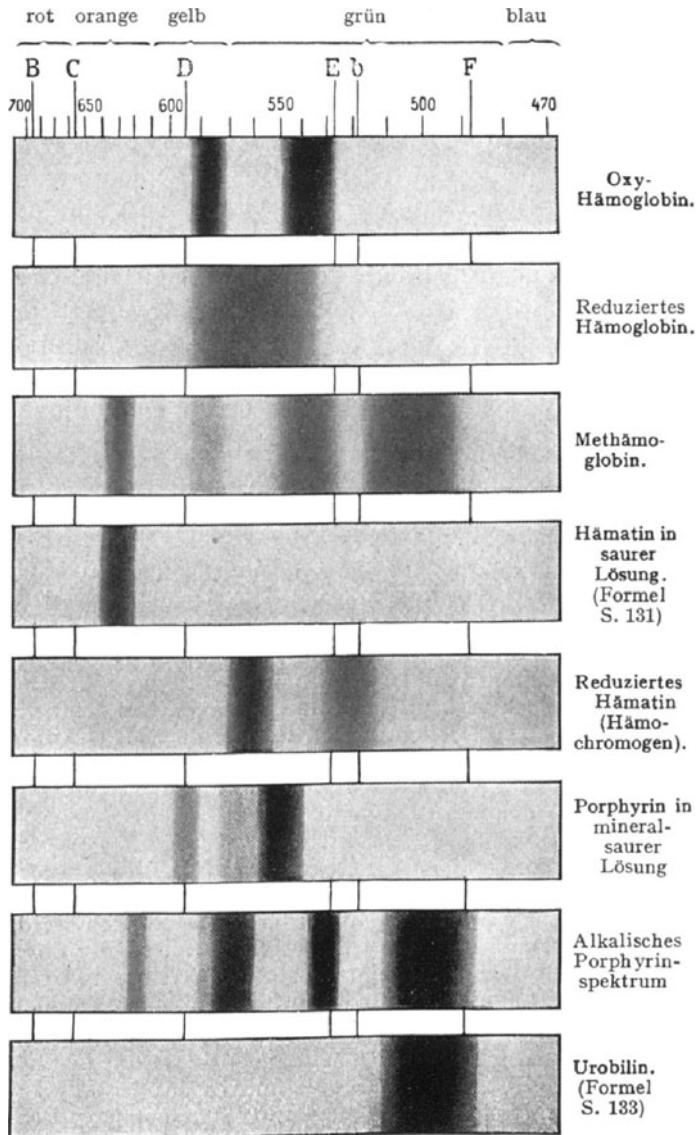
Abb. 58. Spektraltafel.
