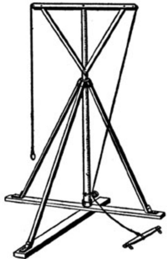
HAY DERRICK
