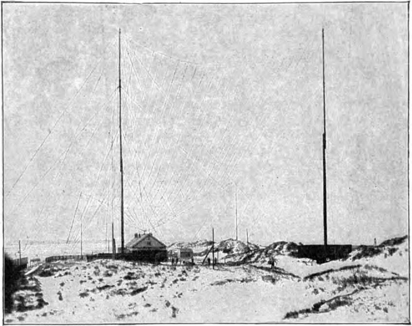
Figur 14. Luftleitergebilde, Scheveningen.
