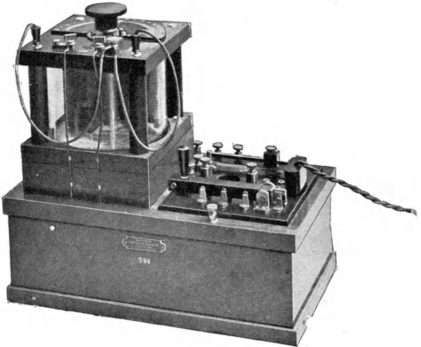
Figur 4. H.Z.M.-Apparat.
