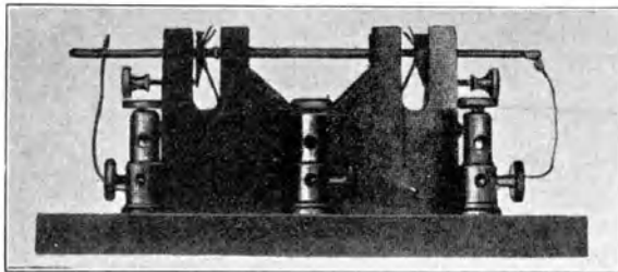
Figur 22. Kontaktkohärer.
