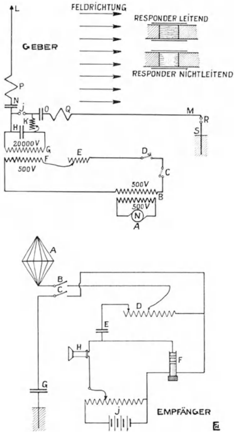
Figur 25. De Forest-Geber und Empfänger.
