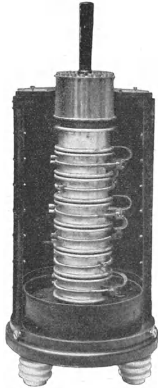
Figur 12. Sechsfach unterteilte Funkenstrecke.
