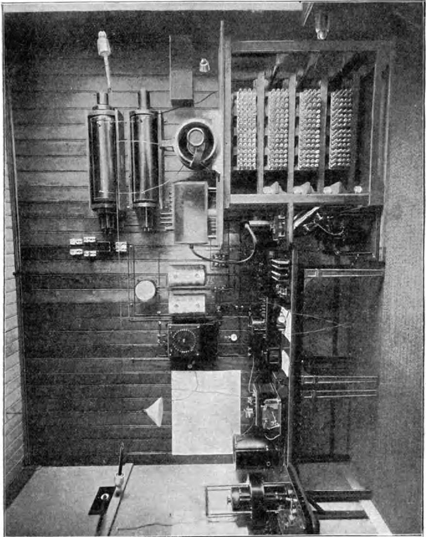
Figur 15. Inneres der Funkenbude, Scheveningen.
