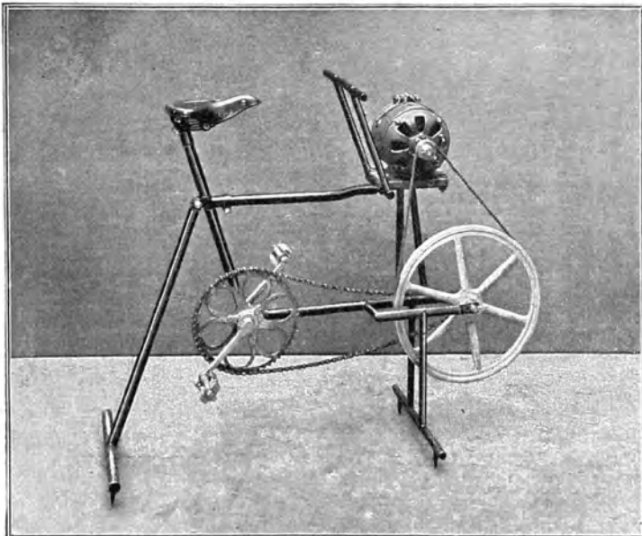
Figur 7. Tretynamo.
