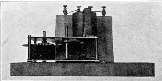
Figur 20. Elektromagnetischer Fessenden-Detektor.
