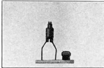
Figur 18. Bolometer-Konstruktion.
