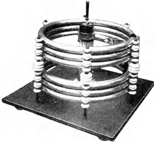
Figur 9. Selbstinduktion für 1000 km-Station.
