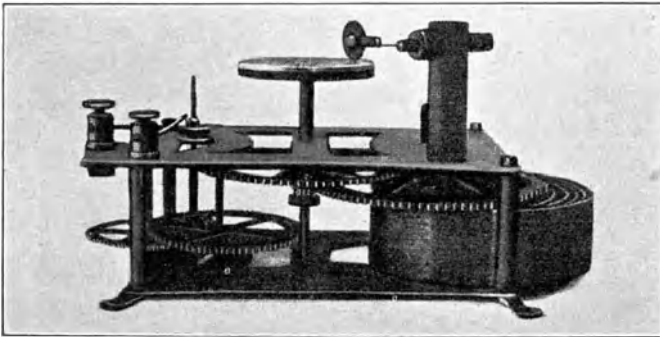
Figur 24. Rotierende Kohärervorrichtung.
