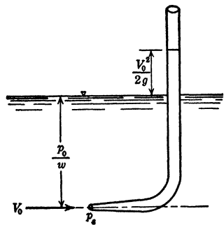
FIG. 146. Pitot Tube.
