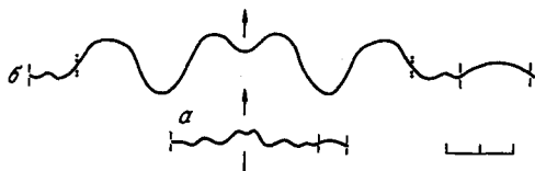
Рис. 54. Перегородочная линия Proclydonautilus kiparisovae Popov, \times 0,66 . Голотип № 32/5925: а — D=21 мм; б — D=65 мм (по Ю. Н. Попову [1959]).
