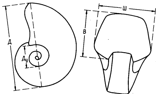
Рис. 2. Основные меристические признаки раковины наutilus. Д — диаметр раковины; В — высота оборота; Ш — ширина оборота; D_y — диаметр умбиликуса.
