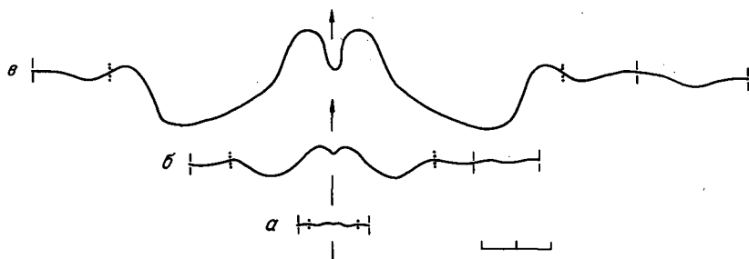
Рис. 56. Перегородочные линии Proclydonautilus anianiensis (Shimansky), \times 0,5 . а, б — экз. 759/246: а — 1 оборот при V=7,0 мм, Ш=8,0 мм; б — 2 оборота при V=32,0 мм, Ш=33,0 мм; в — экз. 759/243: 2\frac{1}{2} оборота при V=66,0 мм, Ш=54,0 мм.
