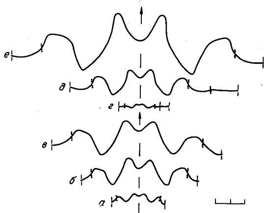
Рис. 58. Перегородочные линии Cosmonautilus polaris sp. nov., \times 0,5 .
