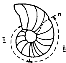
Рис. 14. Схематичное изображение эмбриональной раковины триасовых наутилид.
