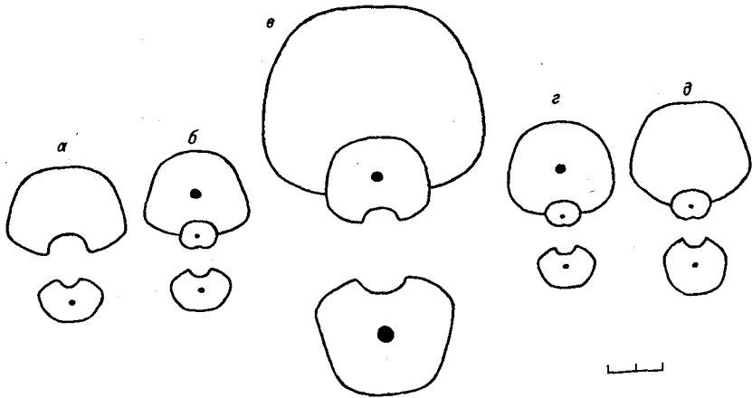
Рис. 62. Поперечные сечения раковин Cenoceras boreale Dagys et Sobolev, \times 0,5 .
