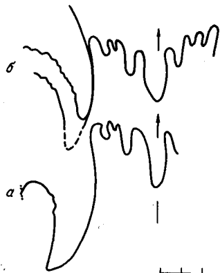
Рис. 61. Перегородочные линии Yakutionautilus angulatus (Popow), \times 0,5 .
