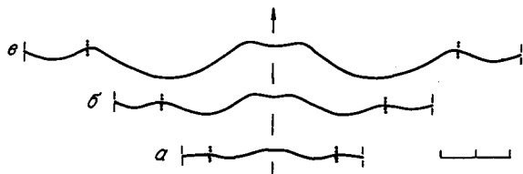
Рис. 47. Перегородочные линии Gryponautilus kegalensis sp. nov., \times 0,5 .
