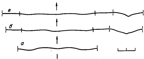
Рис. 51. Перегородочные линии Tomronautilus setorymi sp. nov., \times 0,5 .
