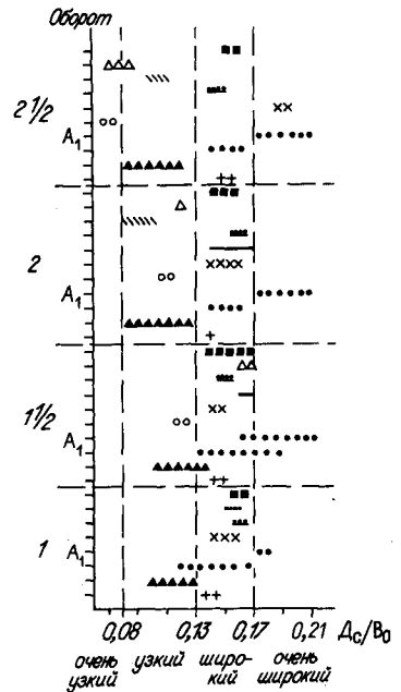
Рис. 10. Изменение относительной ширины сифонов в онтогенезе у некоторых родов триасовых наutilus. Усл. обозн. см. на рис. 8.
