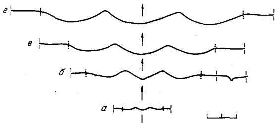
Рис. 20. Перегородочные линии Germanonautilus porowi sp. nov., \times 0,5 .
