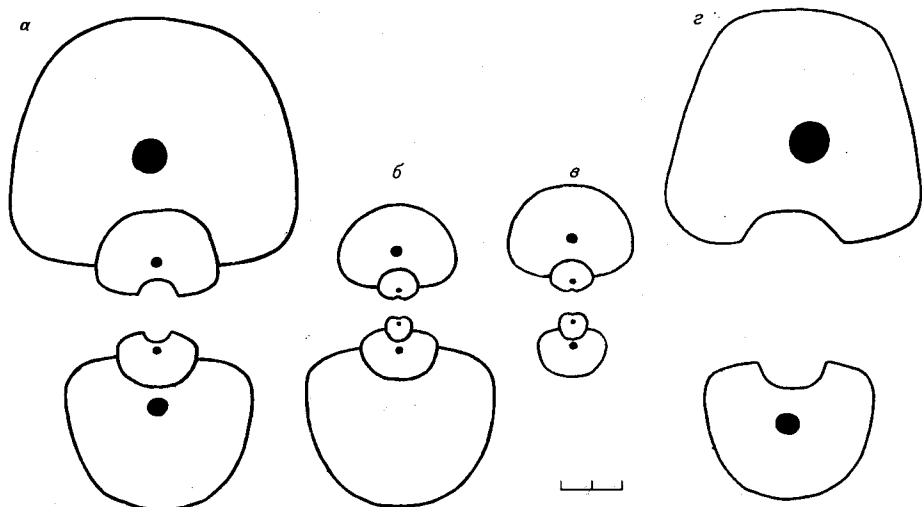
Рис. 43. Поперечные сечения раковин Arctonautilus egorovi sp. nov.
