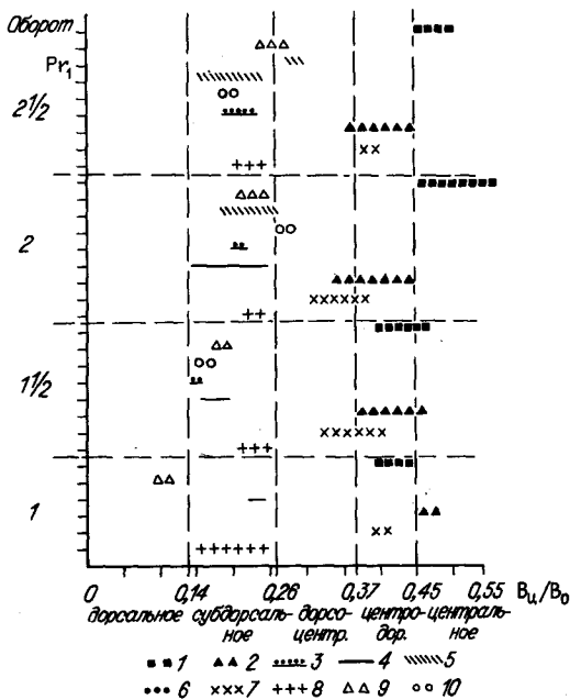
Рис. 8. Изменение положения сифона в онтогенезе у триасовых наutilus.
