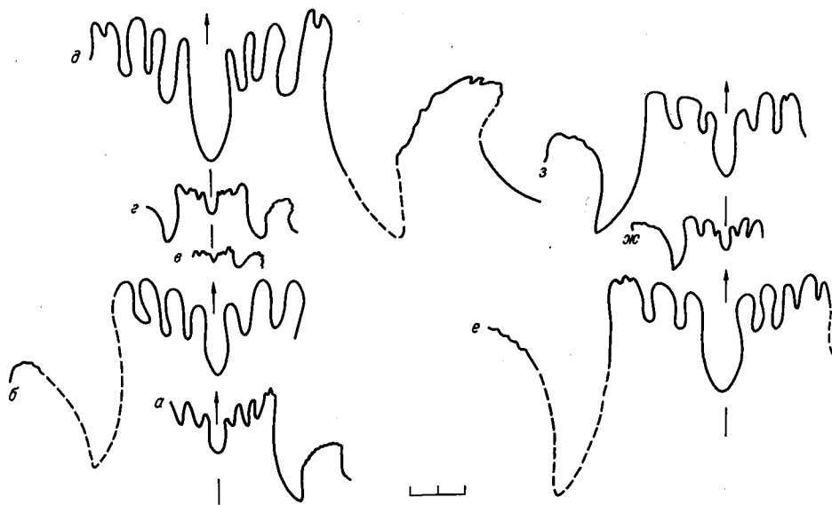
Рис. 60. Перегородочные линии Yakutionautilus kavalerovae Arkhipov et Barskov, \times 0,5 .
