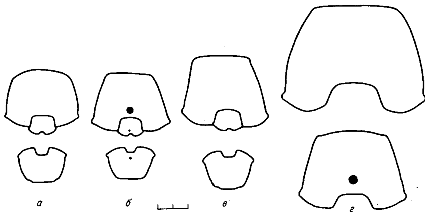
Рис. 19. Поперечные сечения раковин Germanonautilus porowi sp. nov., \times 0,5 .
