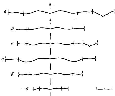
Рис. 25. Перегородочные линии представителей рода Sibyllonautilus , \times 0,5 .
