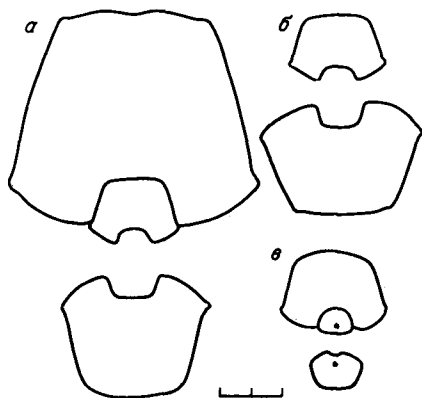
Рис. 17. Поперечные сечения раковин Germanonautilus kyotanii Nakazawa, \times 0,5 .
