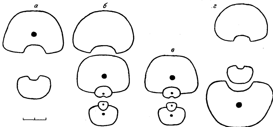
Рис. 38. Поперечные сечения раковин Arctonutilus ljubovae (Schastlivtceva), \times 0,5 . а — экз. № 759/72 ( 1\frac{1}{2} , 2 оборота); б — голотип № 1473/10 ( 1\frac{1}{2} , 1, 1\frac{1}{2} , 2, 2\frac{1}{3} оборота); в — экз. 759/62 ( 1\frac{1}{2} , 1, 1\frac{1}{2} , 2 оборота); г — экз. 759/74 ( 1\frac{1}{2} , 2, 2\frac{1}{3} оборота).
