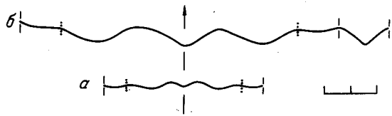
Рис. 41. Перегородочные линии Arctonautilus spatiosus sp. nov., \times 0,5 .
