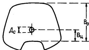
Рис. 3. Измерения основных параметров при определении положения и относительной ширины сифона.
