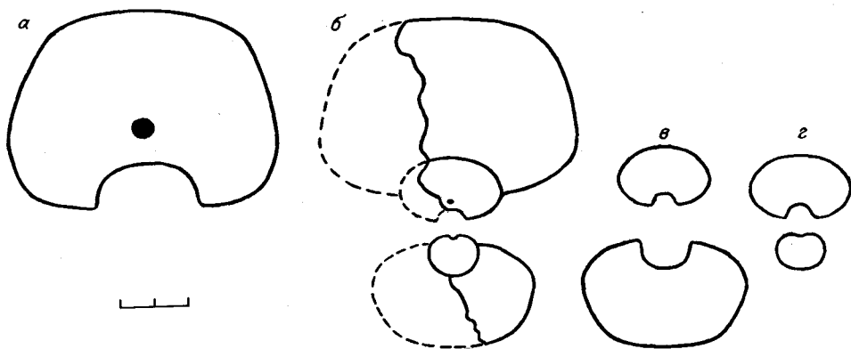
Рис. 50. Поперечные сечения раковин Tomponautilus setorymi sp. nov., \times 0,5 . а — экз. № 759/184 ( 2\frac{1}{2} оборота); б — экз. 759/200 (1, 1\frac{1}{2} , 2, 2\frac{1}{2} оборота); в — экз. 759/189 ( 1\frac{1}{2} , 2 оборота); з — экз. 759/193 (1, 1\frac{1}{2} оборота).
