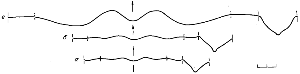
Рис. 45. Перегородочные линии представителей рода Arctonutilus , \times 0,5 .
