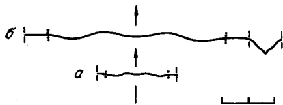
Рис. 16. Перегородочная линия Anoploceras taimyrensis (Schastlivtceva), \times 0,5 . Голотип № 1473/11; а — 1 \frac{1}{2} оборота при V=9,5 мм, III=14,0 мм; б — 2 \frac{1}{2} оборота при V=27 мм, III=38 мм.
