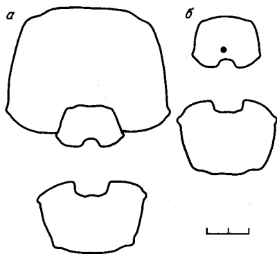
Рис. 21. Поперечные сечения раковин Germanonautilus sibiricus sp. nov., \times 0,5 . а — голотип № 759/114 (1 \frac{1}{2} , 2, 2 \frac{1}{2} оборота); б — экз. 759/110 (1 \frac{1}{2} , 2 оборота).
