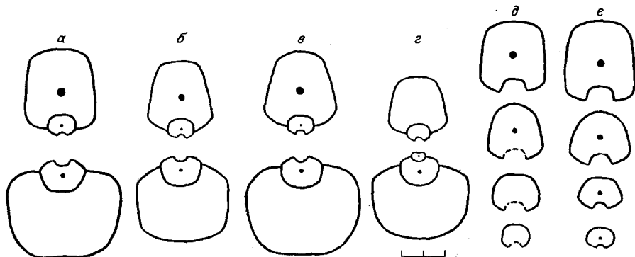
Рис. 26. Поперечные сечения раковин Phaedrysmocheilus subaratus (Keyserling), \times 0,5 . а — экз. 750/4 ( 1^{1/2} , 2, 2^{1/2} , 3 оборота); б — экз. 750/7 ( 1^{1/2} , 2, 2^{1/2} , 3 оборота); в — экз. 750/12 ( 1^{1/2} , 2, 2^{1/2} , 3 оборота); г — экз. 759/42 (1, 1^{1/2} , 2, 2^{1/2} , 3 оборота); д — экз. 750/4 ( 1^{1/2} , 2, 2^{1/3} , 2^{1/2} оборота); е — экз. 750/6 ( 1^{1/2} , 2, 2^{1/3} , 2^{1/2} оборота).
