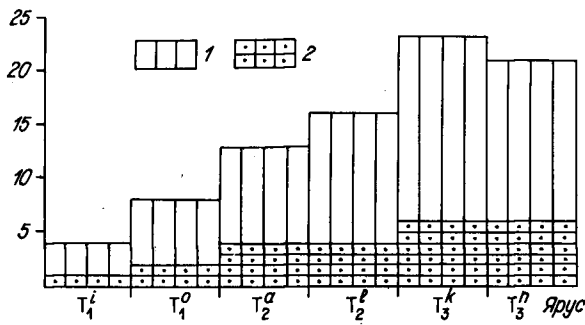
Рис. 64. Количество родов наутилид в триасовых палеоакваториях. 1 — тетическая область, 2 — бореальная.
