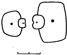
Рис. 15. Поперечное сечение раковины Anoploceras taimyrensis (Schastlivtceva), \times 0,5 . Голотип № 1473/11 (1, 1 \frac{1}{2} , 2, 2 \frac{1}{2} оборота). Перечень оборотов идет от начала раковины.
