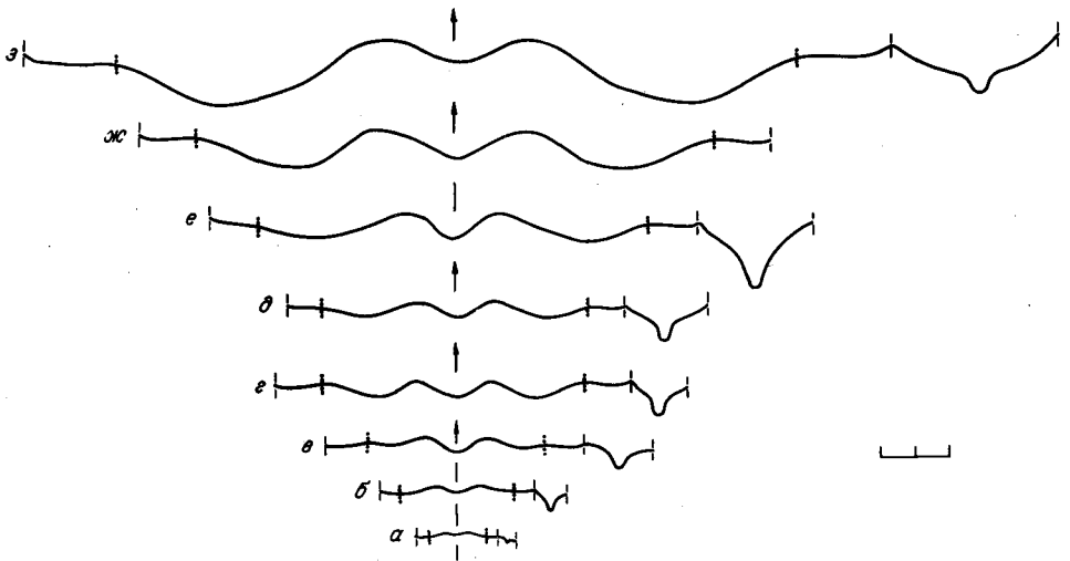
Рис. 44. Перегородочные линии Arctonautilus egorovi sp. nov., \times 0,5 .
