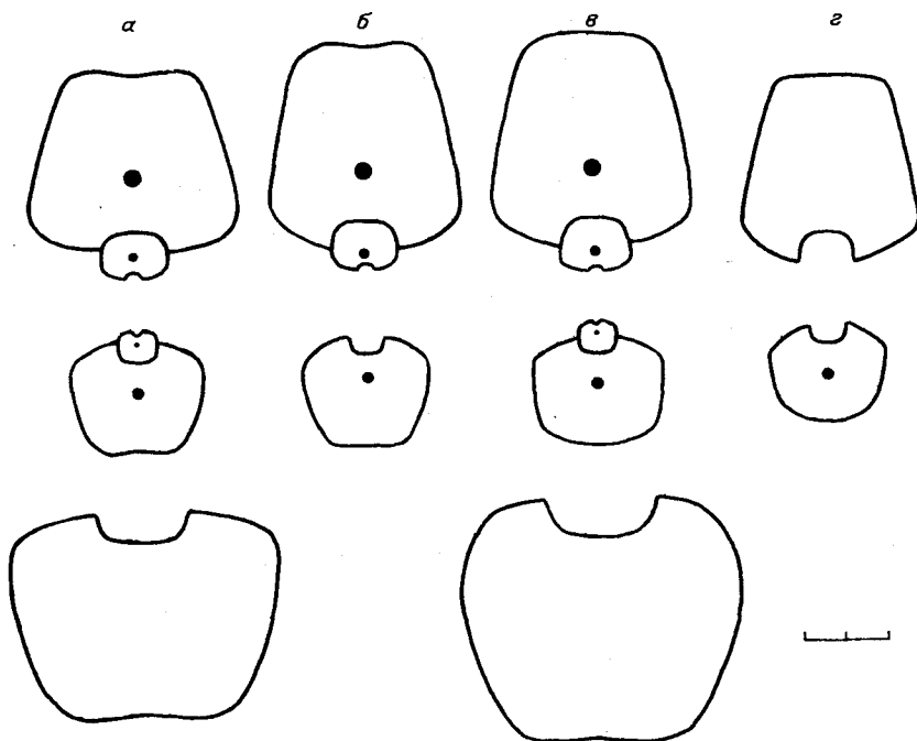
Рис. 28. Поперечные сечения раковин Phaedrysmocheilus nestori (Shimansky), \times 0,5 . а — экз. 758/24 (1, 1^{1/2} , 2, 2^{1/2} , 2^{2/3} оборота); б — экз. 759/31 ( 1^{1/2} , 2, 2^{1/2} оборота); в — экз. 759/25 (1, 1^{1/2} , 2, 2^{1/2} , 2^{2/3} оборота); г — экз. 759/32 (2, 2^{1/2} оборота).
