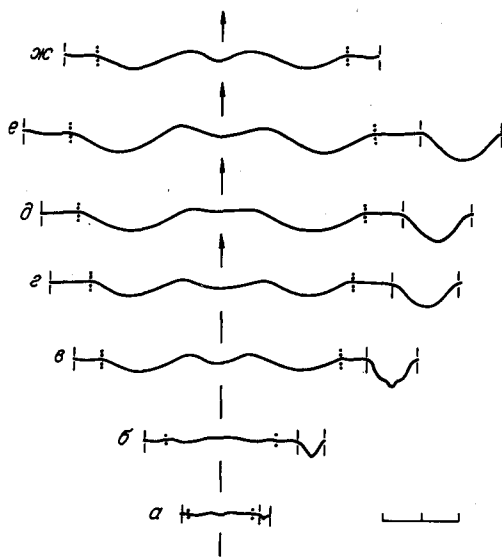
Рис. 33. Перегородочные линии Phaedrysmocheilus involutus sp. nov., \times 0,5 .
