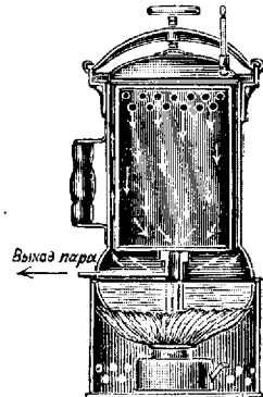
Рис. 6. Схематический разрез автоклава для стерилизации в текущем пару.
