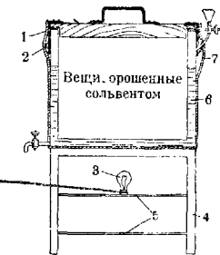
Рис. 7. Ящик Окуневского для быстрого обеззараживания одежды парами сольвента или парами смеси сольвента и бензина (1:3): 1—прокладка; 2—элементы; 3—угольная электролампа на 100—150 свечей; 4—ящик из-под тары; 5—полочка; 6—горячая вода; 7—чехол из ткани.
