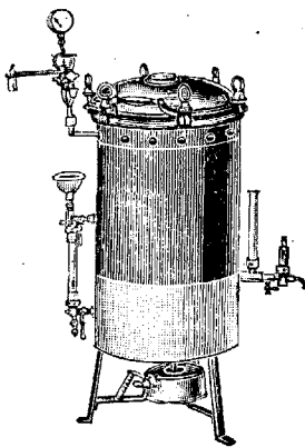
Рис. 2. Вертикальный автоклав (стандартный).
