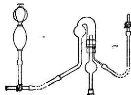
Рис. 7. Прибор Стеффанутти.
