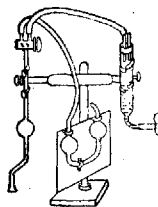
Рис. 3. Аппарат Шеменского.
