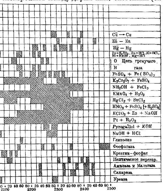
Диаграмма спектров митогенетического излучения различных химических источников.
