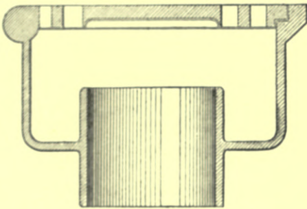
Fig. 332.—Cregeen's Air-inlet Cover.
