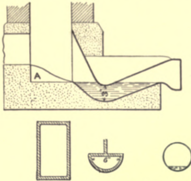
Fig. 371.—Slagg's Intercepting Trap.
