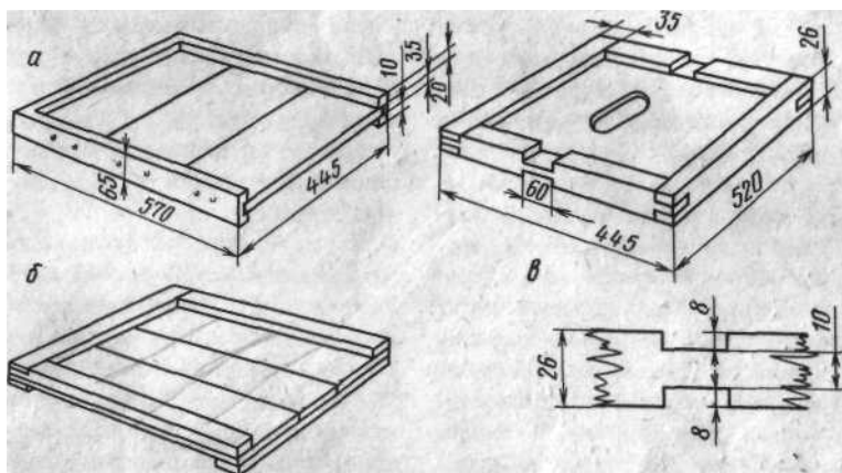
112. Дно улья:
