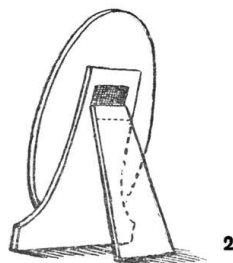
Рамка для фотографии: 1 — общий вид рамки; 2 — крепление ножки.
