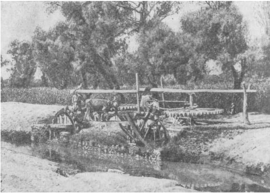
Сакиа — приспособление для орошения. К вертикальному колесу (на переднем плане) прикреплены кувшины. При вращении колеса они черпают воду из водоема и выливают ее в деревянный лоток, откуда она стекает на поля. Сакию приводят в движение быки.
