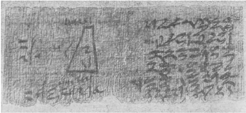
Задача на вычисление объема усеченной пирамиды из Московского математического папируса.
