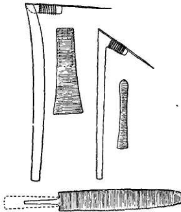
Медные тесла с деревянными рукоятками и пила времени I династии.
