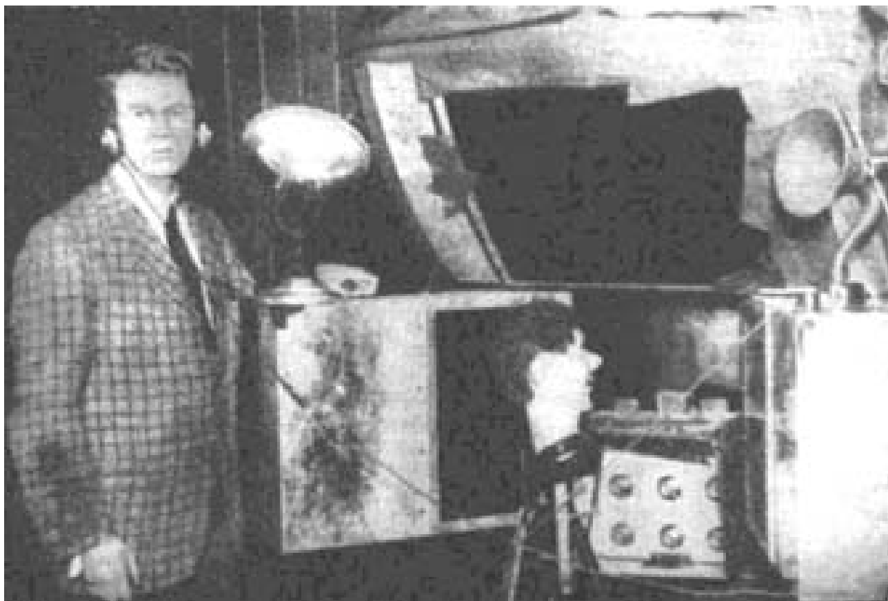
Механическая телевизионная система Дж. Берда. Фотография. 1930 г.
