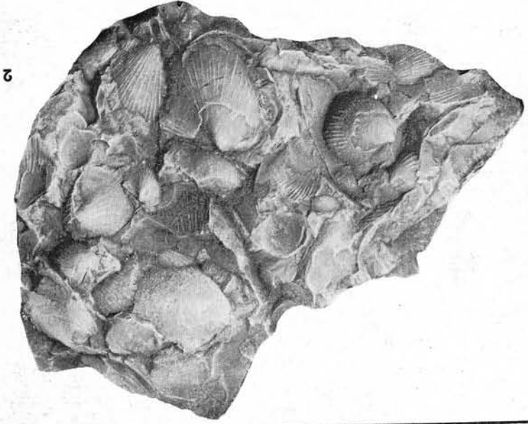
Aucella volgensis
