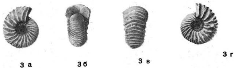
Speetoniceras inversumforme
