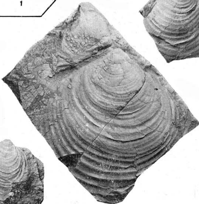
Inoceramus subneocorniensis
