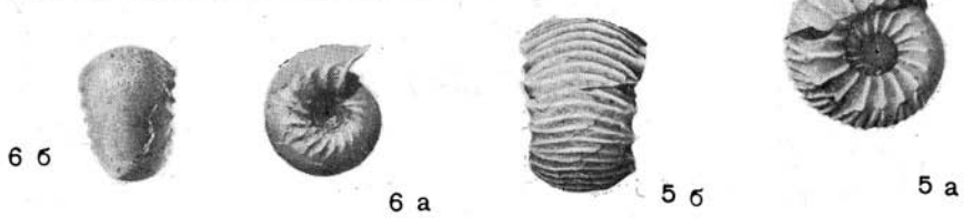
Speetoniceras coronatiforme
