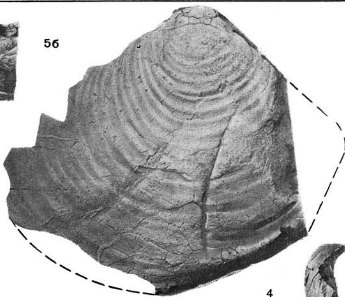
Inoceramus gusselkaensis
