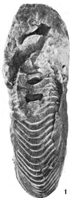
Craspedodiscus progredicus
