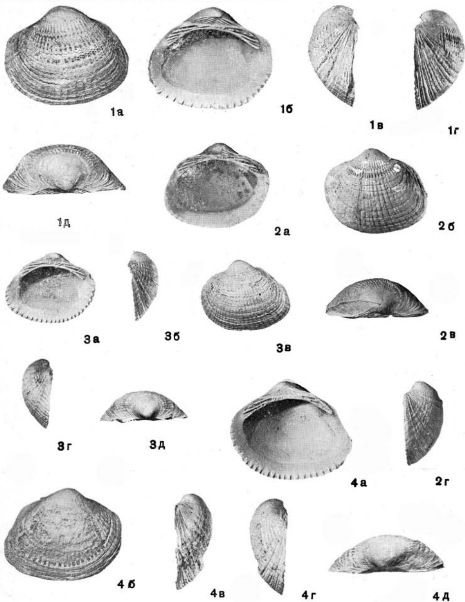
Cucullaea golowkinskii
