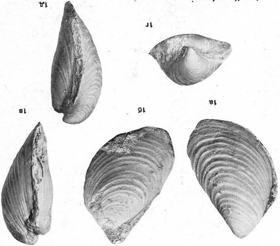
Aucella volgensis
