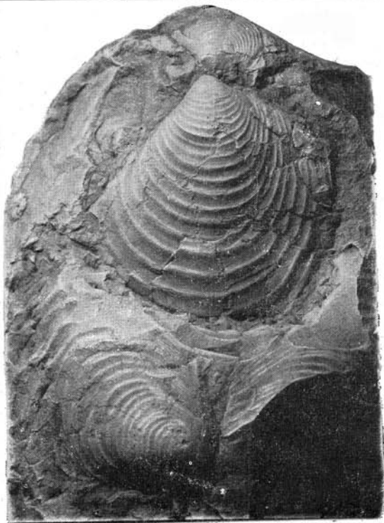
Inoceramus boreatis
