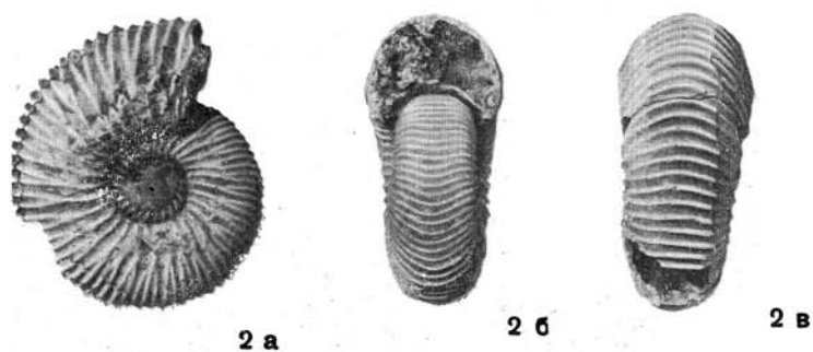
Speetoniceras inversumforme
