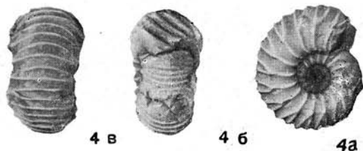
Speetonicerus versicolor
