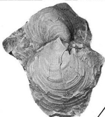
Inoceramus neocomiensis
