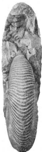
Craspedodiscus discofalcatatus
