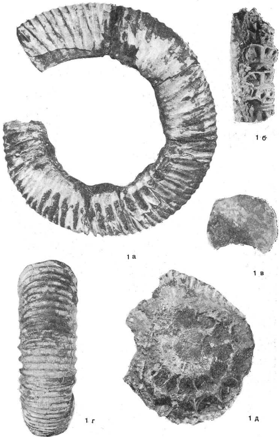
Speetoniceras subinversum
