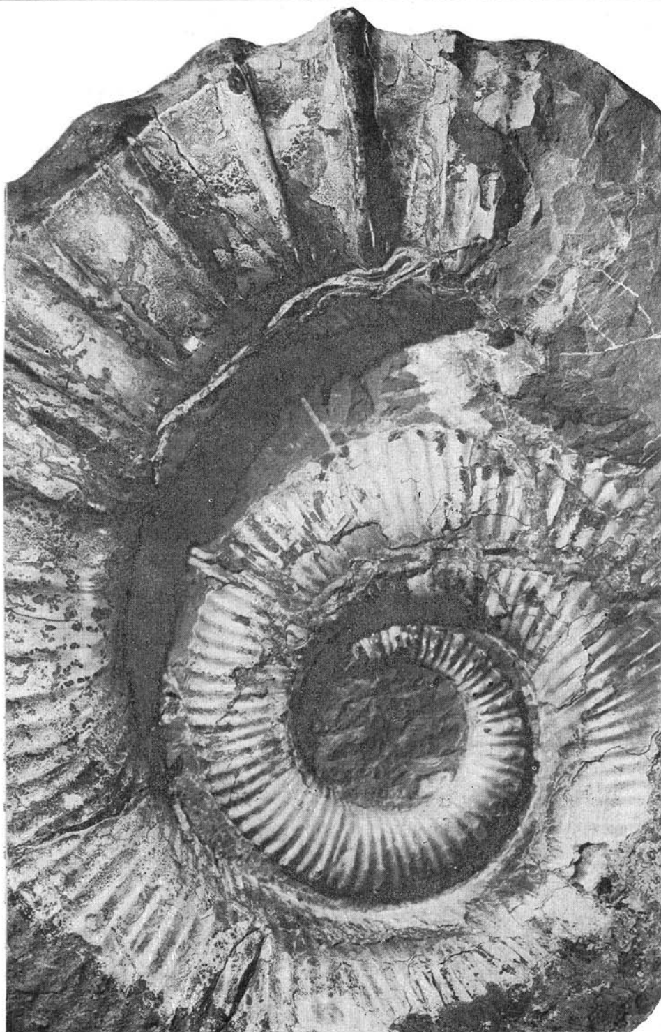
Australiceras simbirskense
