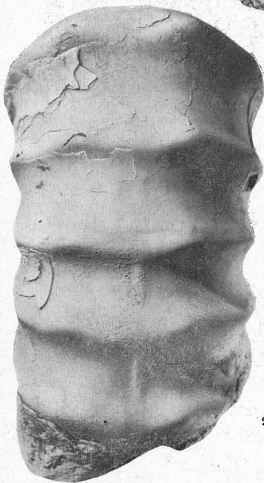
Australiceras simbirskense
