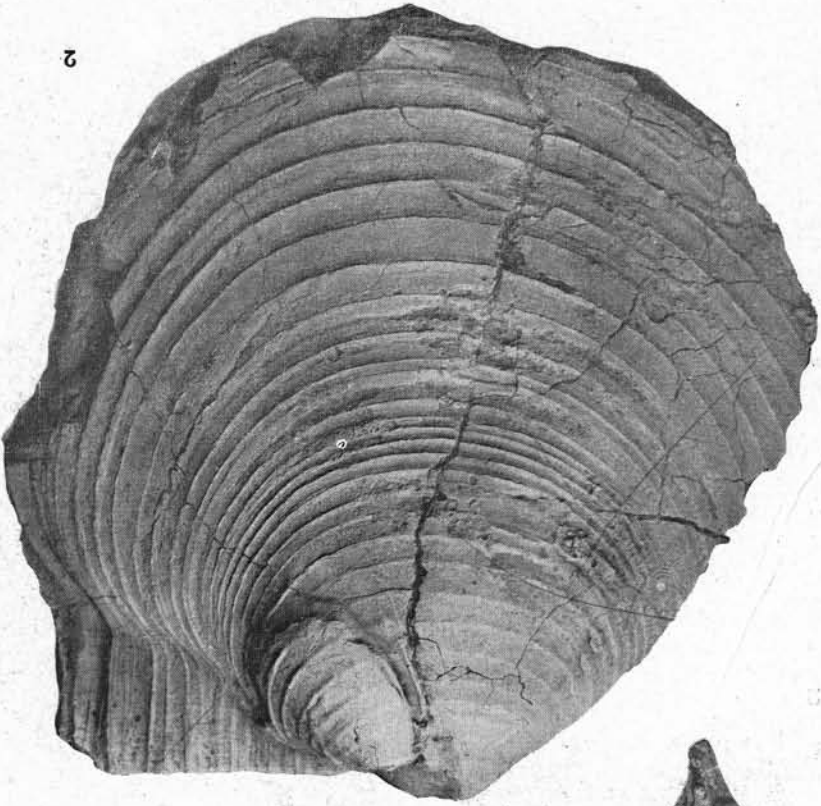
Camptonectes imperialis
