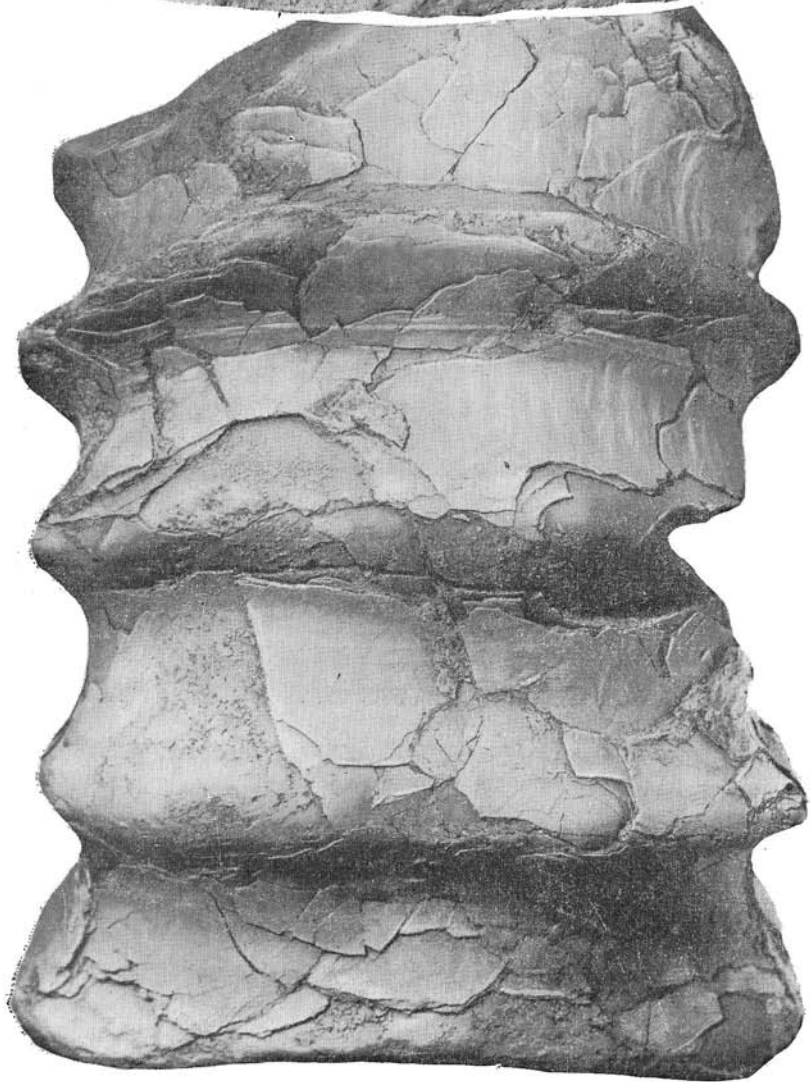
Australiceras apticum
