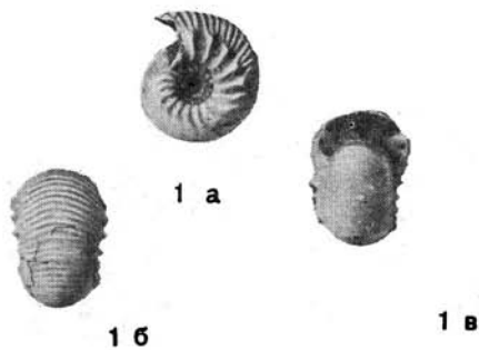
Simbirskites umbonatiformis
