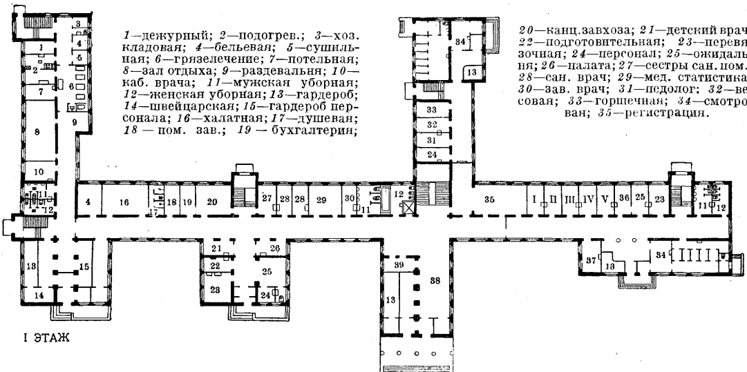
Типовой проект строительства Наркомздрава. Поликлиника на 15 000 посетителей.
