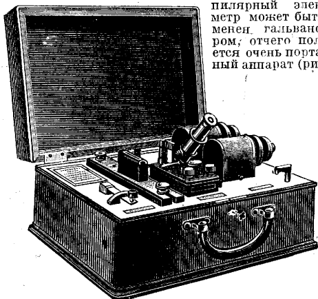
Рис. 5. Микроионметр Лаутеншлегера.
