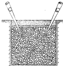
Рис. 7. Устройство окопного писсуара.
