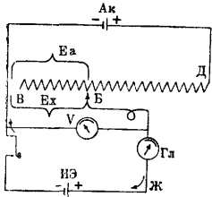
Рис. 1. Устройство потенциометра с вольтметром: Ак—аккумулятор; ИЭ—исследуемый элемент; Гл—гальванометр; V—вольтметр.
