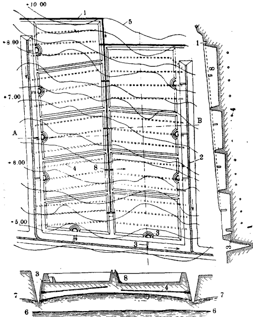
Рис. 1. План участка полей с горизонталями и со всеми необходимыми сооружениями: 1—разводные каналы; 2—осушительные каналы; 3—весенние выпуски; 4—дренаж; 5—горизонтали до устройства полей; 6—поверхность уровня грунтовых вод до орошения; 7—поверхность уровня грунтовых вод после орошения; 8—оросительные борозды.
