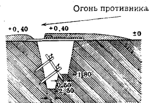
Рис. 5. Отхожее место в окопах.
