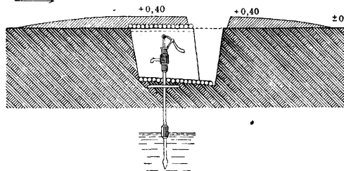
Рис. 4. Установка портоновского колодца в окопах.
