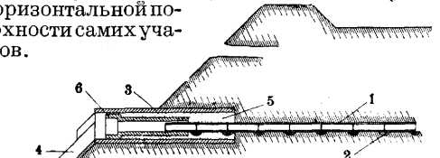
Рис. 4. Выпуск из дренажа в осушительную канаву: 1—дренажная гончарная труба; 2—слой глины; 3—деревянная труба; 4—спускной лоток; 5—засыпка из торфа; 6—гончарная труба.
