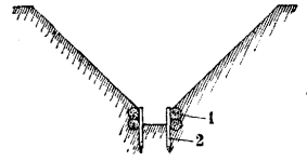
Рис. 11. Осушительная канава: 1—фашины; 2—свая.
