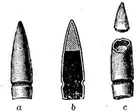
Рис. 6. Алюминиево-свинцовая английская пуля: а—снаружи; б—на распиле; с—при отломе верхушки (уменьшено).
