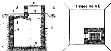
Рис. 1. Кирпичная яма размером 2,13 м × 2,13 м на 70 чел. Стены и дно (а)—в один кирпич, снаружи—слой глины (б); изнутри стены и дно оштукатуриваются цементным раствором. Сверху яма перекрывается решеткой (в). Надземная часть закрыта крышкой (г) с люком, устройство которого видно на рис. 2; 1—пространство между стенами по сводам, заполненное бетоном; 2—свод.
