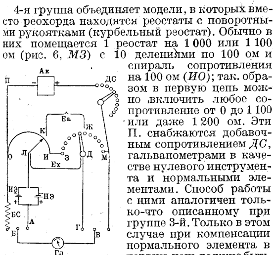
Рис. 6. Устройство потенциометра Мисловицера: Ак—аккумулятор; ИЭ—исследуемый элемент; НЭ—нормальный элемент; Гл—гальванометр; МЗ—реостат с делениями по 100 ом; ИО—проволока сопротивления; ДС—добавочное сопротивление к гальванометру.
