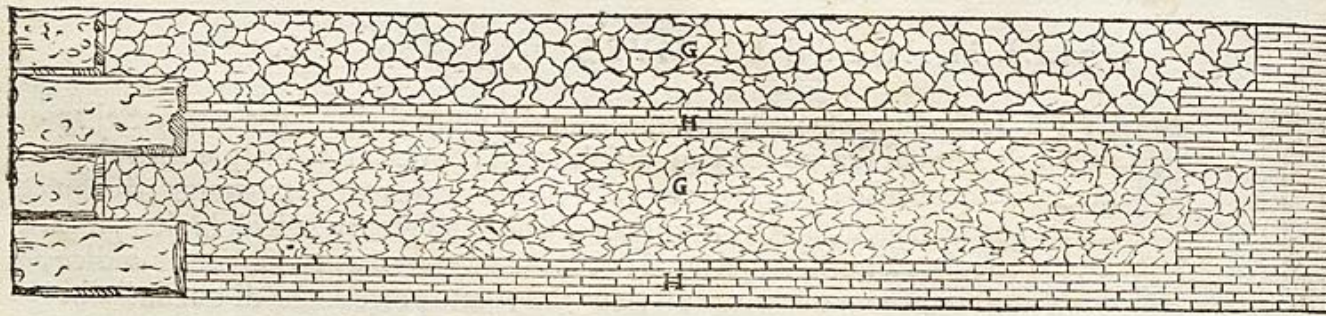
G, Cementi, o cuocoli di fiume. H, Corsi di quadrelli che legano tutto il muro.
