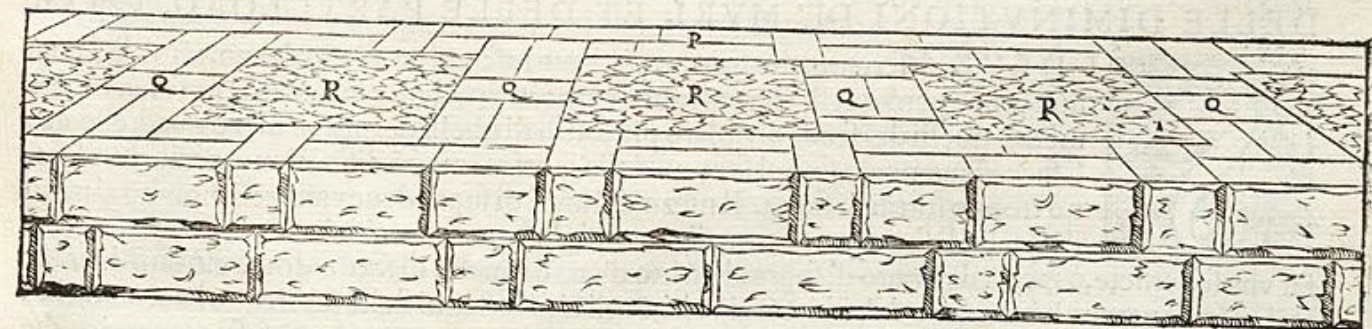
P, Muri di pietra esteriori. Q, Muri di pietra posti per trauerso. R, Casse piene di pietre, e di terra.
