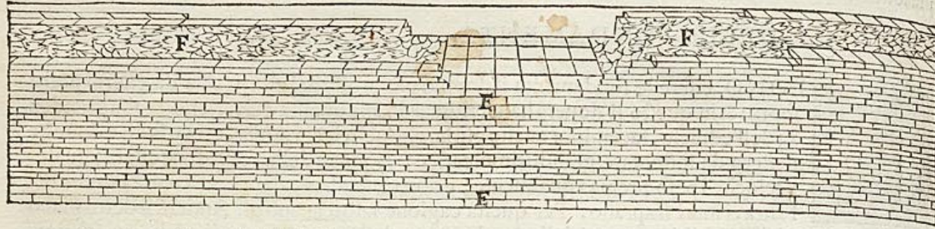
E, Corsi di quadrelli che legano tutto il muro. F, Parte di mezzo del muro fatta di cementi fra l'vn corso e l'altro & i quadrelli esteriori.
