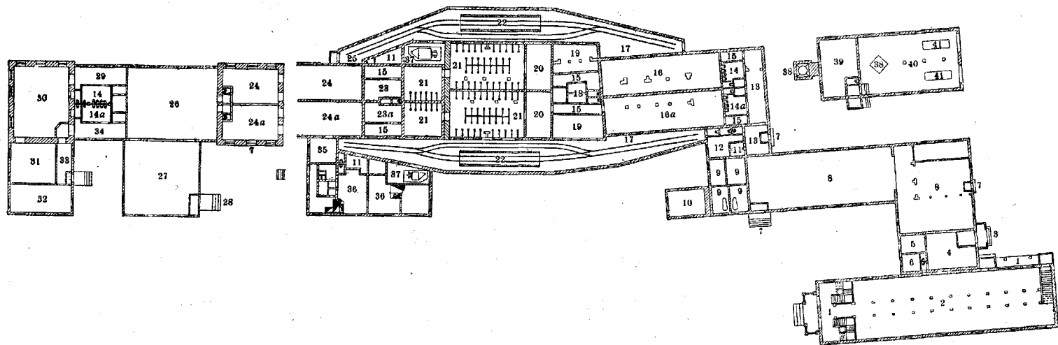
План Брянского санитарно-пропускного пункта:
