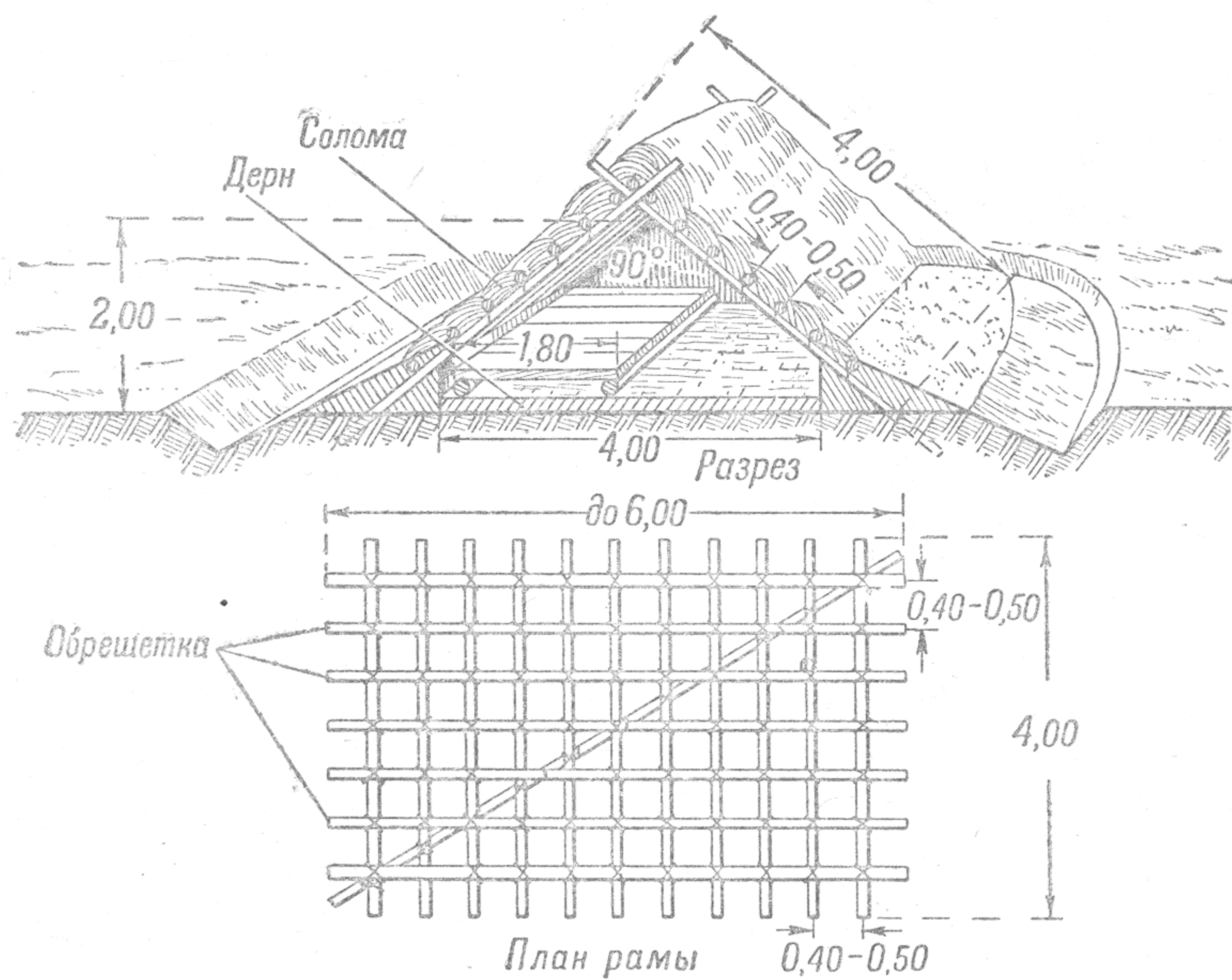
Рис. 10. Двускатный шалаш.
