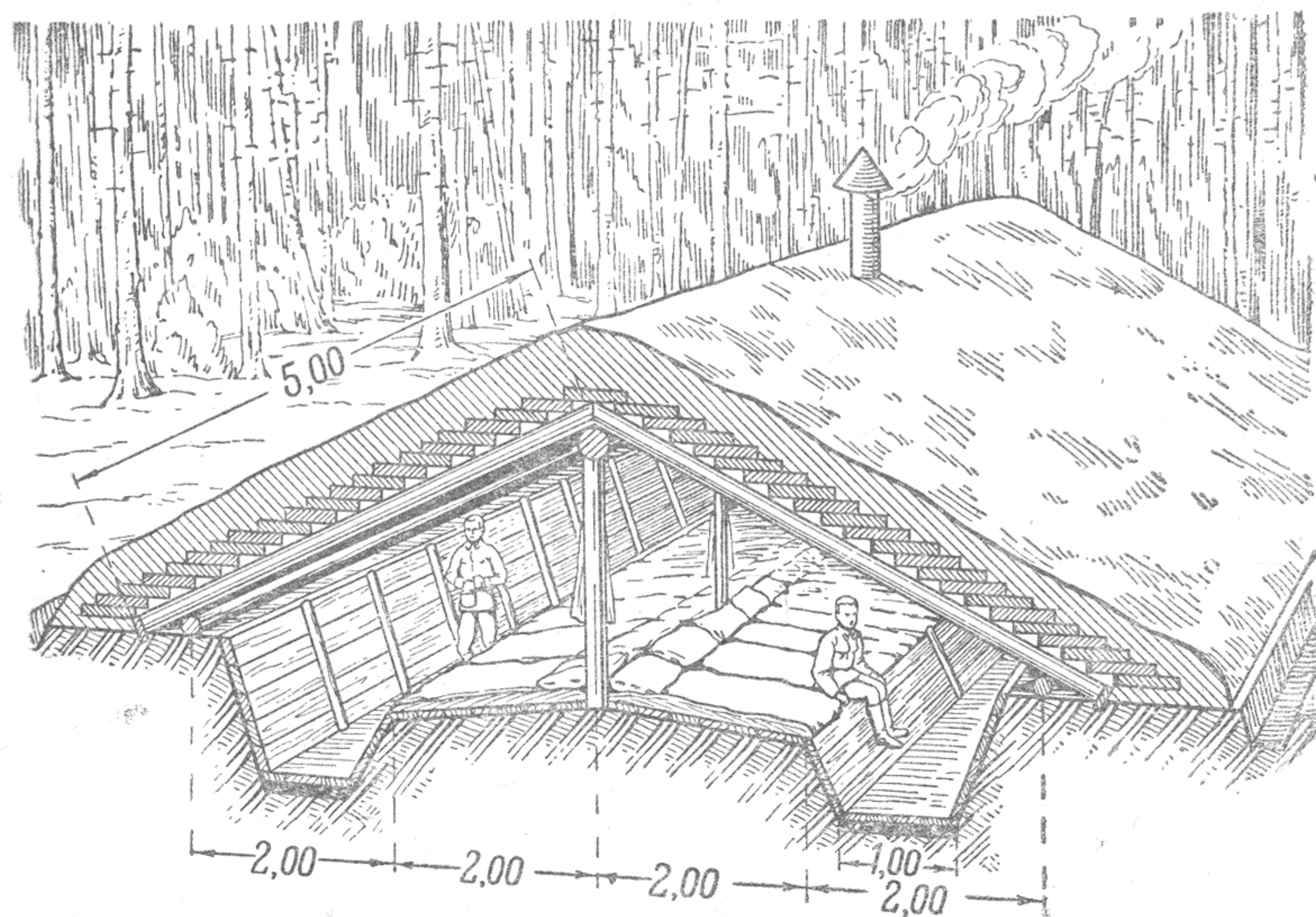
Рис. 13. Двускатная землянка.
