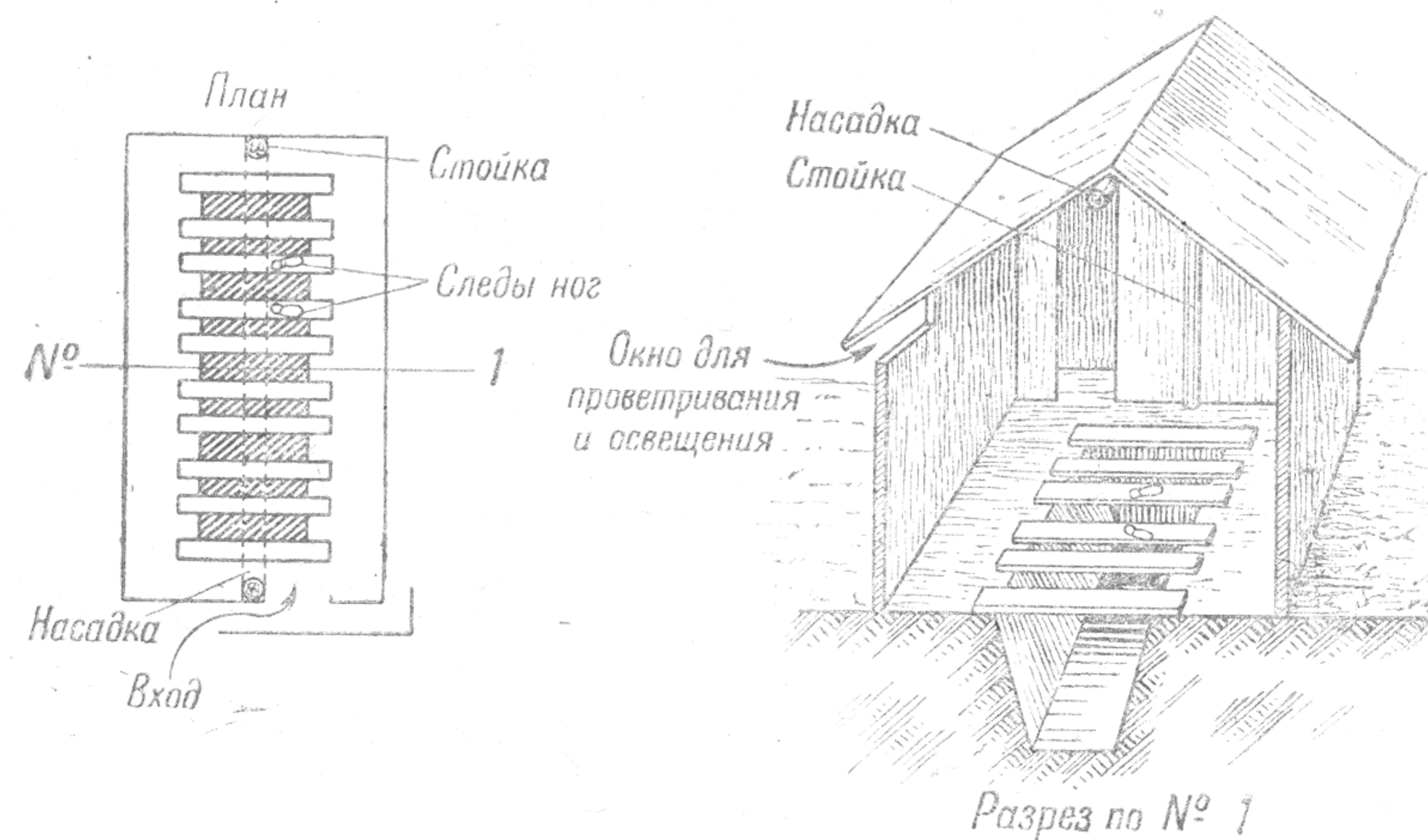
Рис. 29. Отхожее место.
