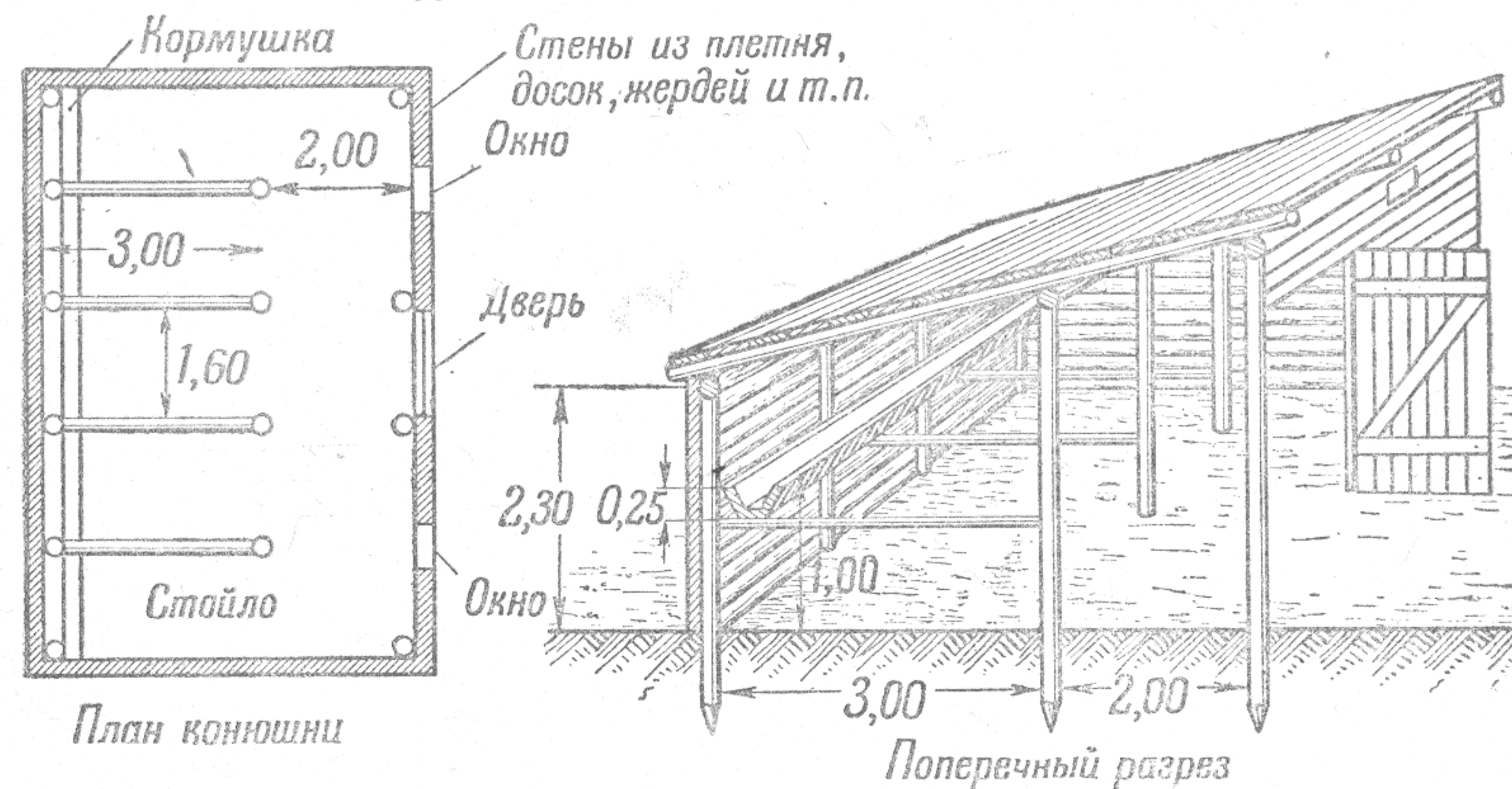
Рис. 18. Полевая конюшня.
