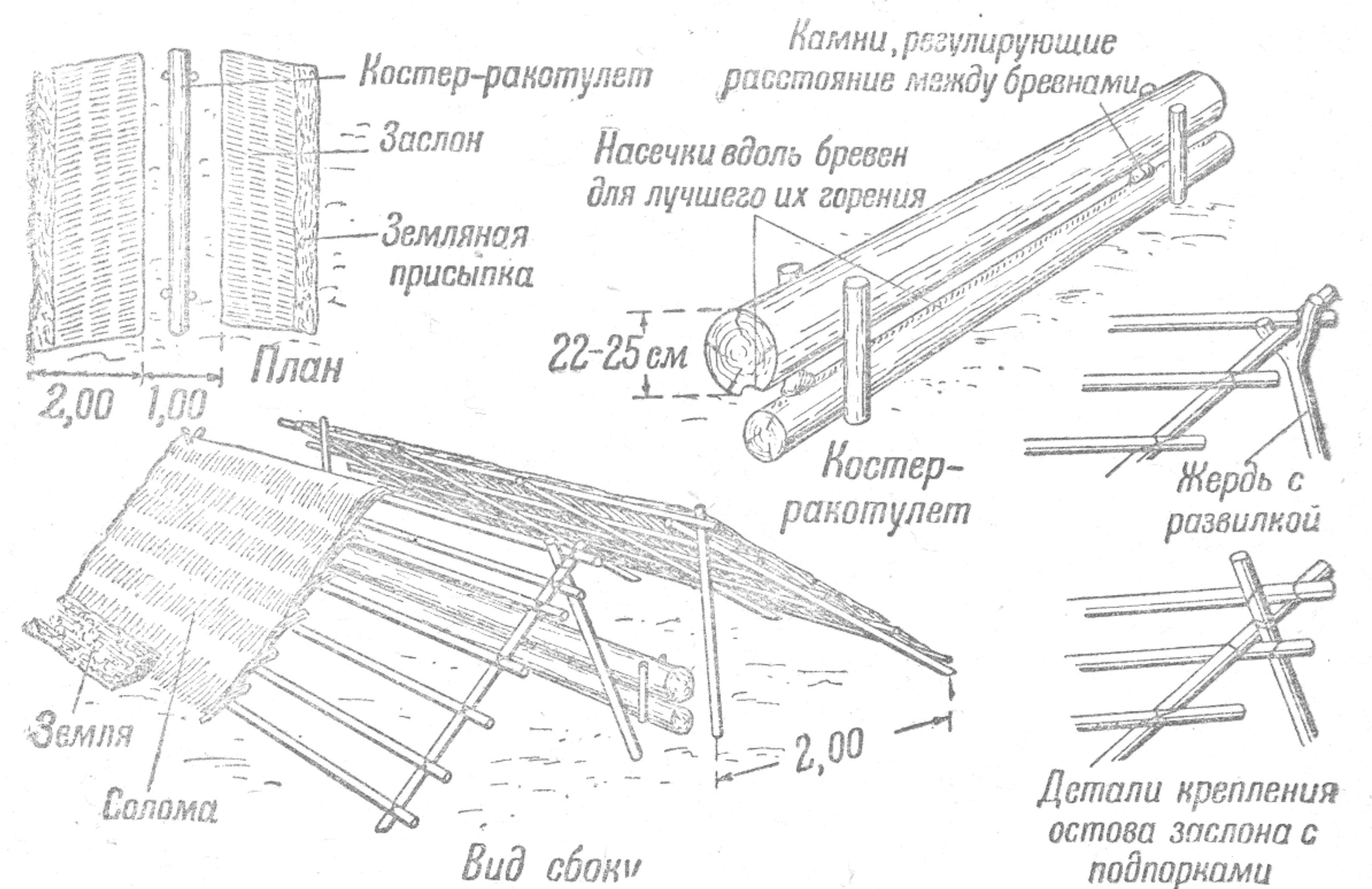
Рис. 8. Жердевой заслон.
