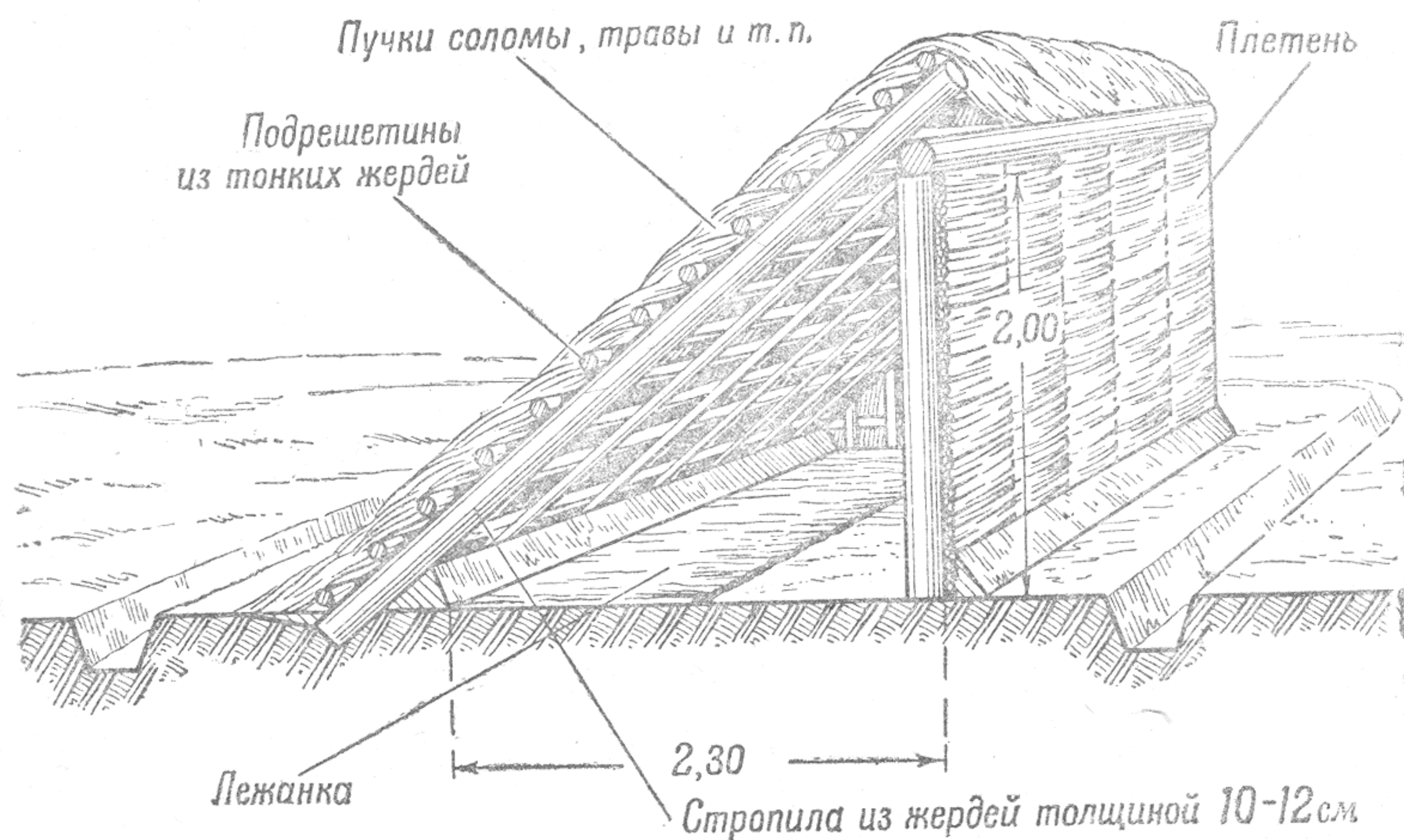
Рис. 9. Односкатный шалаш.
