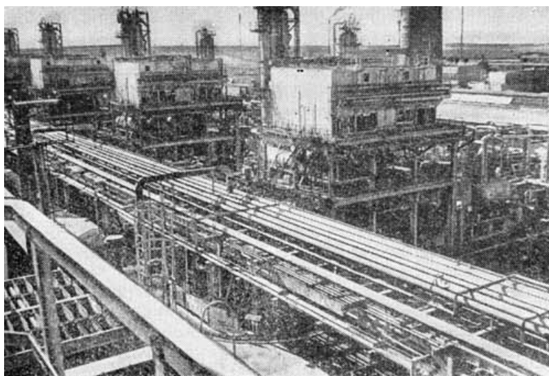
На Оренбургском газоперерабатывающем заводе
