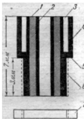
Рис. 84. Схема соединительной розетки к аппаратам
