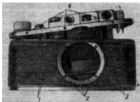
Рис. 78. Снятие кожуха камеры
