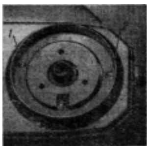
Рис. 116. Винты крепления шкалы скоростей
