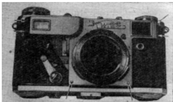
Рис. 143. Отделение обклейки при снятии щитка
