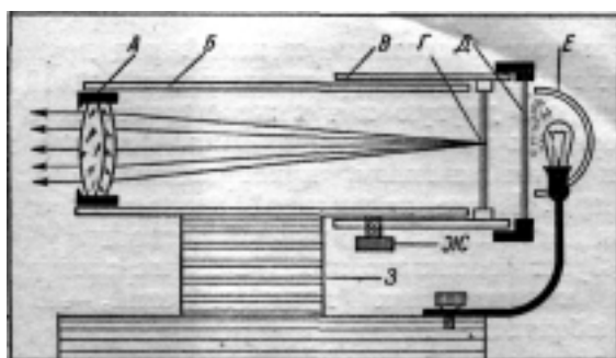
Рис. 7. Схема коллиматора
