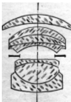
Рис. 5. Объектив «Юпитер-3» и его схема
