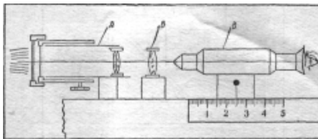
Рис. 9. Схема устройства для определения рабочего отрезка линз
