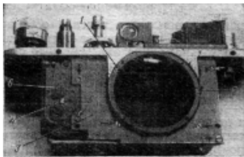
Рис. 106. Расположение рычагов автоспуска и винтов панели объектива
