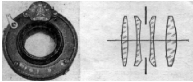
Рис. 3. Объектив «Ортагоз» и его схема
