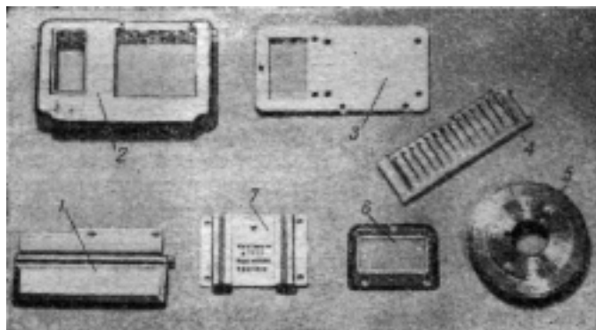
Рис. 152. Детали, подлежащие удалению при разборке экспонометра:
