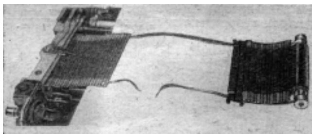
Рис. 133. Пружинный валик и шторка затвора
