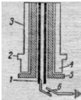
Рис. 50. Схема синхроконтактного гнезда
