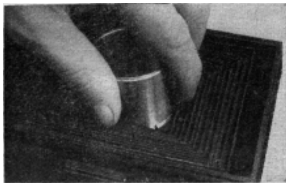
Рис. 13. Отвинчивание зажимного кольца трубчатым ключом
