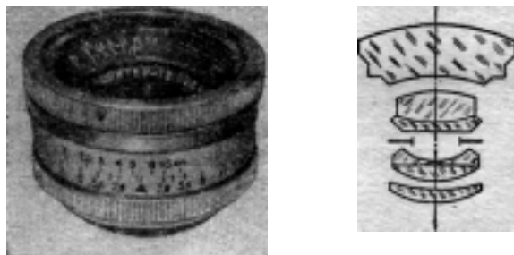
Рис. 6. Объектив «Юпитер-12» и его схема
