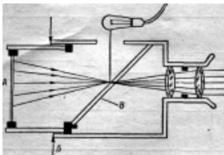
Рис. 8. Схема автоколлиматора
