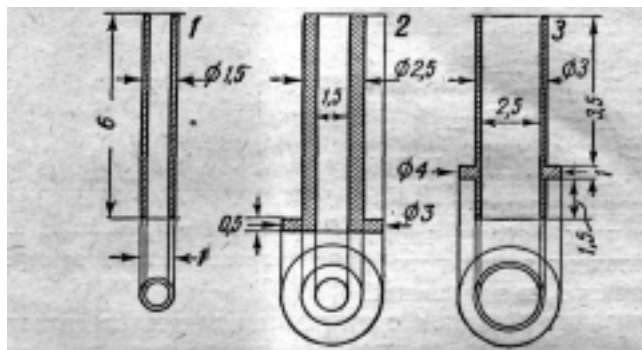
Рис. 51. Размеры трубок синхроконтального гнезда
