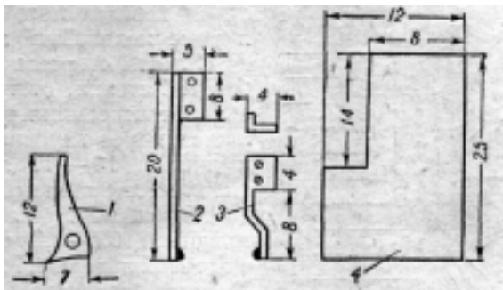
Рис. 140. Размеры деталей синхроустройства аппарата «Киев» (в мм)
