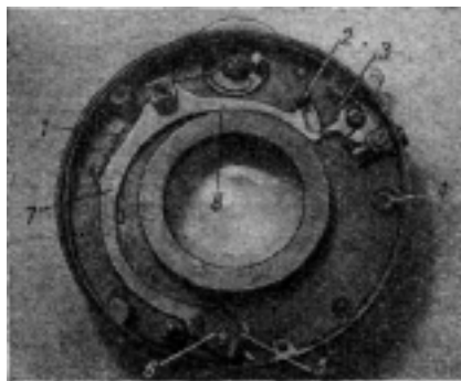
Рис. 28. Механизм затвора
