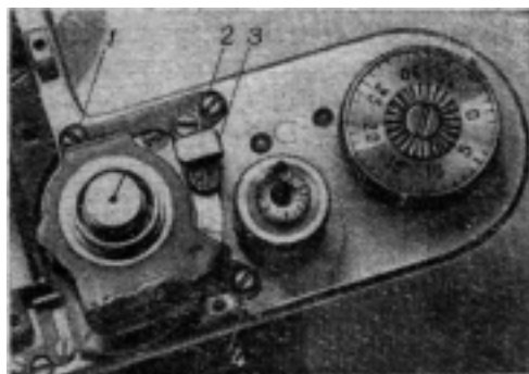
Рис. 165. Установка каретки синхроконт- тактов
