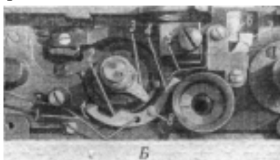
Рис. 99. Синхроустройство аппарата «ФЭД-2»
