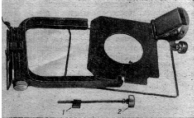
Рис. 16. Отделение доски объектива от стойки
