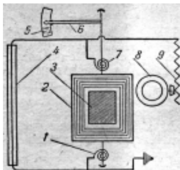
Рис. 147. Схема устройства экспониметра
