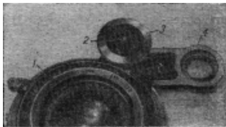
Рис. 42. Разборка компенсатора
