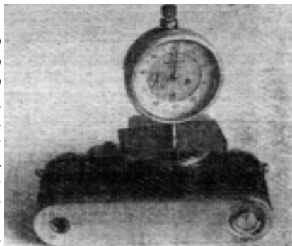
Рис. 176. Измерение рабочего отрезка камеры
