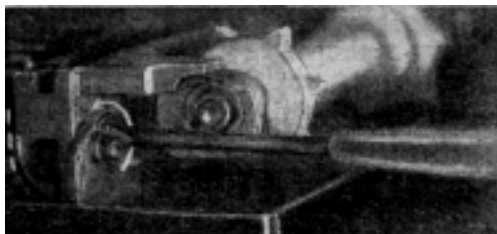
Рис. 137. Натяжение пружины валика
