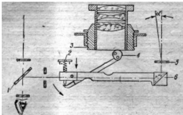
Рис. 87. Схема дальномера:
