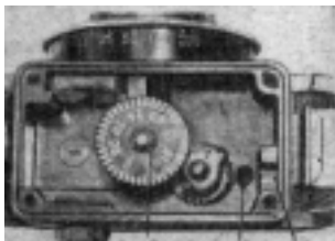
Рис. 66. Счетчик кадров аппарата «Смена»
