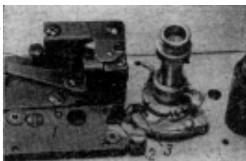
Рис. 109. Расположение запорной пластинки анкерного механизма
