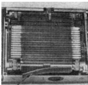
Рис. 127. Отклеилась кожа натяжного барабана
