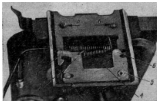
Рис. 17. Устройство фиксатора положения бесконечности
