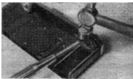
Рис. 121. Исправление замка крышки
