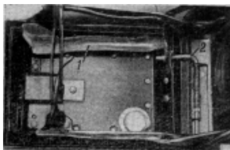
Рис. 37. Рычаги спуска затвора
