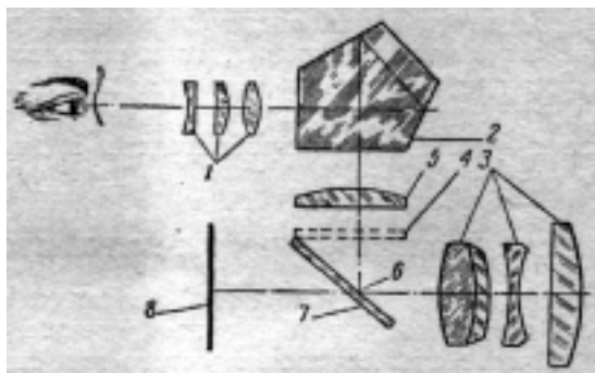
Рис. 167. Схема зеркально-телескопического устройства, работающего совместно с объективом
