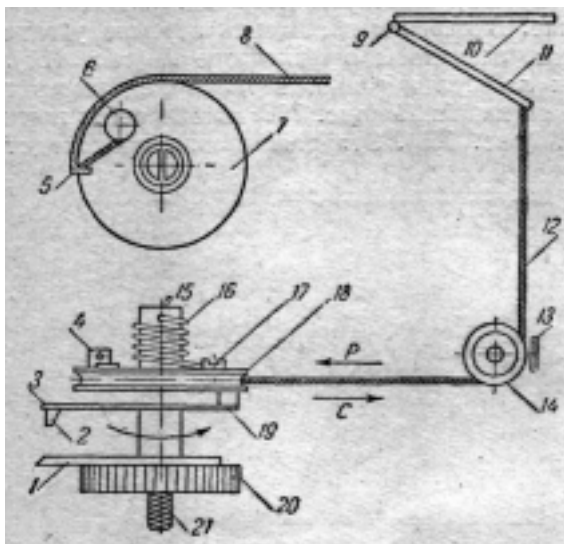
Рис. 168. Схема устройства лебедки для перемещения зеркала
