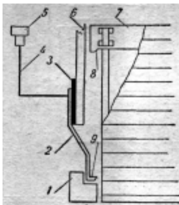
Рис. 141. Схема одноконтakтного замыкания синхроустройства:
