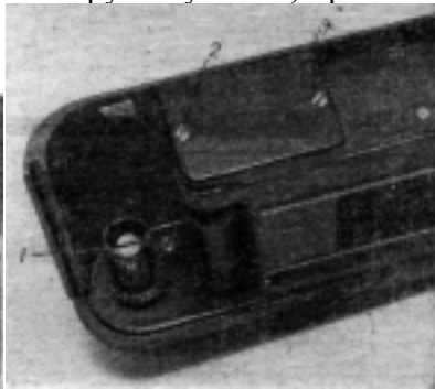
Рис. 97. Винт крепления фрикционного барабана
