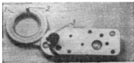
Рис. 110. Анкерный механизм (вид снизу)
