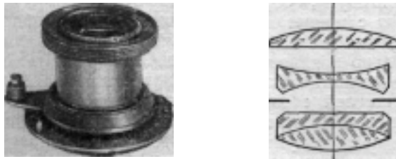
Рис. 4. Объектив «Индустар» и его схема
