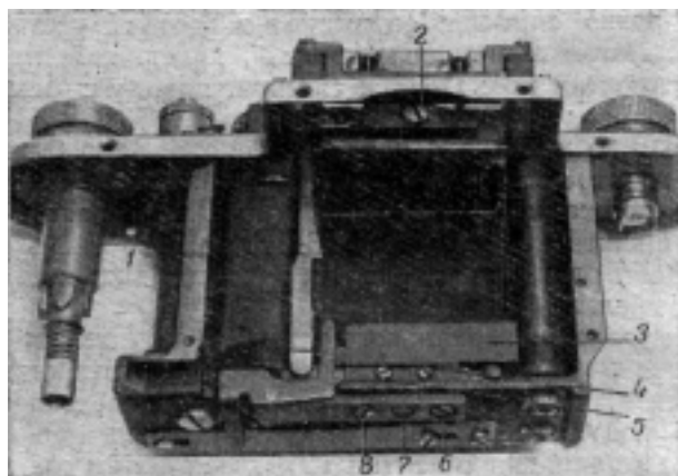
Рис. 157. Система установки зеркала
