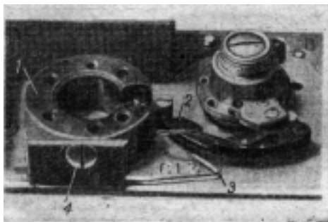
Рис. 85. Крепление синхроконтакта
