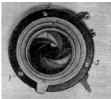
Рис. 47. Винты крепления механизма затвора
