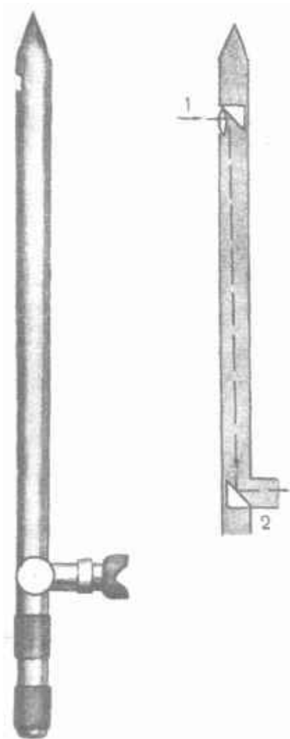
Маленький призмный перископ очень удобен для «потайного» наблюдения за врагом: 1—объектив; 2—окуляр.
