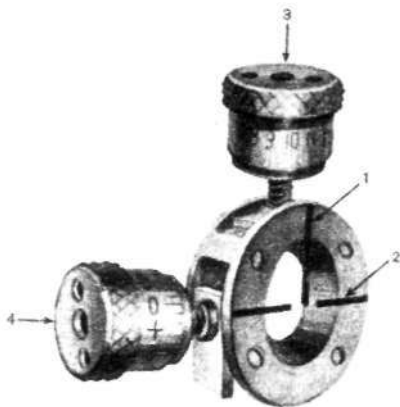
Корпус оптического прицела: 1 — прицельный пеньк; 2 — выравнивающие нити; 3 — дистанционный барабанчик; 4 — барабанчик для боковых поправок.
