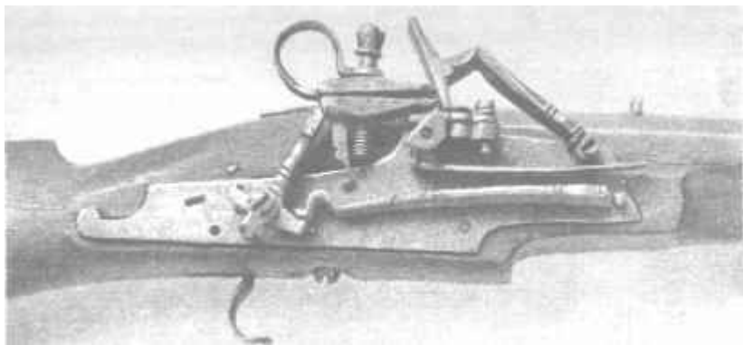
Нидерландский кремневый замок. Мирные жители называли его «курокрад».
