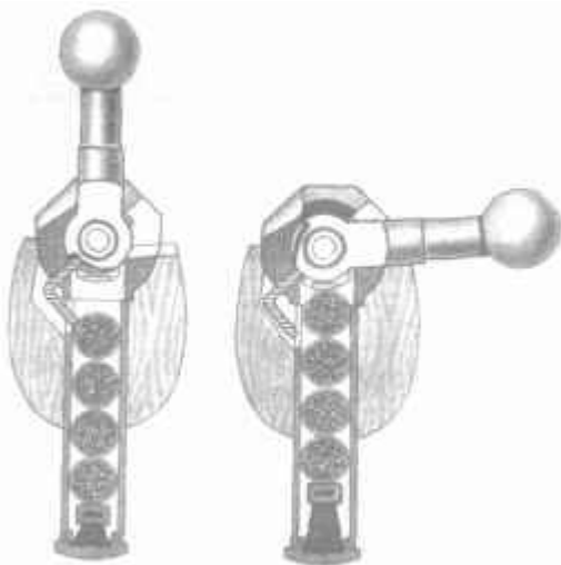
Магазин с отсеккой-отражателем Мосина.
