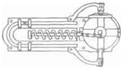
Колесный замок Леонардо да Винчи.
