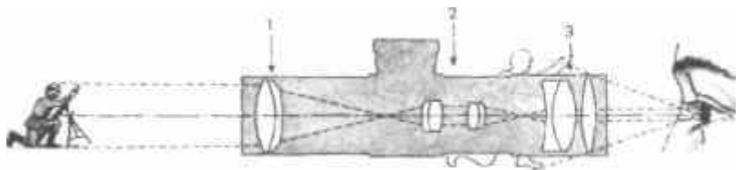
Ход лучей в оптическом прицеле: 1 — объектив. 2 — оборачивающая система линз, 3 -- окуляр
