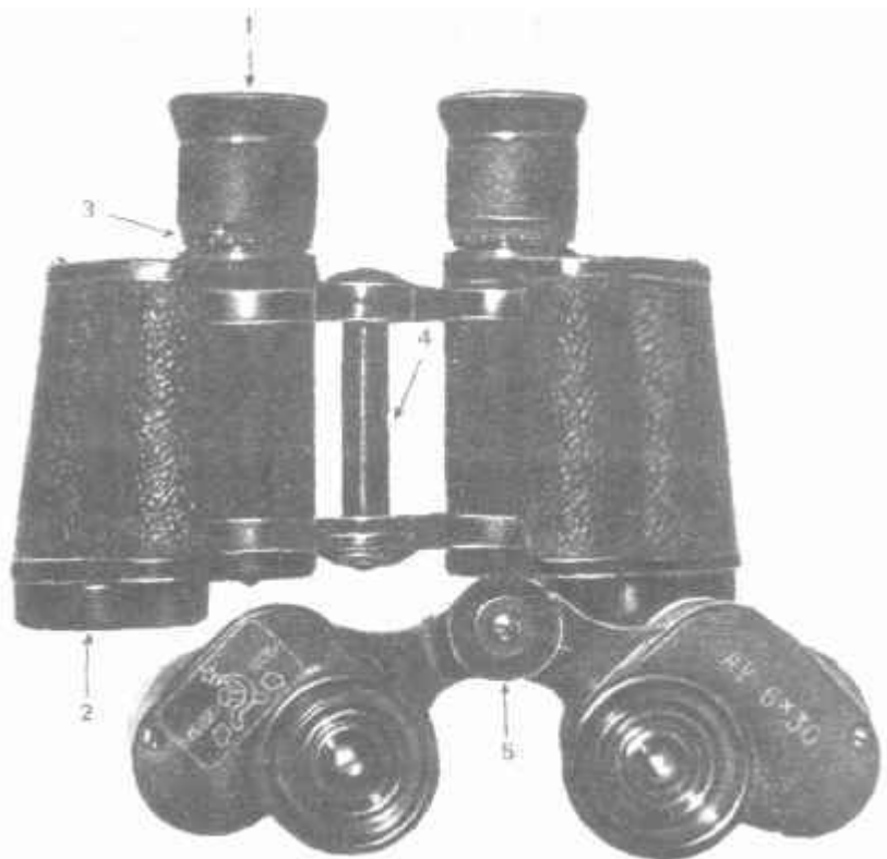
Призматический бинокль: 1--окуляр, 2 — объектив; 3 — шкала для установки на резкость изображения; 4 — шарнирная ось; 5 — шкала для установки по глазам.
