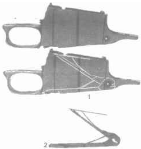
1 — магазинная коробка; 2 — внутри нее находится подающий механизм.
