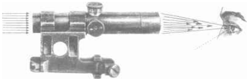
Входной и выходной зрачок.
