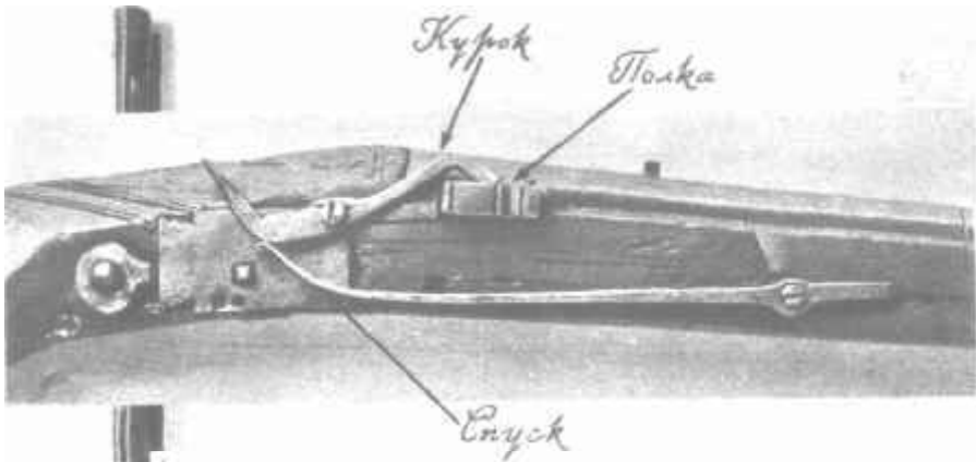
На таких фитильных ружьях стреляли в XVI веке. На верхнем снимке видно, как устроен фитильный замок.
