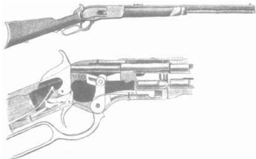
Винтовка с подствольным магазином.
