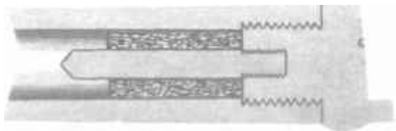
Штуцер со стержнем в пороховой камере
