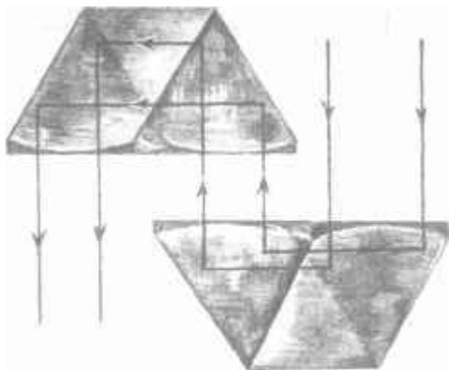
Так луч поворачивается в призмах.
