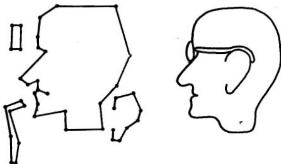
Рис. 20. Аппроксимации: линейная (слева) и кубическими сплайнами (справа)
