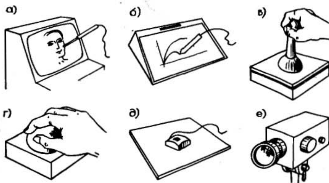
Рис. 2. Устройства ввода графической информации: а — световое перо; б — планшет; в — координатный рычаг; г — шар; д — мышь; е — сканирующая система
