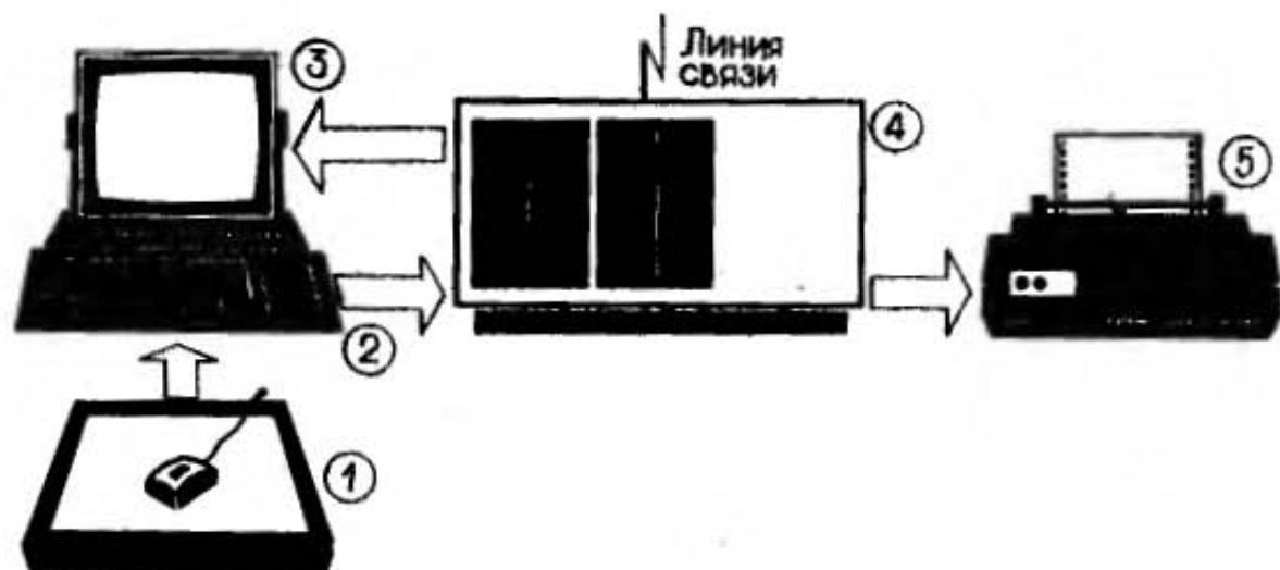
Рис. 1. Персональная графическая система: 1 — устройство ввода; 2 — клавиатура; 3 — дисплей (здесь же располагается и процессор); 4 — устройство внешней памяти (накопитель на магнитных сменных дисках); 5 — устройство регистрации информации
