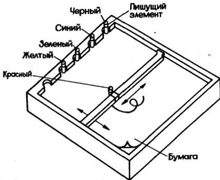
Рис. 10. Планшетный многоцветный графопостроитель
