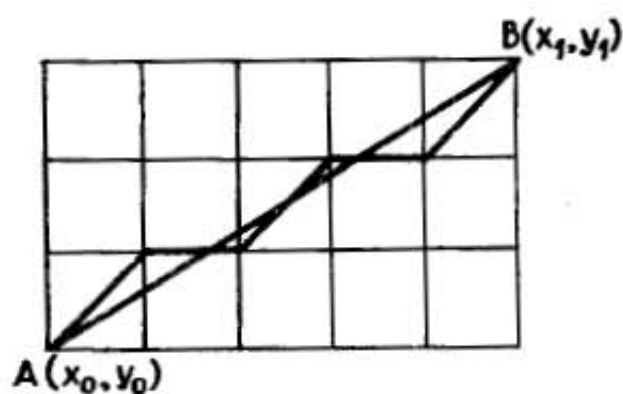
Рис. 15. Аппроксимация прямой линии в векторной графике
