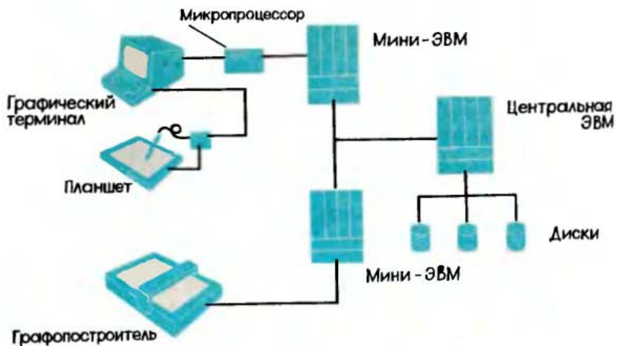
Рис. 51. Графическая система с двумя процессорами
