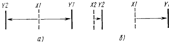
Рис. 2.13. Конкуренция при слиянии: X1 расщепляется (а), X1 не расщепляется благодаря конкуренции со стороны X2 (б)
