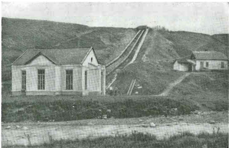
Колхозная гидроэлектростанция. Чуйская долина
