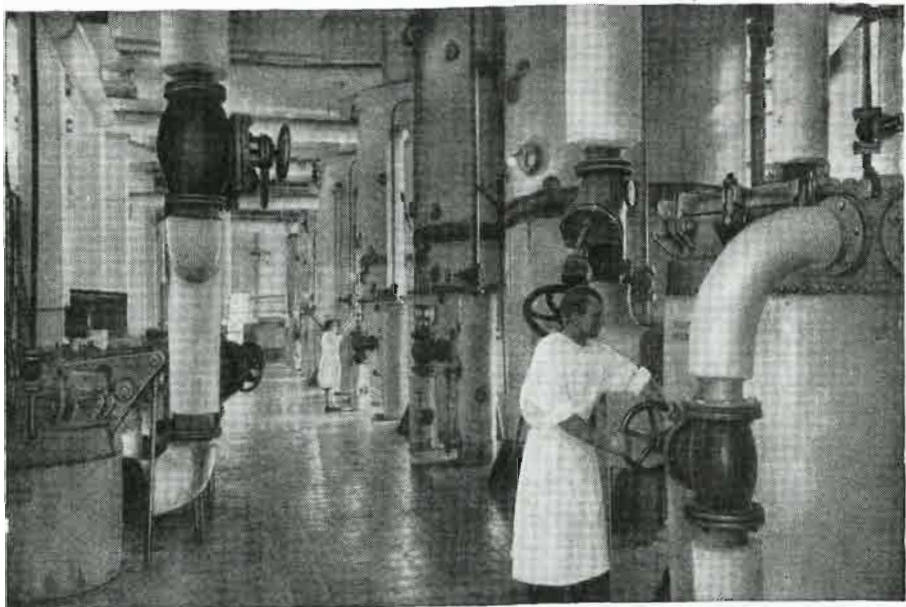
Выпарная станция Новотроицкого сахарного завода. Чуйская долина
