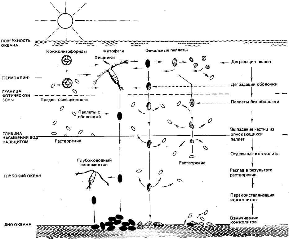
Рис. 14-17. Модель взаимосвязей между продукцией, переносом, растворением и осаждением кокколитоидов в открытом глубоком океане. Шкалы непропорциональны. Скорость осаждения кокколитоидов: в виде пеллет—160 м/сут, в виде дискретных кокколитоидов—0,15 м/сут [482].
