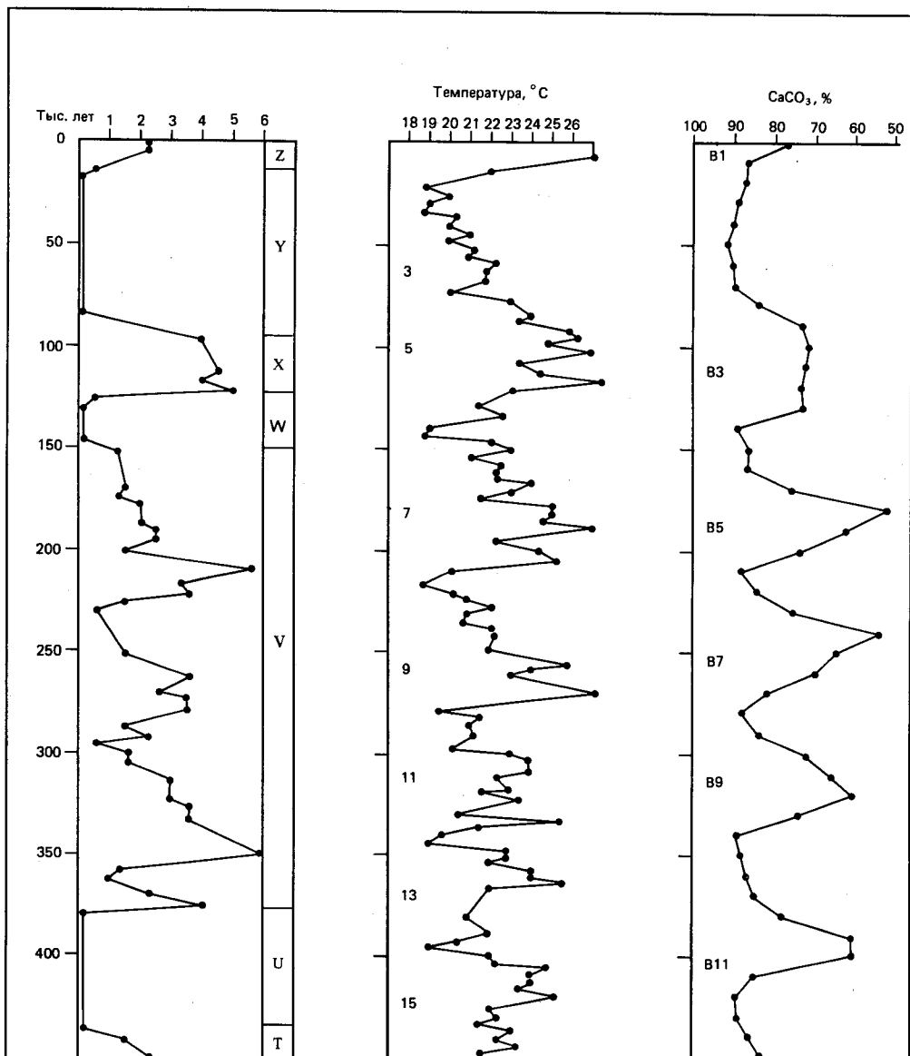
Рис. 17-14. Сравнение двух кривых относительных палеотемператур с кривой содержания CaCO 3 в колонке из экваториальной части Тихого океана. Кривая слева отражает колебания содержания тропического вида планктонных фораминифер Globorotalia menardii ([440], с. 507; публикуется с разрешения Геологического общества США).
