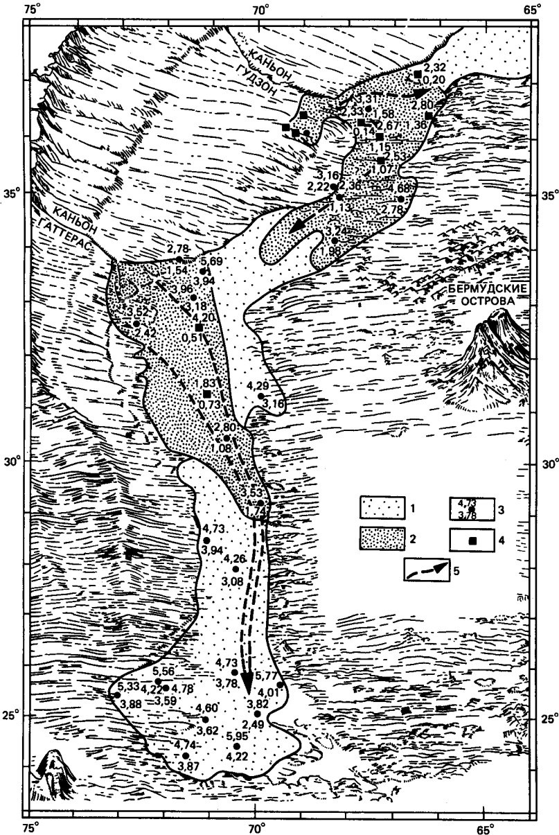
Рис. 13-12. Распространение песка и силта на абиссальной равнине Гаттерас у восточного побережья США, отложенных турбидными потоками, вытекающими из подводных каньонов. 1—силт; 2—песок; 3—расположение колонок; цифрами обозначены медианный (верхняя) и максимальный (нижняя) диаметры зерен (в единицах фи) в наиболее грубозернистом базальном слое турбидита в каждой колонке; 4—колонки с неградационными слоями; 5—предполагаемые главные трассы турбидных потоков [488].
