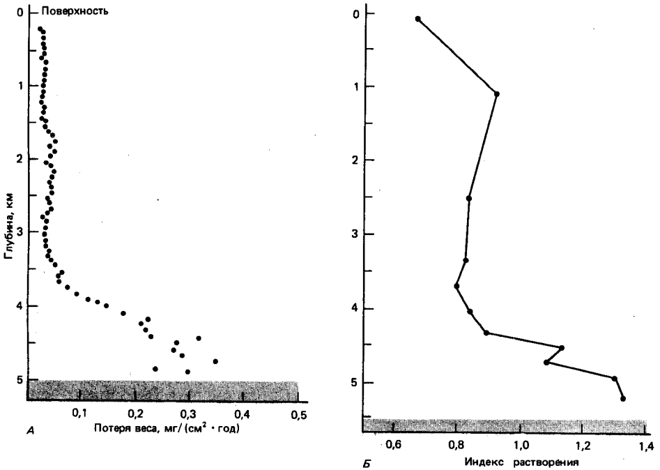
Рис. 14-7. Кривые растворения карбоната кальция в океанах. А — график скорости растворения кальцита на заякоренном буе в центральной части Тихого океана, демонстрирующий существование уровня быстрого увеличения скорости растворения вблизи 3700 м (по данным Петерсона [823]). Б — график степени сохранности («индекса растворения») фораминифер в Центральной Атлантике, показывающий резкий переход от комплексов фораминифер хорошей сохранности к комплексам плохой сохранности на глубине около 4500 м (фораминиферовый лизоклин) [71].
