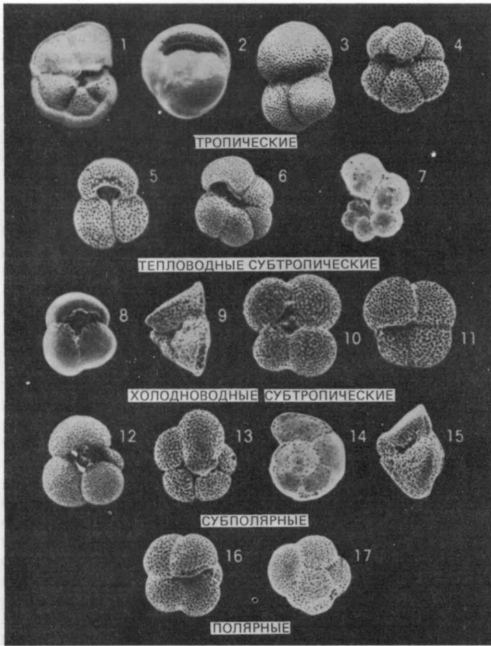
Рис. 16-1. Распространение современных видов планктонных фораминифер. Тропические виды: 1 - Globorotalia menardii , \times 54 ; 2 - Pulleniatina obliquiloculata , \times 110 ; 3 - Globigerinoides sacculifer , \times 148 ; 4 - Neogloboquadrina dutertrei (форма с зубом), \times 81 . Тепловодные субтропические виды: 5 - Globigerinoides ruber , \times 102 ; 6 - Neogloboquadrina dutertrei , \times 72 ; 7 - Hastigerina pelagica , \times 60 . Холодноводные субтропические виды: 8 - Globorotalia inflata , \times 60 ; 9 - Globorotalia truncatulinoides , \times 86 ; 10 - Globigerina falconensis , \times 120 ; 11 - Neogloboquadrina pachyderma (правозавитая), \times 138 . Субполярные виды: 12 - Globigerina bulloides , \times 91 ; 13 - Globigerina quinqueloba , \times 180 ; 14 - Globorotalia truncatulinoides , \times 60 ; 15 - Globorotalia truncatulinoides , \times 89 . Полярные виды: 16 - Neogloboquadrina pachyderma (левозавитая), \times 141 ; 17 - Neogloboquadrina pachyderma (левозавитая), \times 152 .
