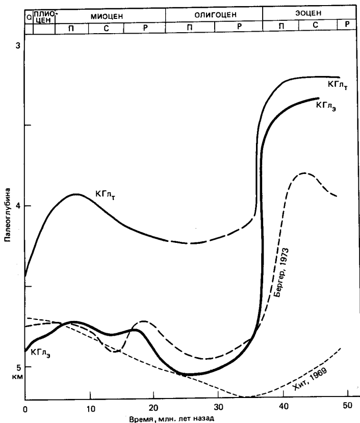
Рис. 19-14. Изменения компенсационной глубины карбоната (КГл) в кайнозое в экваториальной зоне, между 3° с. ш. и 3° ю. ш. (КГл 3 ), и в Тихом океане, севернее 4° с. ш. и южнее 4° ю. ш. (КГл т ) [1075]. Для сравнения приведены кривые колебания КГл, полученные Хитом [441] и Бергером [68]. На всех кривых видно резкое опускание КГл у границы эоцено-олигоцен [1075].
