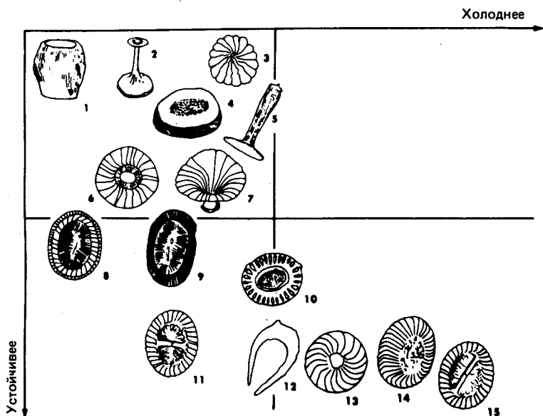
Рис. 16-15. Известковые нанофоссилии как показатель палеотемператур и условий сохранности. Можно видеть, что флора худшей сохранности явно имеет холодноводный облик. Кокколлиты: 1— Scyphosphaera sp.; 2— Discosphaera tubifera ; 3— Cyclocolithina fragilis ; 4— Pontosphaera sp.; 5— Rhabdosphaera clavigerina ; 6— Cyclolithella annual ; 7— Umbellosphaera sp.; 8— Syracosphaera pulchra ; 9— Helicopontosphaera kamptneri ; 10— Emiliana huxleyi ; 11— Gephyrocapsa oceanica ; 12— Ceratolithus cristatus ; 13— Cyclococcolithina leptopora ; 14— Coccolithus pelagicus ; 15— Gephyrocapsa caribbeanica ([78], с. 564).
