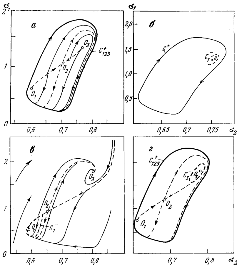
Рис. 13. Фазовые портреты модели (2.36) реакции (2.32) при \gamma = 2 , \xi = 0,1 и \alpha = 1 , \varepsilon = 0,02 (a — б), \alpha = 5 , \varepsilon = 0,08 (в)
