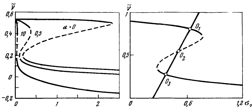
Рис. 6. Семейство квазистационарных выходных характеристик реакции (2.12), построенных по уравнению (2.19) при \nu_{1m} = 0,55 , \beta_1 = 0,165 , \xi = 0,1 , \gamma = 2 и различных значениях \alpha (цифры на кривых)
