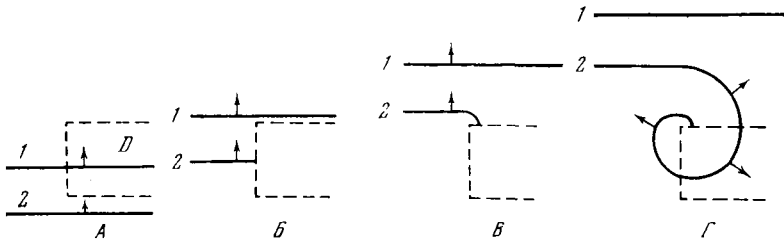
Рис. 61. Возникновение ревербератора (спиральной волны в среде без отверстий и препятствий)
