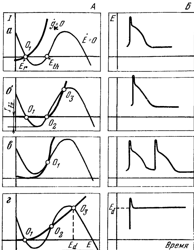
Рис. 45. Фазовые портреты мембран (А) и их электрическая активность (Б) а, б — нормальные мембраны без спонтанной активности; в — спонтанно активная мембрана; з — мембрана с устойчивой деполяризацией. E_r — потенциал покоя, E_{th} — пороговый потенциал, E_d — потенциал устойчивой деполяризации, I_{th} — пороговый ток (ток реобазы)
