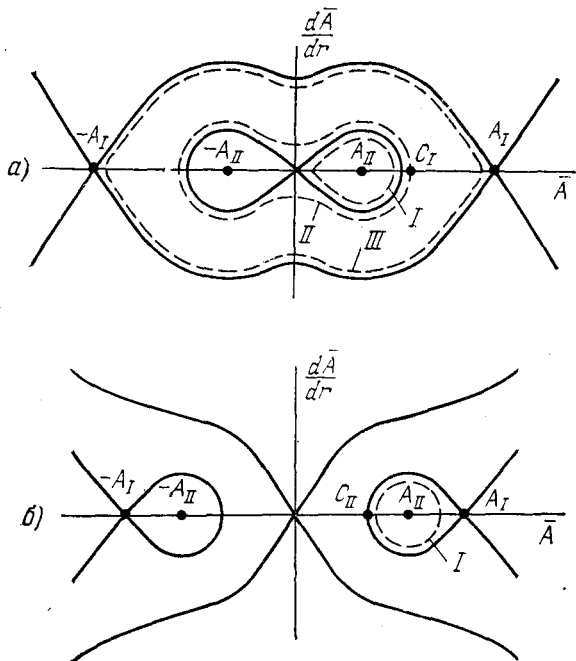
Рис. 10.8. Фазовая плоскость уравнения (10.34).
