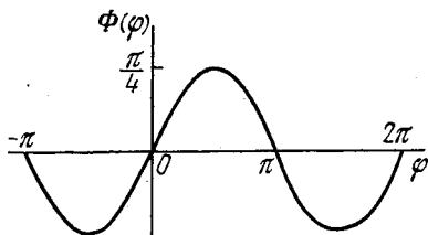
Рис. 12.6. График функции \Phi(\varphi) .
