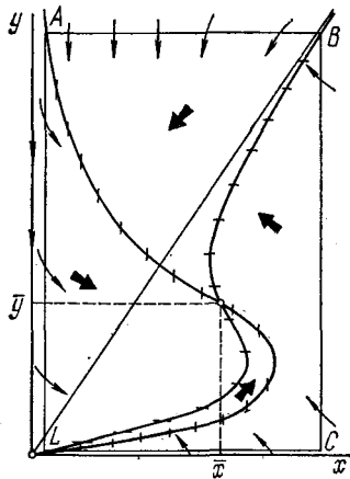
Рис. 8.9. Главные изоклины системы (8.22).
