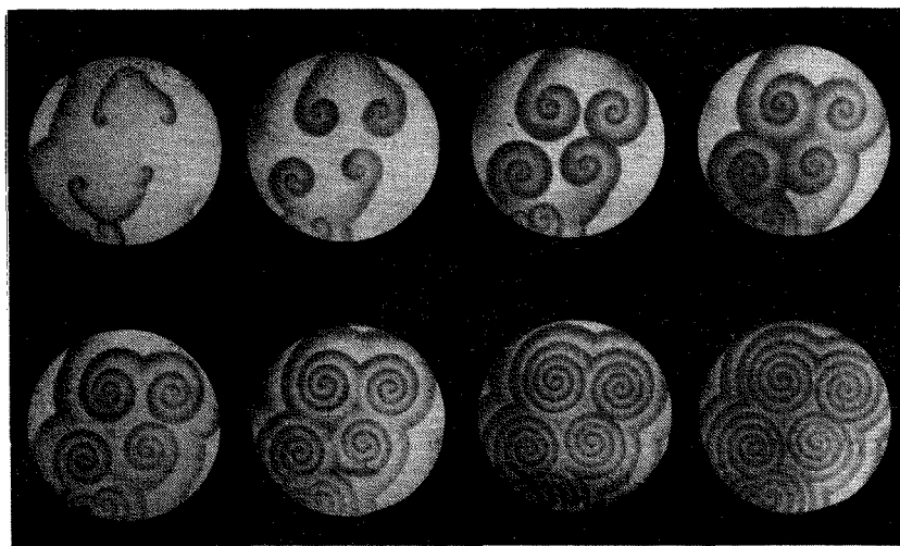
Рис. 10.2. Ревербераторы в плоском реакторе.
