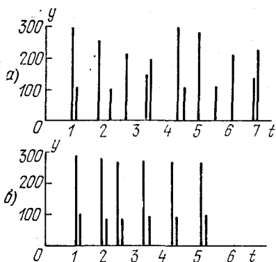
Рис. 13.7. Колебания связанных релаксаторов (13.52) (расчет на ЭВМ). Вертикальные линии соответствуют фронтам импульсов. а) Режим бистабильный. б) Синхронный режим; первые два периода — время установления синхронизма.
