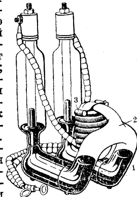
Рис. 6. Самозажигающаяся ртутно-кварцевая горелка Jaeniske: 1—ртуть в полном сосуде; 2—световая трубка; 3—спираль накала.
