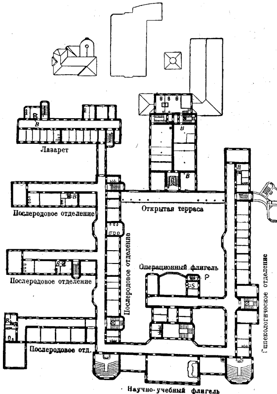
Рис. 3. План III этажа: В—подъемные машины; S—паровые стерилизаторы; P—аппараты для физиологического раствора.
