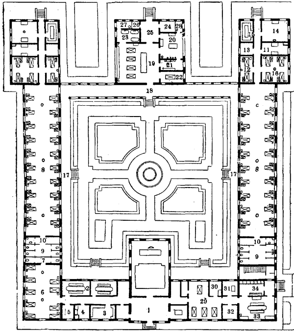
Рис. 4. План родильного дома St.-Antoine в Париже: 1—вестибюль; 2—7—отделение беременных; 8—16—послеродовое отделение; 17—открытая галерея; 18—закрытая веранда; 19—28—родильное отделение с приемной; 29—34—консультация; 35—39—изоляционное отделение (отдельное здание).
