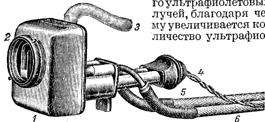
Рис. 5. Лампа Крамайера: 1—футляр для ртутно-кварцевой горелки; 2—кварцевое окно; 3—ручка для наклона лампы при зажигании; 4—электрические провода; 5 и 6—резиновые трубки—приводящая и отводящая воду для охлаждения.
