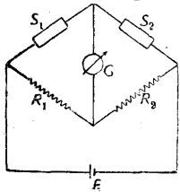
Рис. 5. Схема болометра: S_1 —тонкая платиновая полоска, на которую падает свет; S_2 —такая же пластинка, защищенная от света; R_1 и R_2 —известные сопротивления; G —гальванометр; E —электрическая батарея.
