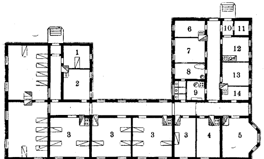
Рис. 17. План 10—20-кратного сельского родильного приюта: 1—изоляция; 2—акушерка; 3—палаты; 4—родильная; 5—операционная; 6—бельевая; 7—смотровая; 8—ванная; 9—уборная; 10—прихожая; 11—кладовая; 12—кухня; 13—сиделки; 14—стерилизационная.
