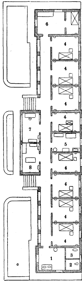
Рис. 13. План изоляционного отделения родильного дома St.-Antoine в Париже: 1—умывальная; 2 и 3—уборная; 4—палаты; 5—служебная; 6—комната для акушерок; 7—комната для сиделок; 8—операционная.
