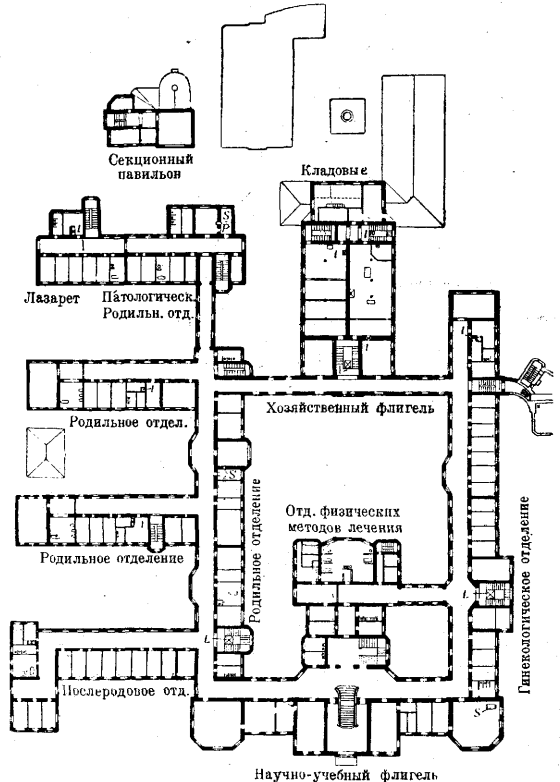
Рис. 2. План II этажа: L—лифты для больных; S—подъемные машины; S—паровые стерилизаторы; P—аппараты для физиологического раствора.
