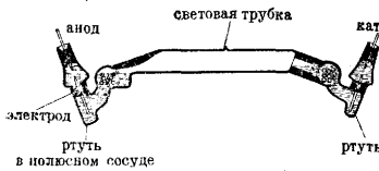
Рис. 1. Продольный разрез ртутно-кварцевой горелки.
