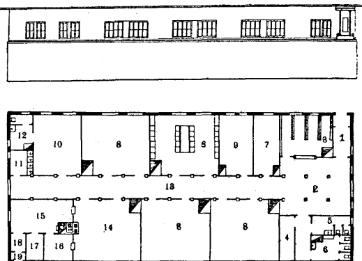
Рис. 1. Барак-ожидания: 1—вход для прибывших; 2—вестибюль; 3—гардеробная; 4—хозяйственная; 5—женская уборная; 6—мужская уборная; 7—персональная; 8—комната на 25 чел.; 9—комната первой мед. помощи; 10—детская комната; 11—умывальня; 12—детская уборная; 13—коридор; 14—закусочная; 15—комната подачи пищи; 16—мойка посуды; 17—кладовая; 18—сени; 19—вход и выход персонала буфета.
