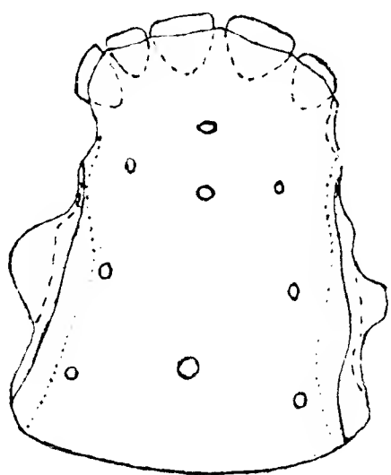
Фиг. 3. Сплошная линія — «per[r'ε]» 2 ; пунктиръ — «e».
