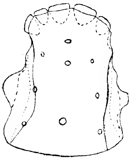
Фиг. 1. Сплошная линия — «і»; пунктиръ — «і».
