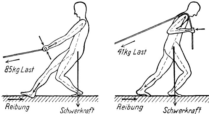
Abb. 64. Zerlegung der Bewegungs- und Gleichgewichtskräfte bei der Zieharbeit.
