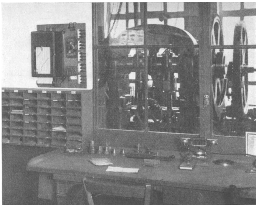
Abb. 50. Die Arbeitsschauuhr im Betriebe zur Überwachung der Arbeitsleistung von Stanzen. Die Uhr ist im Meisterraum angeordnet, so daß sich der Meister jederzeit von der Ausnutzung der Maschinen überzeugen kann.
