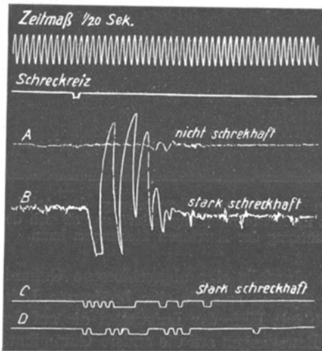
Abb. 52. Registrierung von Zitterbewegungen mittels des pneumatischen Registrierverfahrens.
