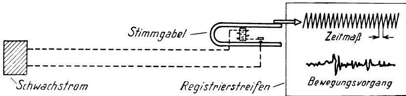
Abb. 41. Schaltbild für die Zeitmessung mittels Registrierapparates und Stimmgabel.
