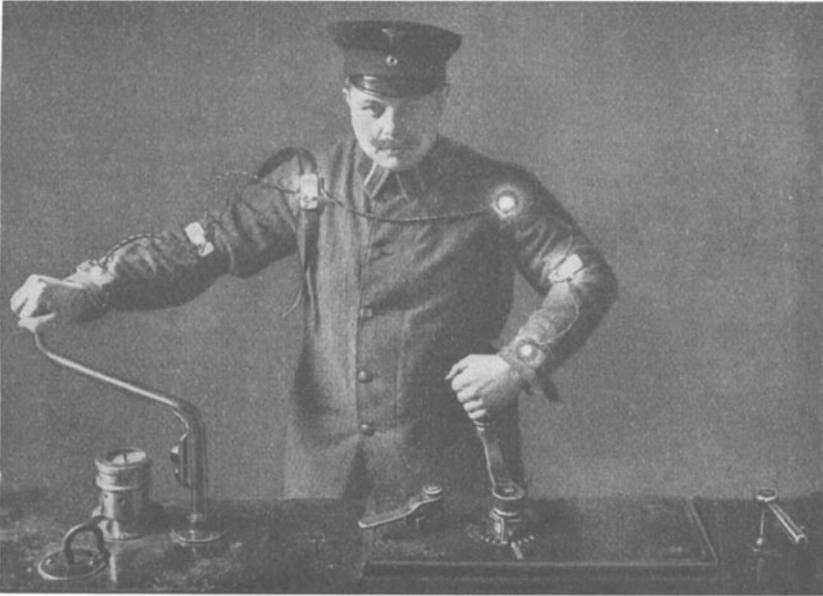
Abb. 55. Ausrüstung einer Versuchsperson für die gewöhnliche Punktbewegungsphotographie. Die Anordnung wurde bei der Untersuchung von Straßenbahnnotbremsenbedienungen angewandt.
