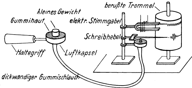
Abb. 51. Versuchsanordnung für die Untersuchung von Bewegungsruhe und Schreckhaftigkeit mittels pneumatischer Registrierung.
