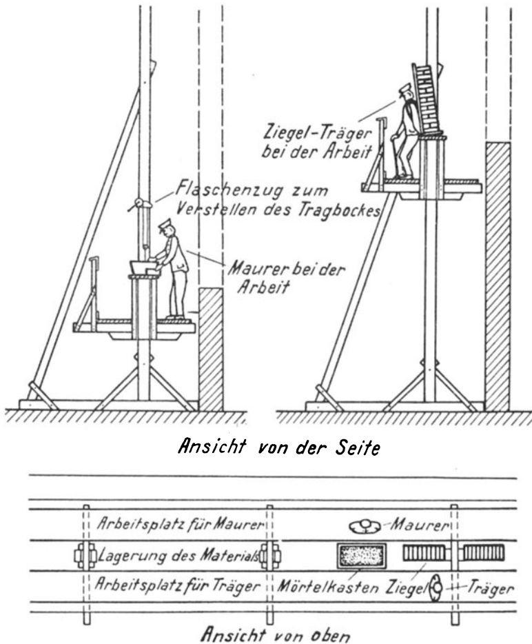
Abb. 66. Ein neuzeitliches Baugerüst (Gilbreth-Gerüst), welches das Bücken des Maurers und Trägers vermeidet, und hierdurch die ungünstigen dynamischen und statischen Beanspruchungen beseitigt.
