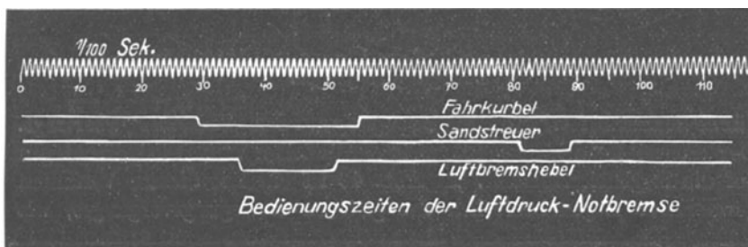
Abb. 44. Ergebnis einer Zeitmessung mittels Stimmgabel und Zeichenmagneten.
