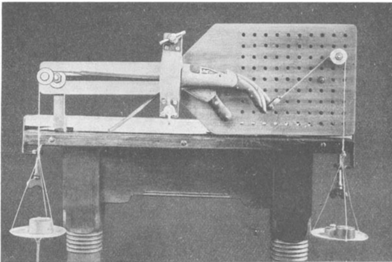
Abb. 69. Messung einer künstlichen Hand durch Auswägen.
