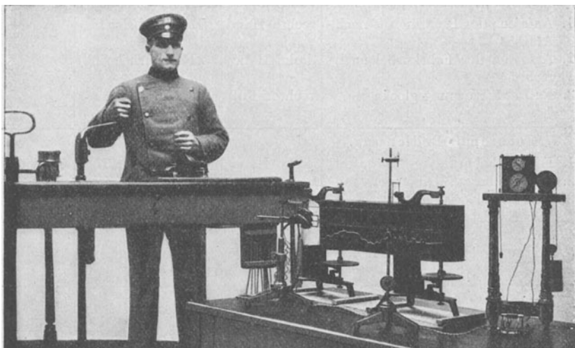
Abb. 73. Versuchsanordnung zur Messung von Bedienungszeiten für Straßenbahnnotbremsen. Die Zeit wurde mittels Doppelregistrierapparat gemessen (vgl. Abb. 42).
