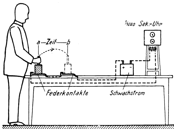
Abb. 34. Beispiel für eine Zeitmessung mittels \frac{1}{1000} -Sekunden-Uhr. Die Zeit für die Bewegung von a nach b wird bei obiger Schaltung in \frac{1}{1000} -Sekunden gemessen.
