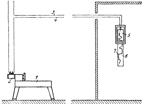
Abb. 39. Die Beurteilung der menschlichen Arbeitsleistung an Hand der Antriebsleistung des Elektromotors.
