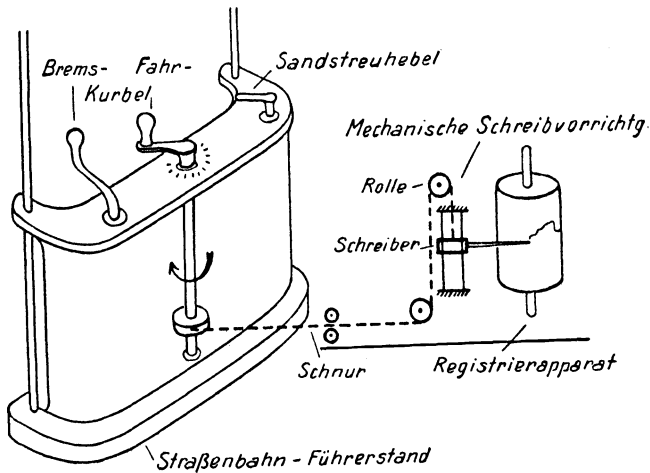
Abb. 45. Mechanische Schreibvorrichtung zur Aufzeichnung von Bewegungsvorgängen.
