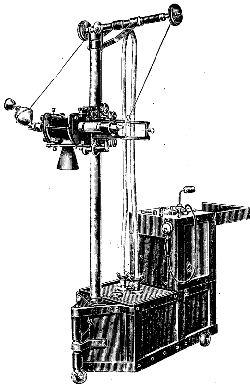
Рис. 13. Внешний вид аппарата без выпрямителя Моск. рентген. завода; 85 kV max до 30 mA.
