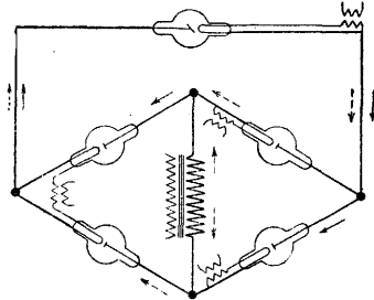
Рис. 18. Схема включения 4 кенотронов по правилу Греца.
