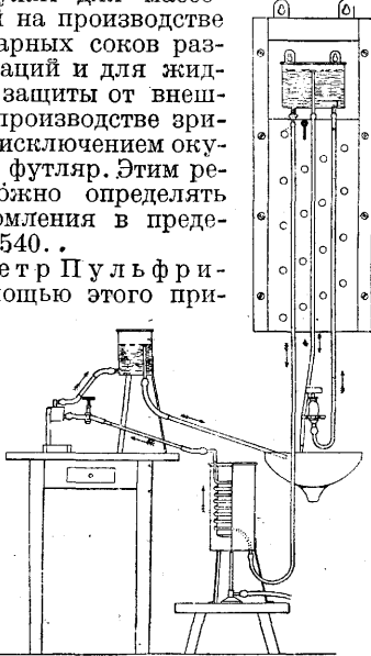
Рис. 5. Приспособление для нагревания рефрактометра.
