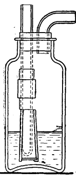
Рис. 3. Импинджер.
