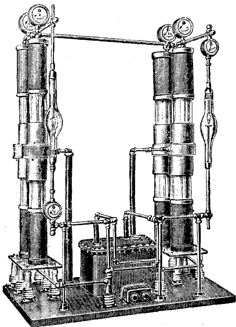
Рис. 24. Внешний вид аппарата Моск. рентген. зав. по системе Витка; до 220 kV max и 10 mA.
