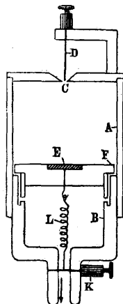
Рис. 4. Микроэлектрофильтр.
