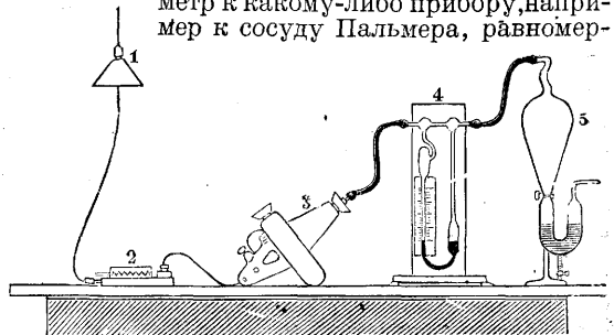
Рис. 2. Схема применения реометра: 1—электрическая арматура со штепселем для получения электрического тока; 2—реостат; 3—электрический насос-вентилятор; 4—реометр; 5—сосуд Пальмера для улавливания пыли.
