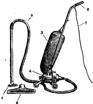
Рис. 2. Переносный пылесос «Вампир»: 1—гладкий наконечник; 2—гибкий металлический шланг; 3—вентилятор; 4—мотор; 5—собираетель пыли; 6—наконечник со щеткой; 7—шнур к штепселю; 8—рукоятка с выключателем.
