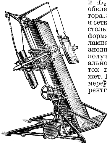
Рис. 37. Штатив для просвечивания заграничных фирм.
