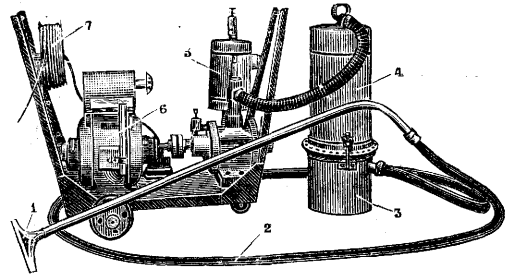
Рис. 3. Первозимый пылесос: 1—наконечник; 2—насосывающий шланг; 3—сосуд для собирания пыли; 4—резервуар с фильтрами; 5—засасывающий вентилятор; 6—мотор; 7—шнур к штепселю. Насасывательная нагрузка прибора равна 60 м 3 в час. Электромотор в одну лошадиную силу. Размеры прибора—90,0×43,5×70,0 см. Вес—95 кг без принадлежностей.
