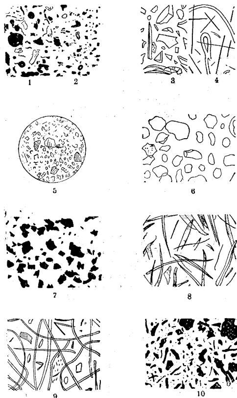
Рис. 2. Виды пыли по Wegmann'у: 1—пыль при точке игол; 2—пыль при чистое литье; 3—стекло; 4—шлаковая шерсть; 5—мрамор; 6—кварцевый песок; 7—бронза; 8—хвойное дерево; 9—пенька; 10—каменный уголь.
