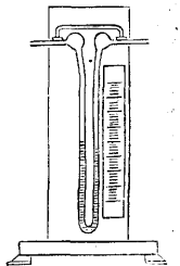
Рис. 3. Реометр с капилляром.
