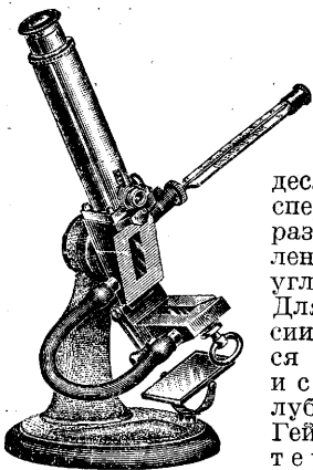
Рис. 6. Буттеррефрактометр Волни с открытой двойной призмой.
