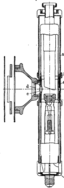
Рис. 8. Схема металлической рентгеновской трубки: а—бакелитовая муфта; б—медная оболочка; в—свинцовая; г—фильтр; д—окошечко для выхода лучей; е—окошечко для выхода лучей; ф—цилиндр из хромистого железа; г—просвинцованная резина.
