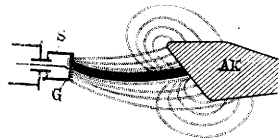
Рис. 6. Пути электронов в трубке: G —спираль катода; AK —антикатод; S —чашечка катода.
