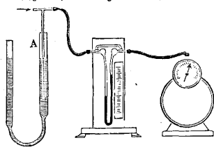
Рис. 4. Соединение реометра с газовыми часами.
