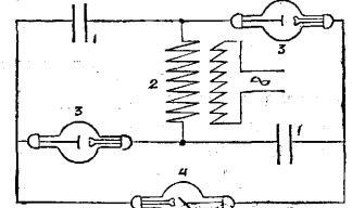
Рис. 22. Схема утраивания: 1—конденсатор; 2—трансформатор; 3—кеноотрон; 4—рентг. трубка.
