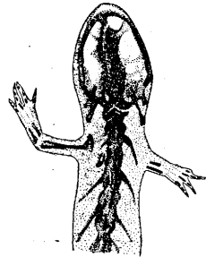
рис. 8. Рентгенограмма регенерации бескостной конечности у Triton cristatus. Удалены плечевой пояс и плечо; ампутация выше локтя. Регенерированы предплечье с костями предплечья и кисть с фалангами. Сargus еще хрящевой, radius и ulna сдвинуты в бескостное плечо. (По Коршельту.)
