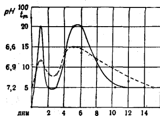
Рис. 3. Сплошная линия — изменение интенсивности митогенетического излучения регенерирующего хвоста аксолотля. На ординате условные единицы интенсивности излучения. Прерывистая линия — изменения активной реакции тканей регенерирующей конечности аксолотля. На ординате — значения pH (данные Окунева). На абсциссе — дни регенерации. (Из Бляхера и Бромлей.)
