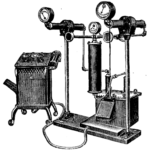
Рис. 17. Однокенотронный аппарат, нагрузка—до 150 mA и 100 kV max .
