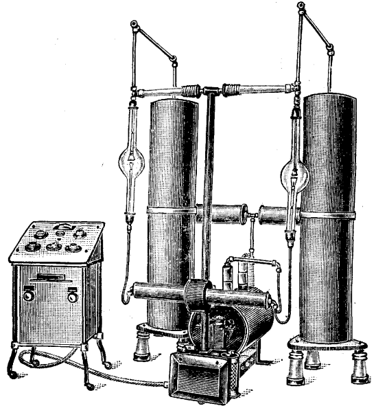
Рис. 21. Внешний вид конденсаторной установки.
