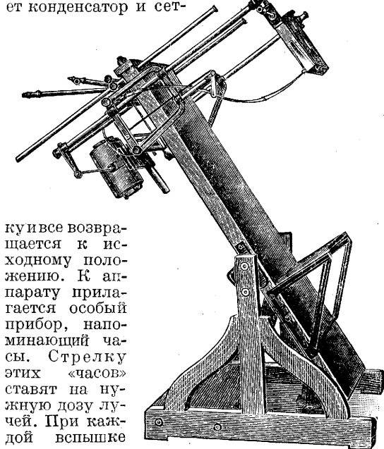
Рис. 38. Штатив для просвечиваний Моск. рентген. завода.
