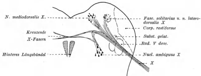
Abb. 63. Vagusursprung. (Schema.)
