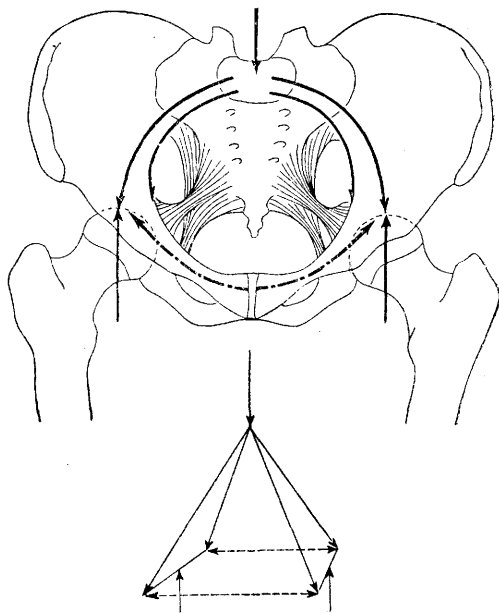
Рис. 25. Схема статики человеческого таза. Вертикальные стрелки—нагрузка крестца от туловища и опорные реакции тазобедренных сочленений. Кривые стрелки: сплошные—линии усилий сжатия, пунктирные—линии усилий растяжения. Внизу приведена схема тех усилий в виде палатки.
