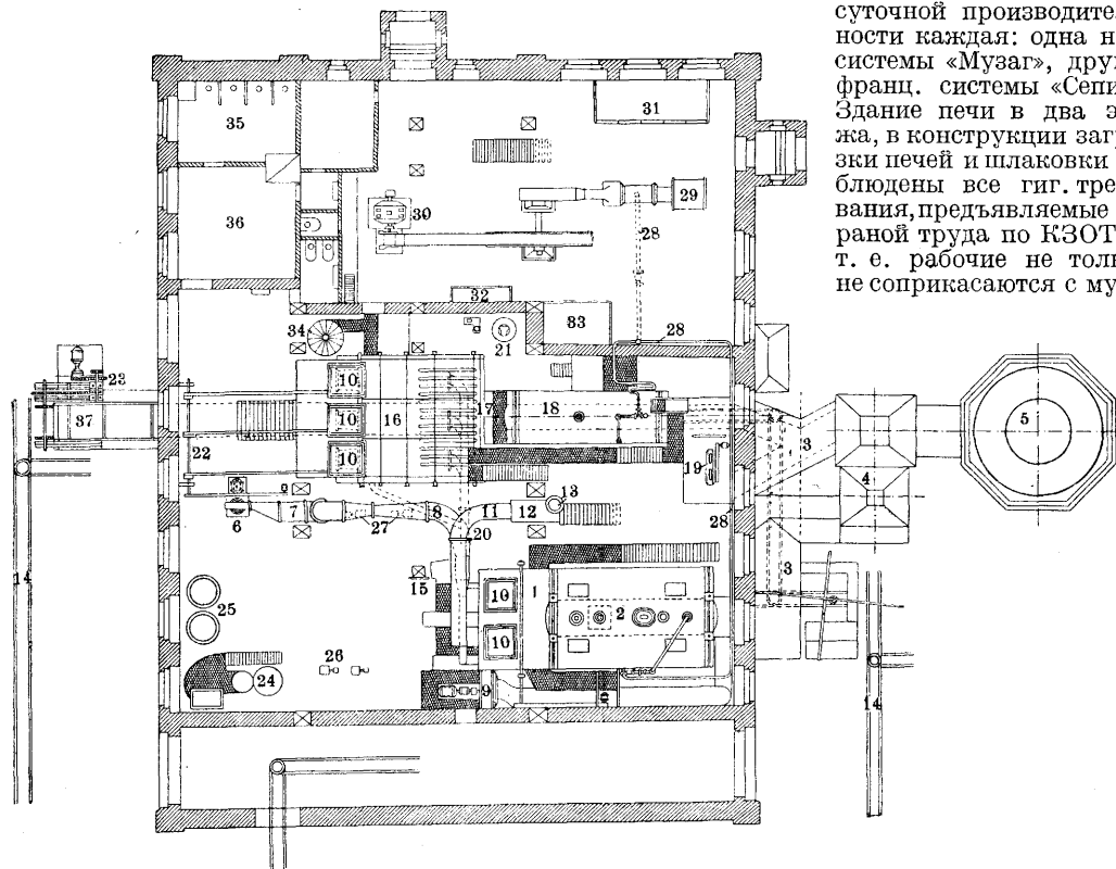
Рис. 2. План мусоросжигательной станции в Москве: 1—печь системы «Музаг»; 2—котел системы «Гумбольдт»; 3—боров к дымовой трубе; 4 и 12—теплоуловитель; 5—дымовая труба; 6—вентилятор для печи; 7—паровой подогреватель воздуха; 8—воздухопровод в печь; 9—эксгаустерное устройство; 10—сушильный аппарат; 11—трубопровод от сушильного аппарата; 13—труба для отвода паров подсушиваемого мусора; 14—вагонетные пути; 15—измерительные приборы; 16—печь системы «Сепиа»; 17—боров, соединяющий печь с котлом; 18—котел системы «Бабкок и Вилькокс»; 19—экономайзер Грина; 20—вентилятор для печи «Сепиа»; 21—гидравлический аккумулятор; 22—трансмиссия для загрузочного устройства; 23—трансмиссия для транспорта шлама; 24—водоочиститель системы «Зейферт»; 25—бани питательной воды; 26—насосы для котла «Гумбольдт»; 27—насосы для котла «Бабкок и Вилькокс»; 28—трубопровод и паровой машине; 29—паровая машина; 30—генератор; 31—главный распределительный щит; 32—осветительный щит; 33—регистрирующие измерительные приборы; 34—винтовая лестница; 35—душ; 36—раздевальня; 37—транспортёр для подъема шлама.
